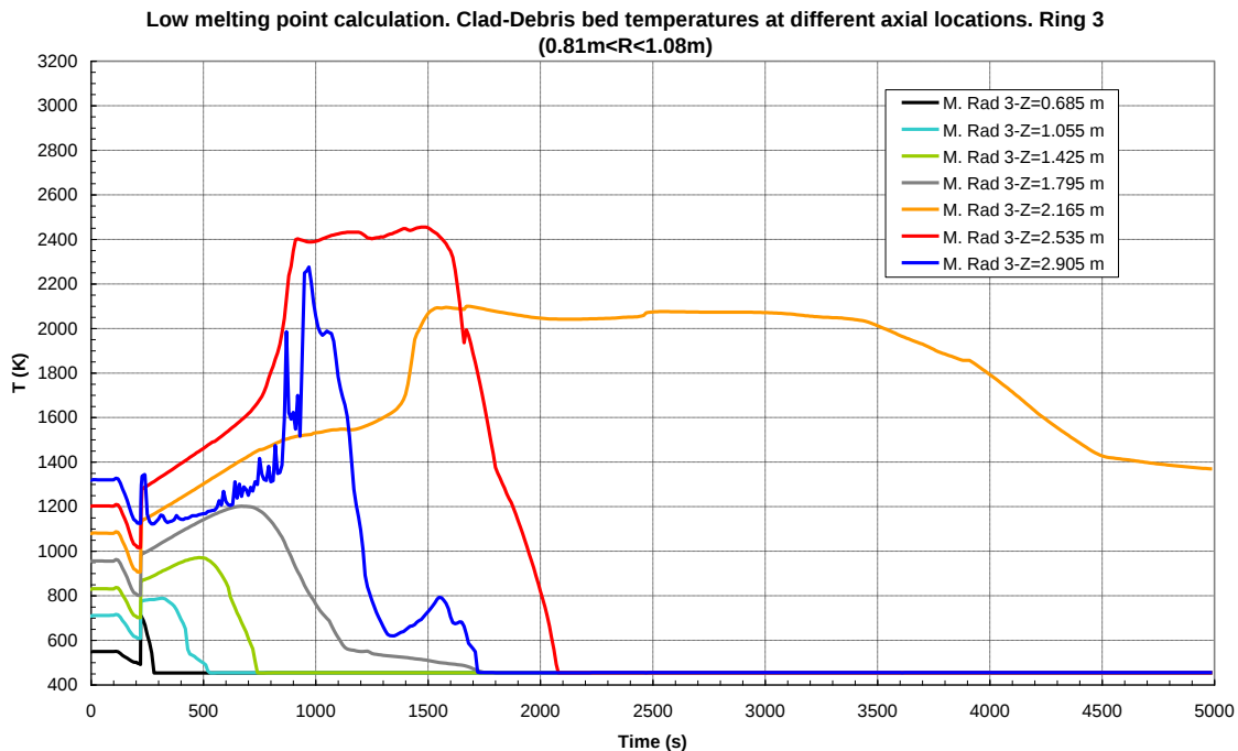
Figura 42: Calcolo con bassa temperatura di fusione (UO 2 e ZrO 2 ). Temperature del combustibile a diverse quote nella regione fra 0.81 m e 1.08 m (maglia radiale 3)
