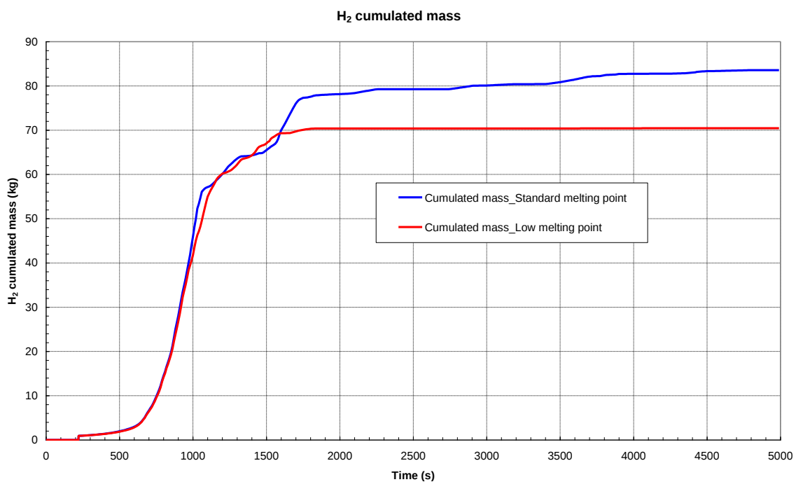
Figura 47: Calcolo di sensibilità alla temperatura di fusione. Idrogeno prodotto durante il transitorio
