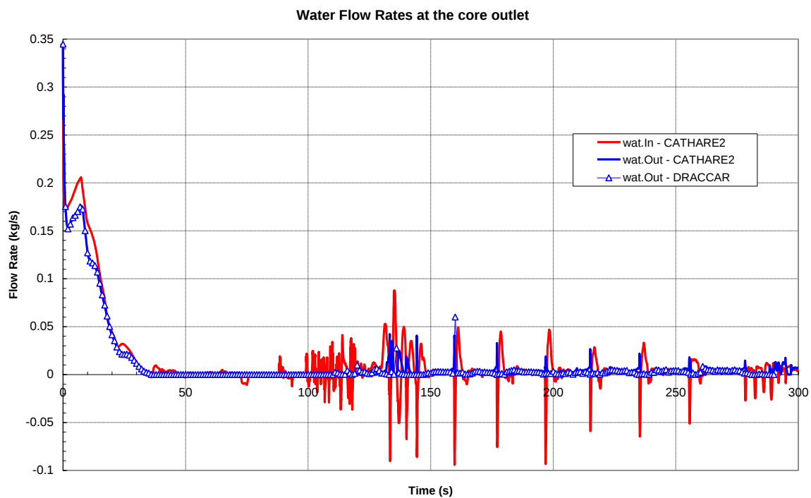
Figura 56: Portata di acqua in funzione del tempo all'uscita del sottocanale fluido
