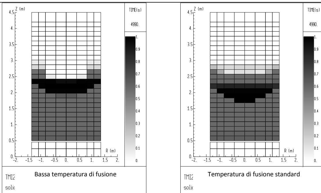
Figura 39: Calcolo di sensibilità alla temperatura di fusione. Frazione volumica di corium a 5000 s
