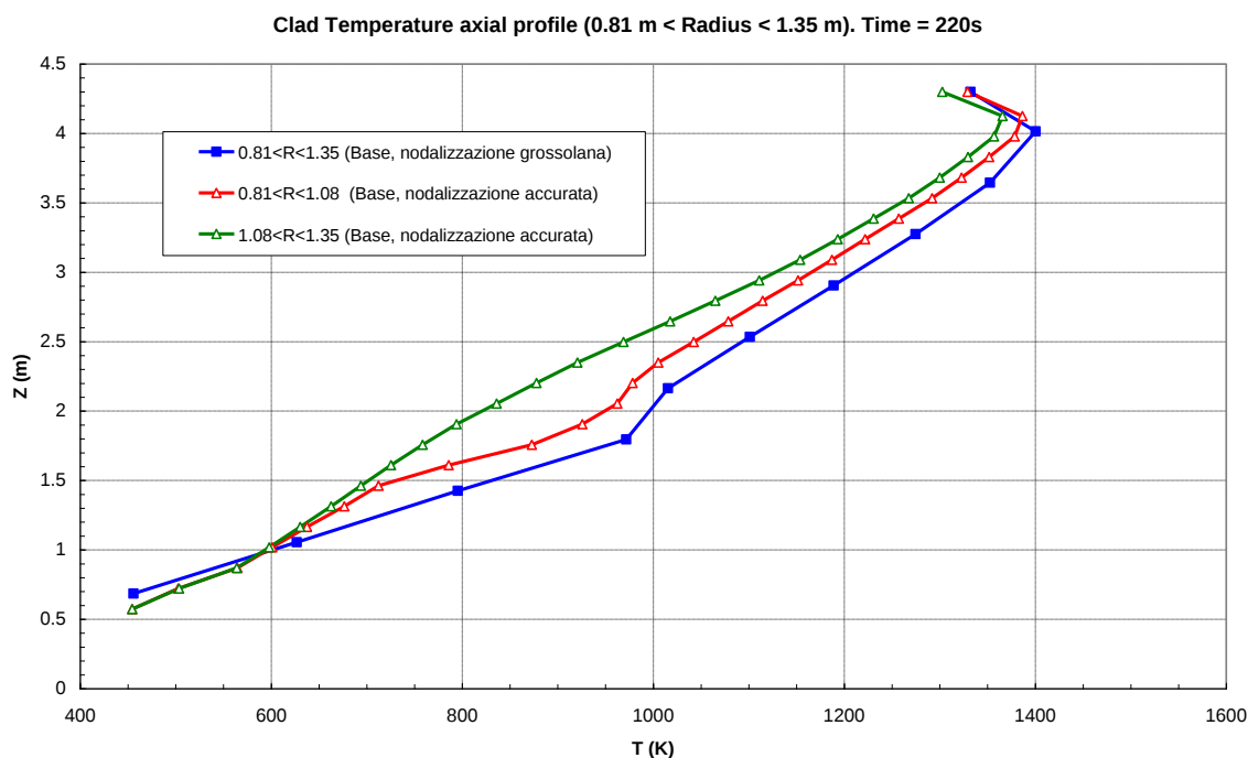
Figura 5: Calcolo Base. Profilo assiale delle temperature di guaina, nella regione fra 0.81 m e 1.35 m, a 220 s (prima della formazione del debris bed)
