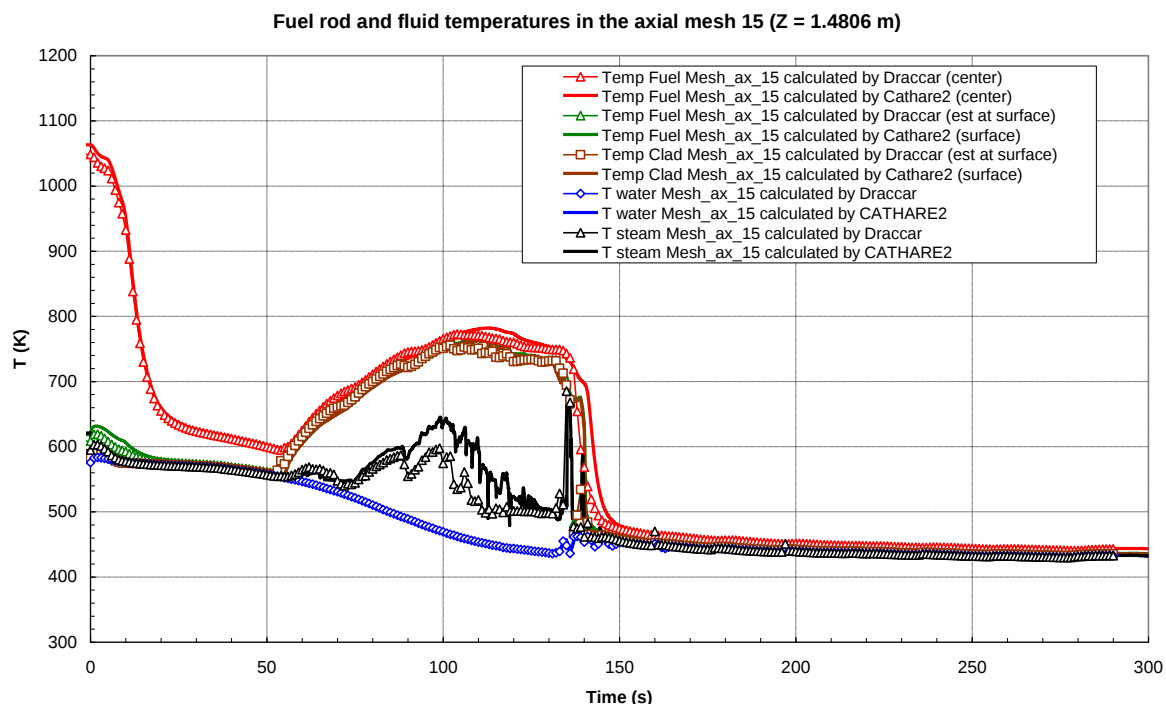
Figura 64: Temperature durante il transitorio alla quota di 1.4806 m (maglia assiale 15)
