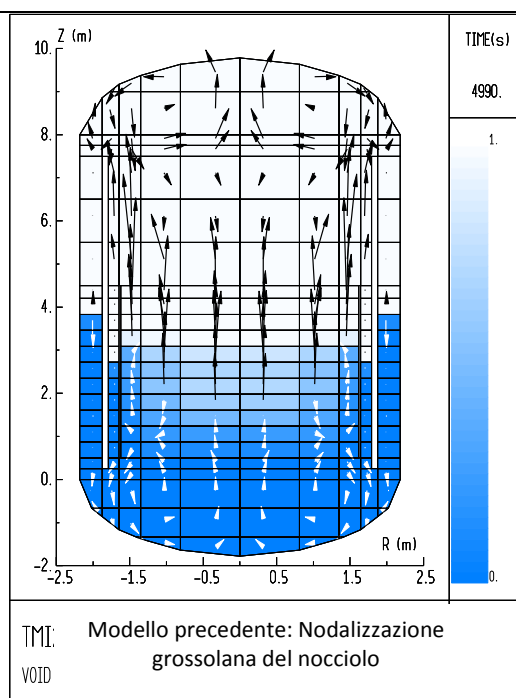
Figura 18: Calcolo base. Frazione di vuoto e velocità del fluido (acqua - vapore) a 5000 s
