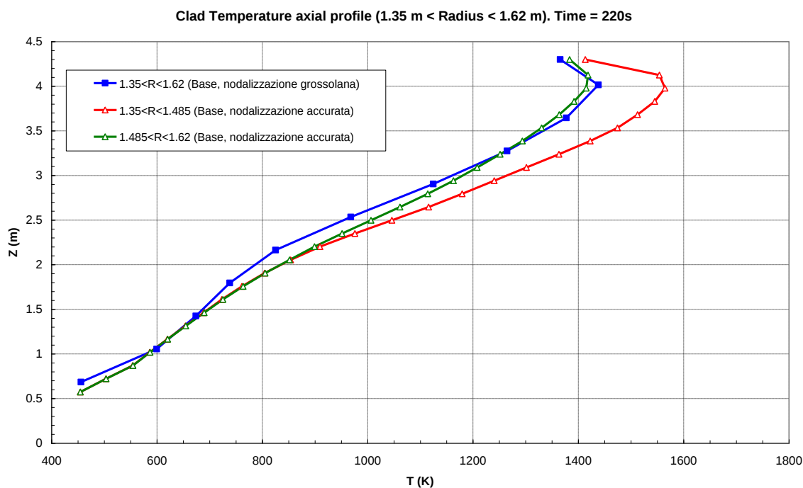
Figura 6: Calcolo Base. Profilo assiale delle temperature di guaina, nella regione fra 1.35 m e 1.62 m, a 220 s (prima della formazione del debris bed)
