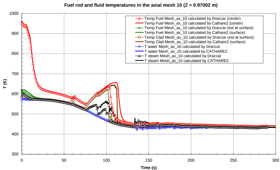
Figura 62: Temperature durante il transitorio alla quota di 0.97002 m (maglia assiale 10)
