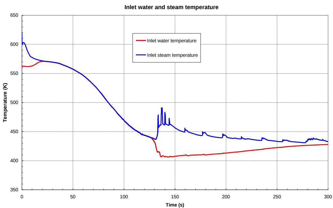
Figura 53: Condizioni al contorno - Temperatura acqua e vapore all'ingresso dell'estremità inferiore del sottocanale fluido
