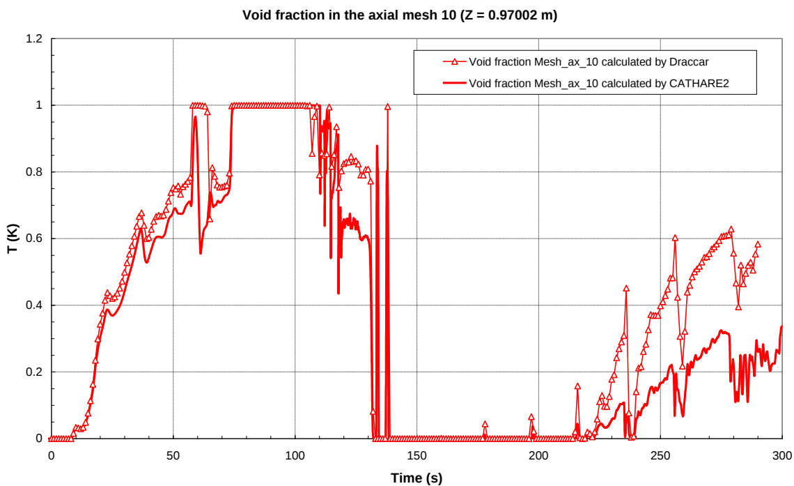
Figura 63: Frazione di vuoto durante il transitorio alla quota di 0.97002 m (maglia assiale 10)
