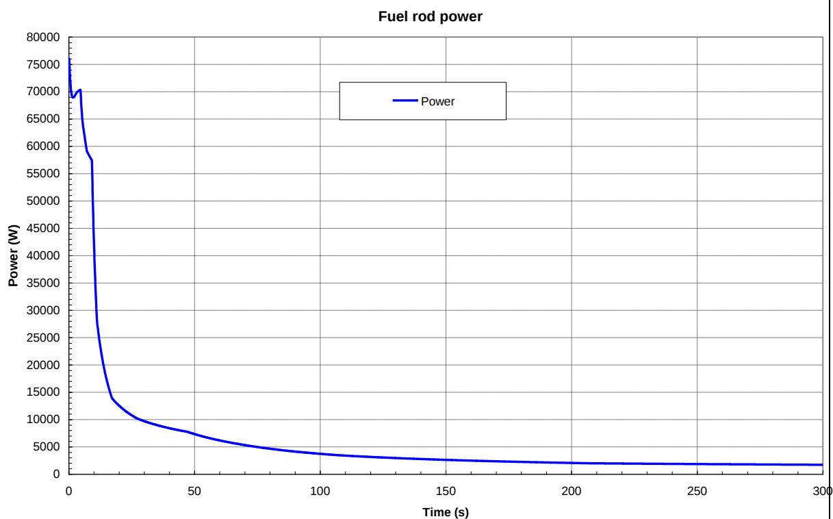
Figura 50: Condizioni al contorno - Potenza della singola barretta di combustibile
