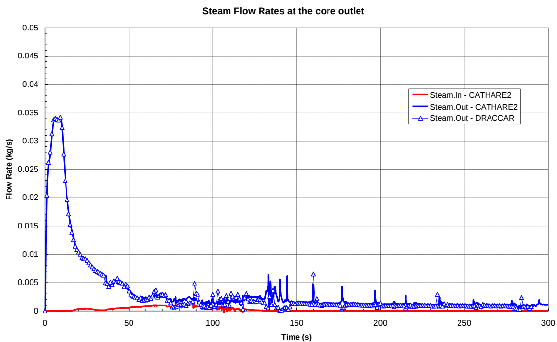
Figura 57: Portata di vapore in funzione del tempo all'uscita del sottocanale fluido
