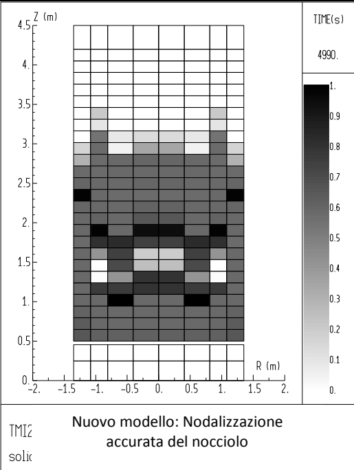
Figura 17: Calcolo base. Frazione volumica di corium (liquido + solido) a 5000 s
