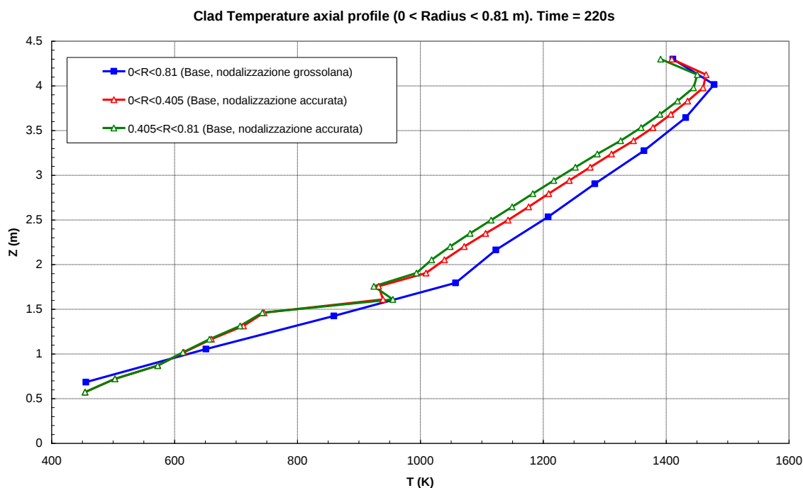
Figura 4: Calcolo Base. Profilo assiale delle temperature di guaina, nella regione fra 0 e 0.81 m, a 220 s (prima della formazione del debris bed)
