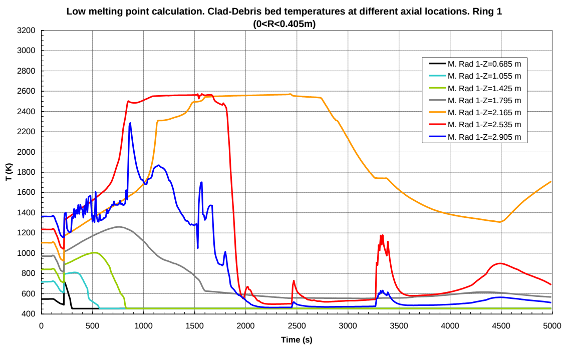
Figura 40: Calcolo con bassa temperatura di fusione (UO 2 e ZrO 2 ). Temperature del combustibile a diverse quote nella regione fra 0 e 0.405 m (maglia radiale 1)
