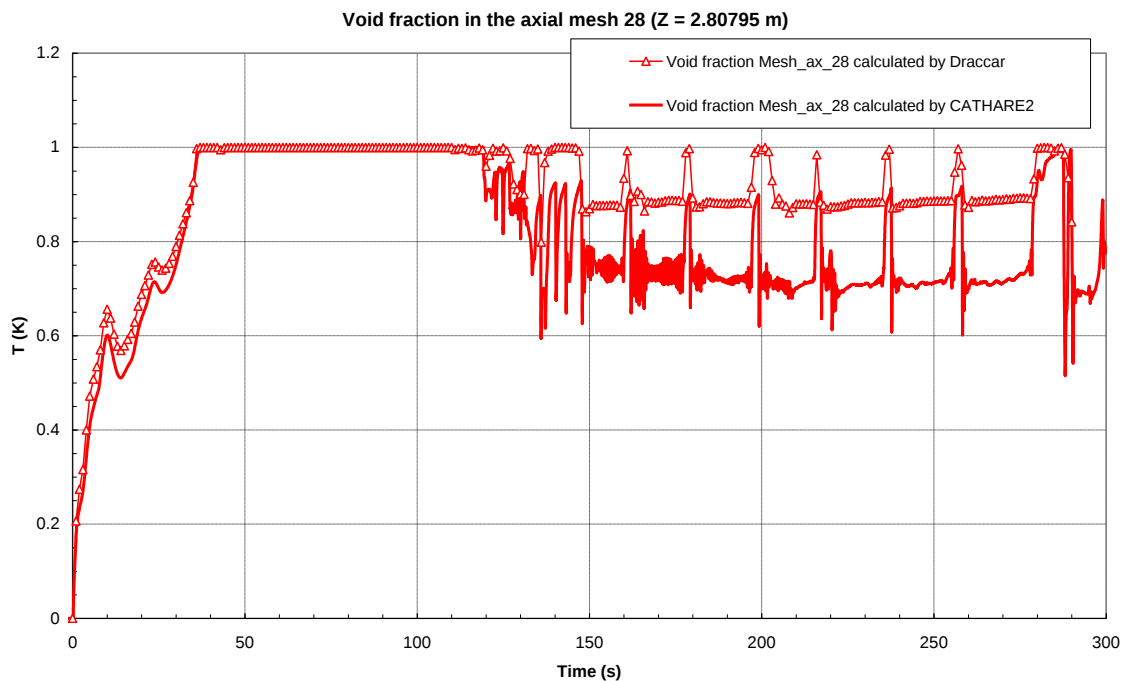
Figura 69: Frazione di vuoto durante il transitorio alla quota di 2.80795 m (maglia assiale 28)
