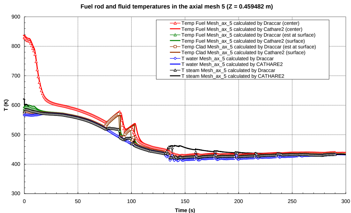
Figura 60: Temperature durante il transitorio alla quota di 0.459482 m (maglia assiale 5)
