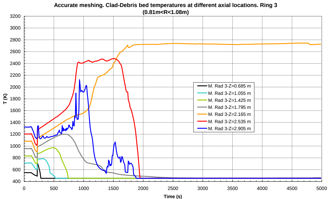
Figura 24: Calcolo senza le barre di controllo (nodalizzazione accurata). Temperature del combustibile a diverse quote nella regione fra 0.81 m e 1.08 m (maglia radiale 3)
