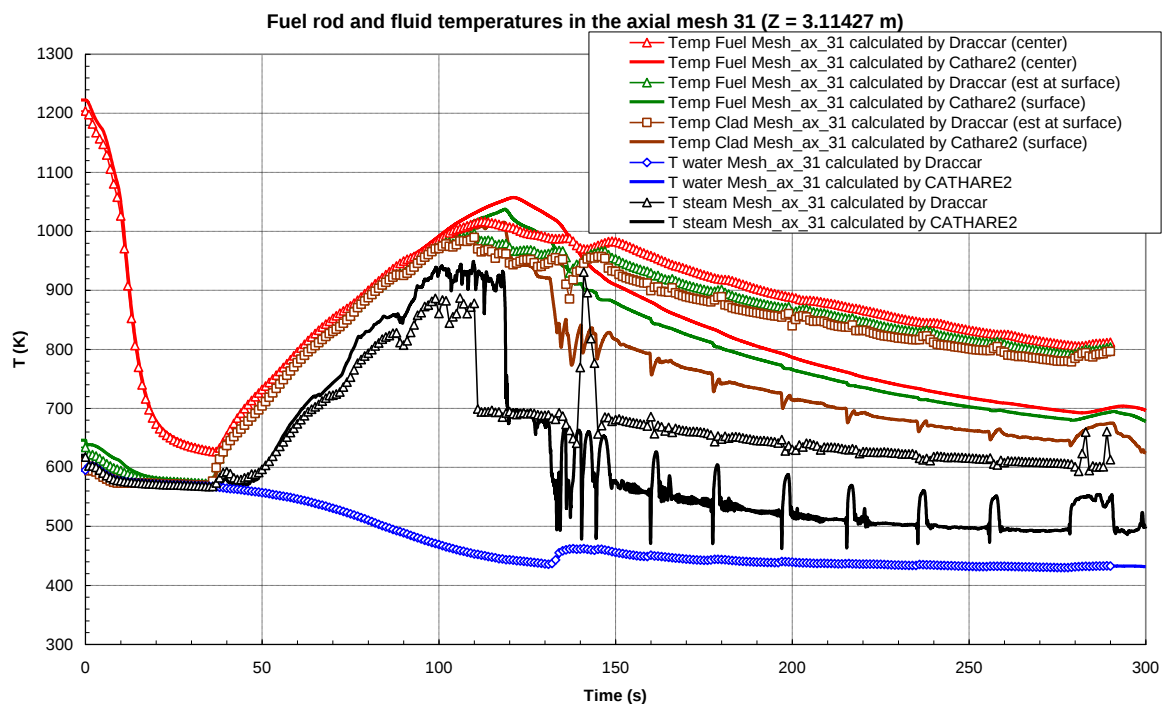
Figura 70: Temperature durante il transitorio alla quota di 3.11427 m (maglia assiale 31)
