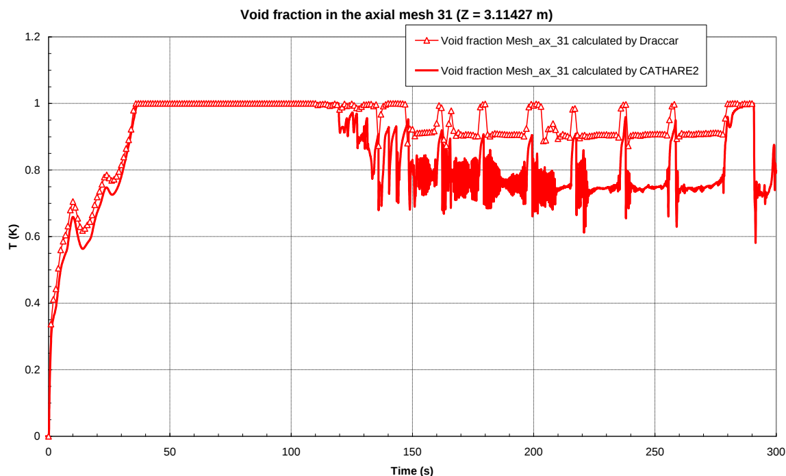
Figura 71: Frazione di vuoto durante il transitorio alla quota di 3.11427 m (maglia assiale 31)
