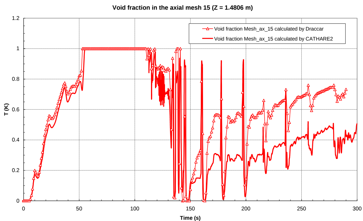
Figura 65: Frazione di vuoto durante il transitorio alla quota di 1.4806 m (maglia assiale 15)
