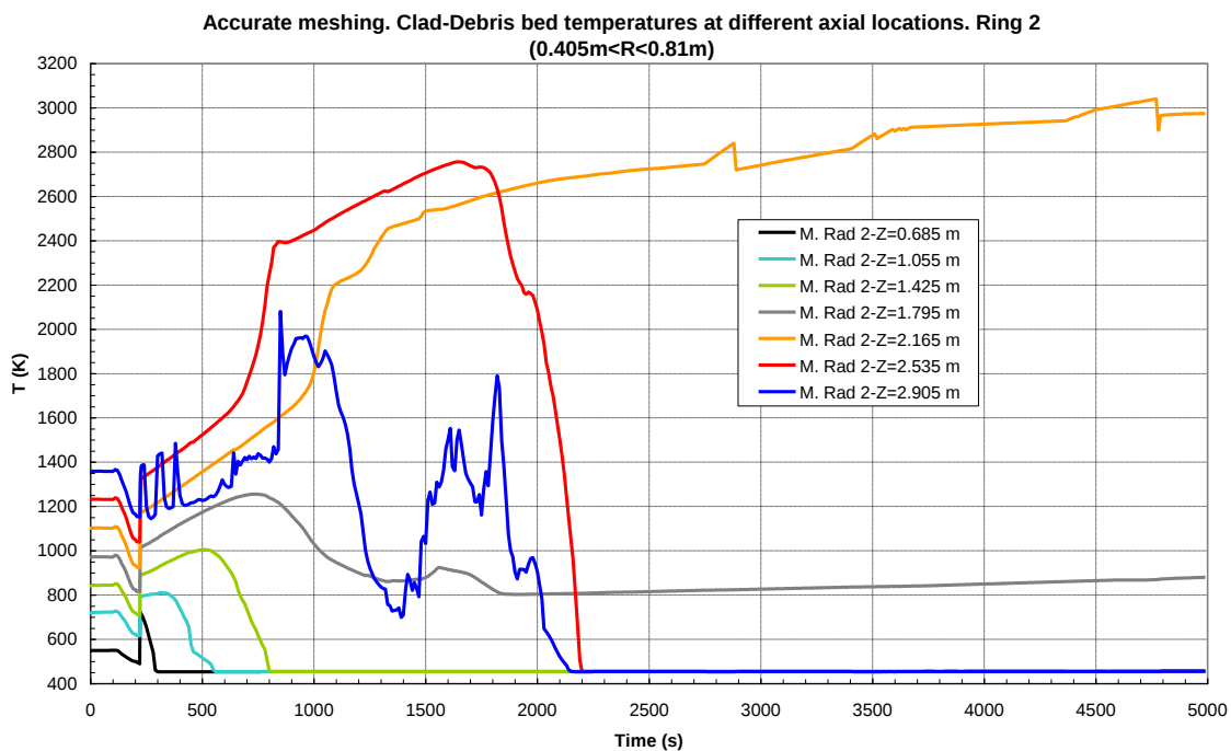
Figura 23: Calcolo senza le barre di controllo (nodalizzazione accurata). Temperature del combustibile a diverse quote nella regione fra 0.405 m e 0.81 m (maglia radiale 2)
