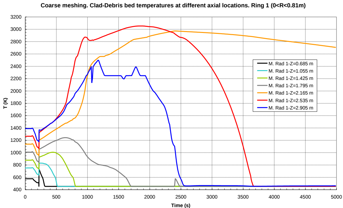
Figura 28: Calcolo senza le barre di controllo (nodalizzazione grossolana). Temperature del combustibile a diverse quote nella regione fra 0 e 0.81 m (maglia radiale 1)
