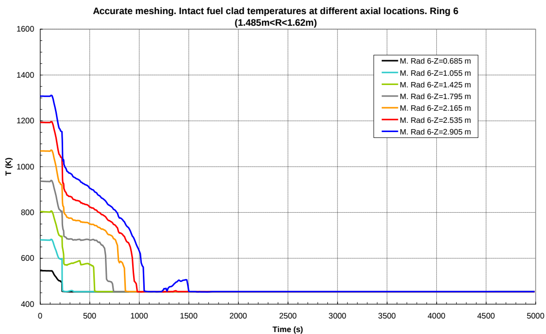
Figura 27: Calcolo senza le barre di controllo (nodalizzazione accurata). Temperature del combustibile (intatto) a diverse quote nella regione fra 1.485 m e 1.62 m (maglia radiale 6)
