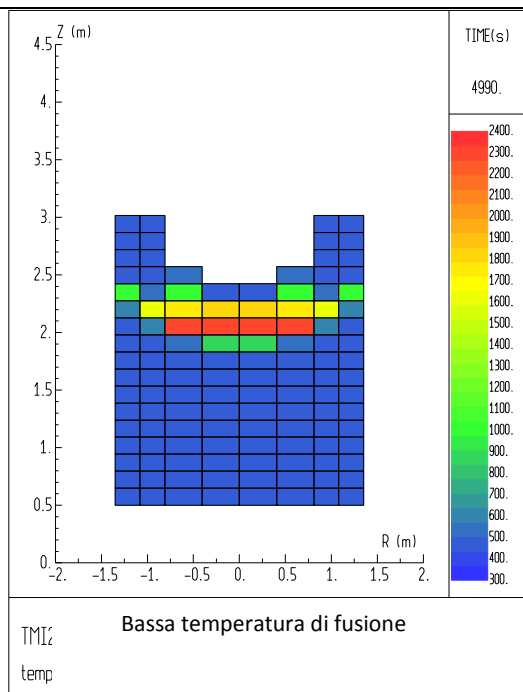
Figura 46: Calcolo di sensibilità alla temperatura di fusione. Campo di temperature nel corium a 5000 s
