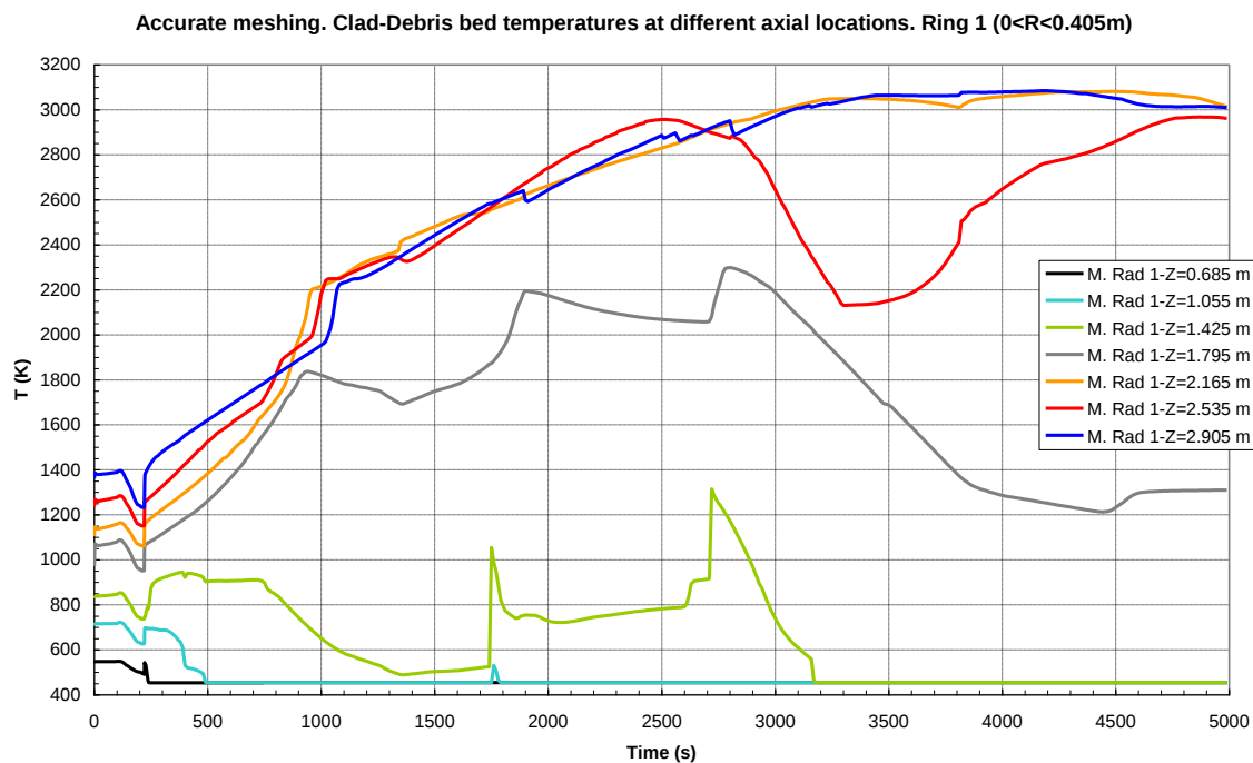
Figura 8: Calcolo base (nodalizzazione accurata). Temperature del combustibile a diverse quote nella regione fra 0 e 0.405 m (maglia radiale 1)
