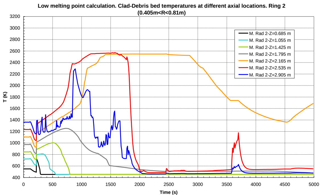
Figura 41: Calcolo con bassa temperatura di fusione (UO 2 e ZrO 2 ). Temperature del combustibile a diverse quote nella regione fra 0.405 m e 0.81 m (maglia radiale 2)
