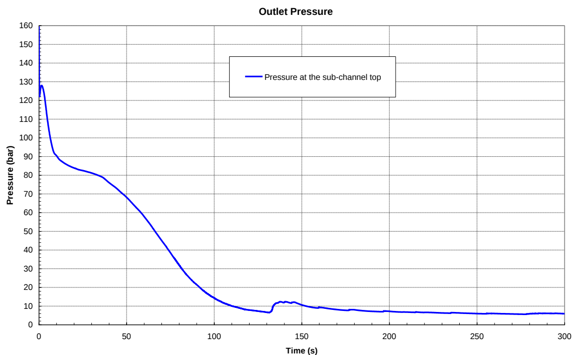
Figura 54: Condizioni al contorno - Pressione all'estremità superiore del sottocanale fluido
