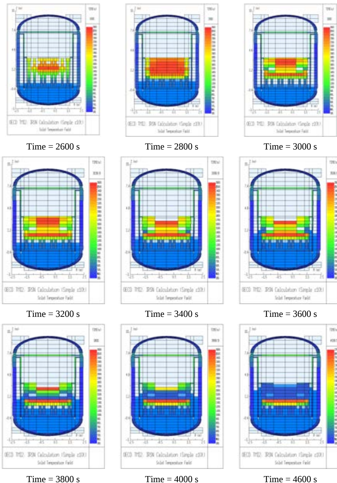
Figura 88: Progressione della degradazione del core durante la fase di reflooding
