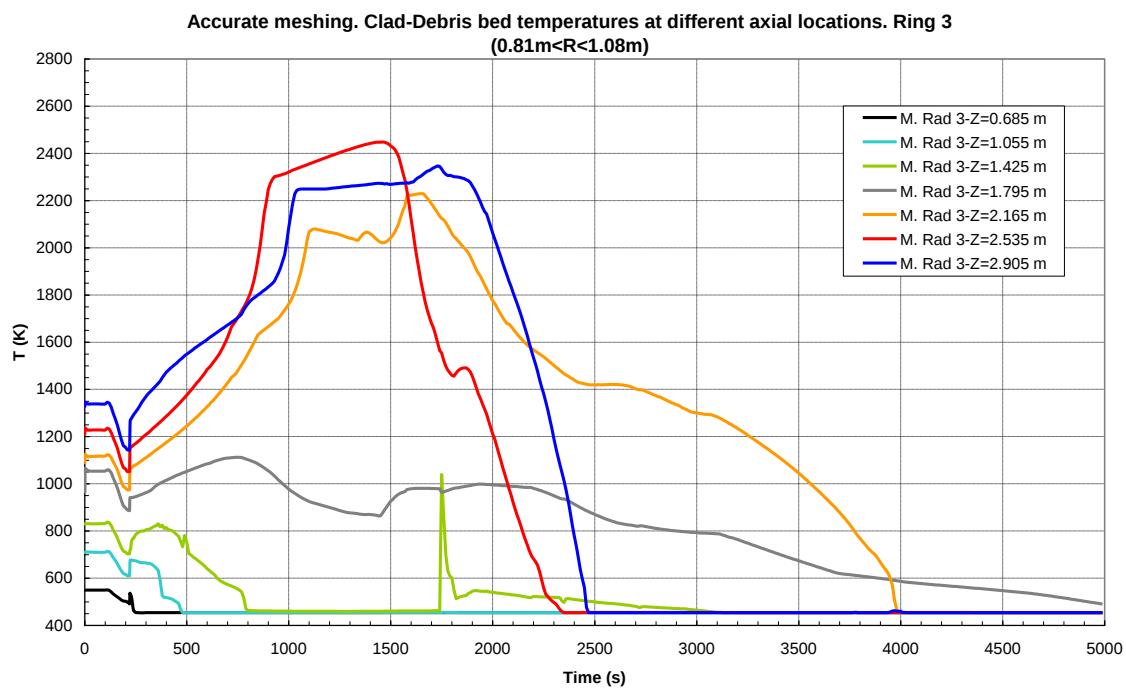
Figura 10: Calcolo base (nodalizzazione accurata). Temperature del combustibile a diverse quote nella regione fra 0.81 m e 1.08 m (maglia radiale 3)
