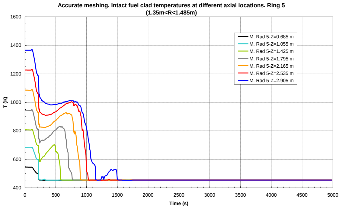
Figura 26: Calcolo senza le barre di controllo (nodalizzazione accurata). Temperature del combustibile (intatto) a diverse quote nella regione fra 1.35 m e 1.485 m (maglia radiale 5)
