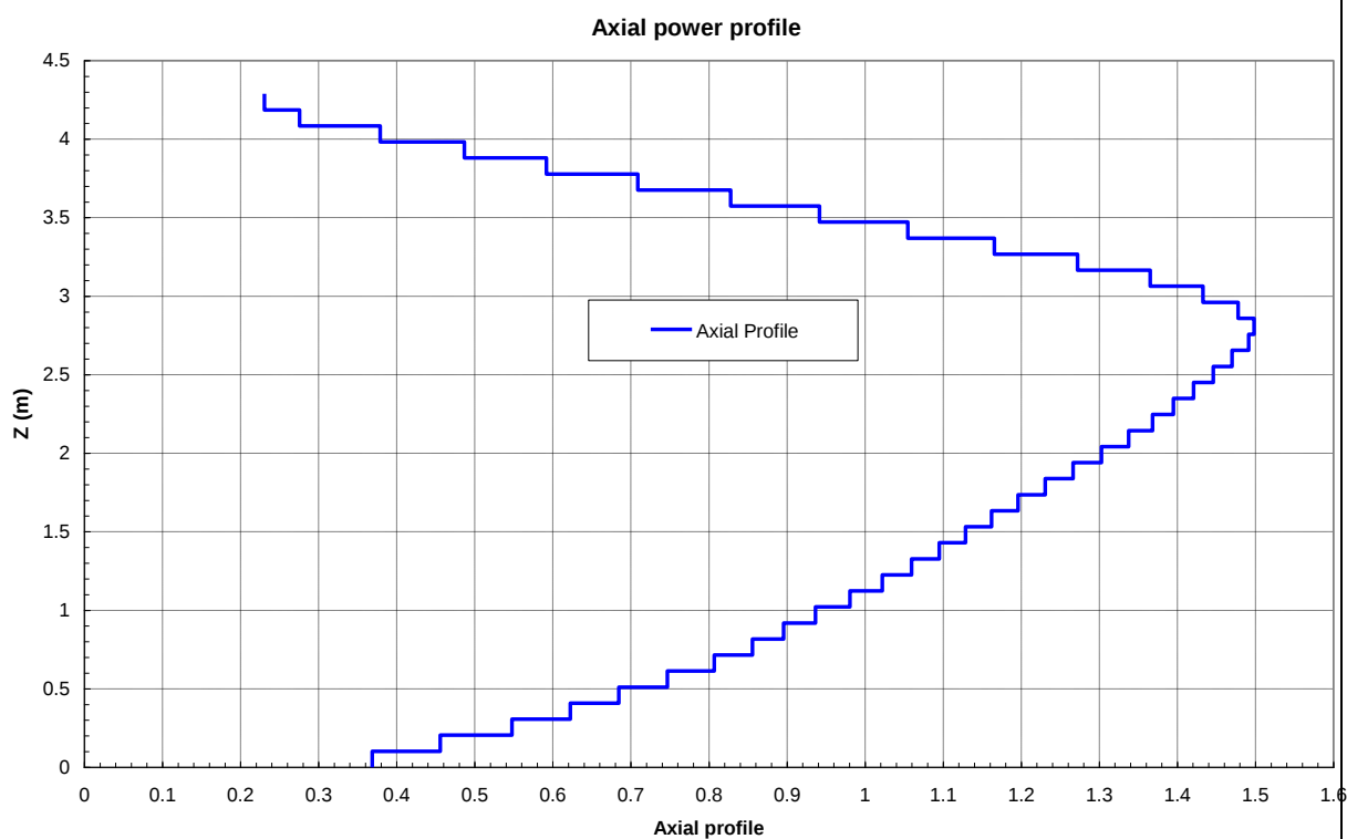
Figura 51: Condizioni al contorno - Profilo assiale di potenza
