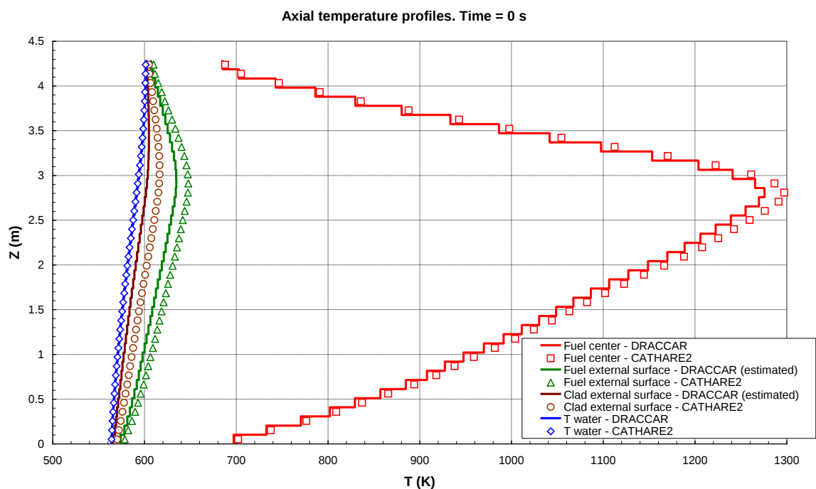
Figura 55: Profilo assiale delle temperature (barretta di combustibile ed acqua) all'inizio del transitorio incidentale (istante = 0 s)
