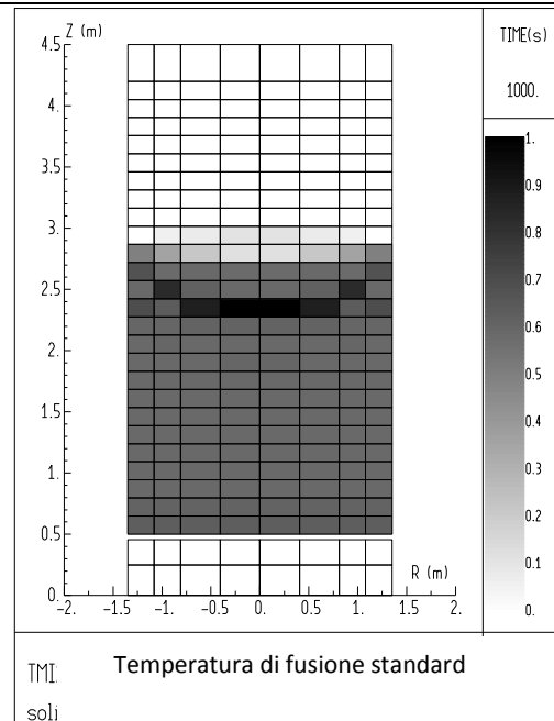
Figura 36: Calcolo di sensibilità alla temperatura di fusione. Frazione volumica di corium a 1000 s
