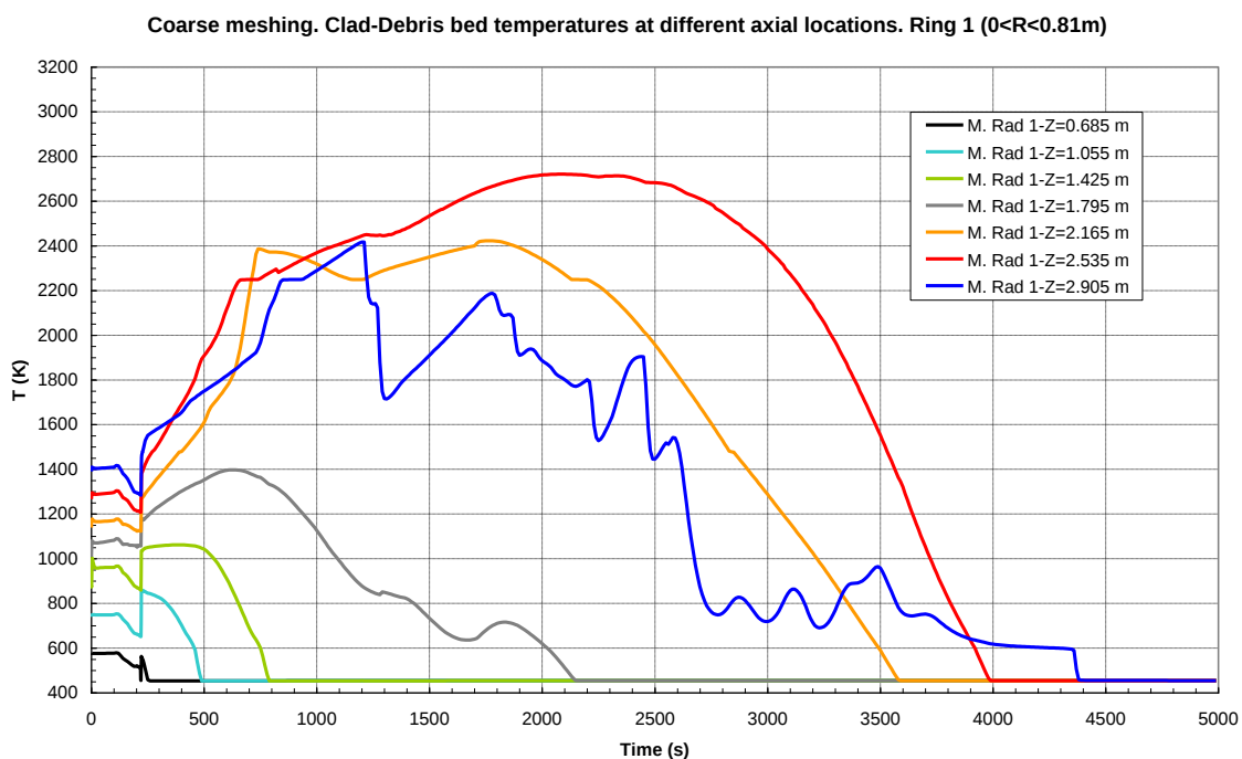
Figura 14: Calcolo base (nodalizzazione grossolana). Temperature del combustibile a diverse quote nella regione fra 0 e 0.81 m (maglia radiale 1)
