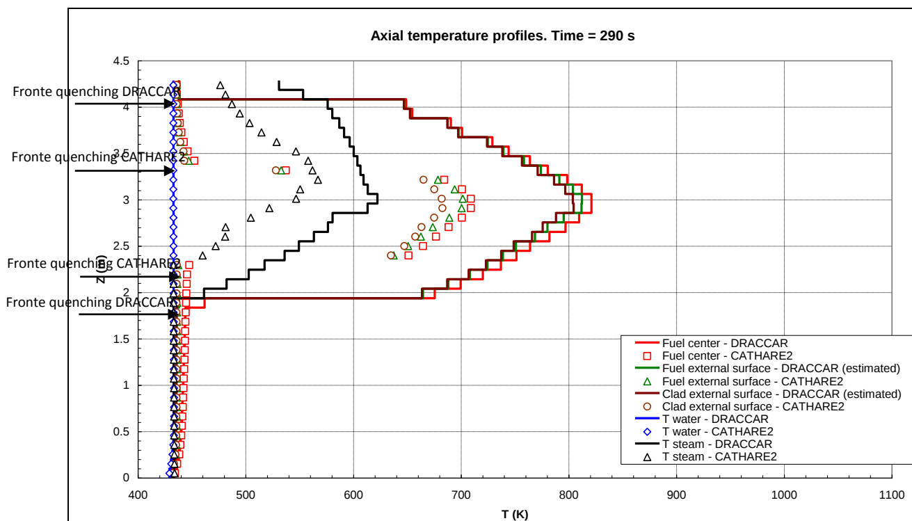
Figura 76: Profilo assiale delle temperature (combustibile e fluido) a 290 s (fine del transitorio calcolato)
