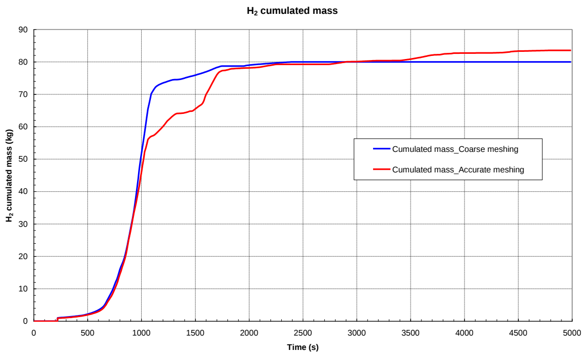
Figura 35: Calcolo senza le barre di controllo. Idrogeno prodotto durante il transitorio
