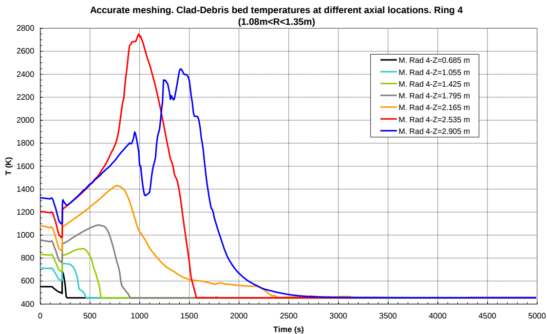
Figura 11: Calcolo base (nodalizzazione accurata). Temperature del combustibile a diverse quote nella regione fra 1.08 m e 1.35 m (maglia radiale 4)
