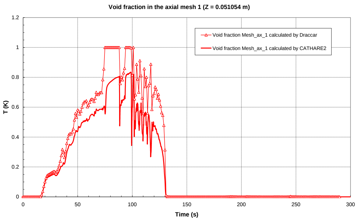
Figura 59: Frazione di vuoto durante il transitorio alla quota di 0.051054 m (maglia assiale 1)
