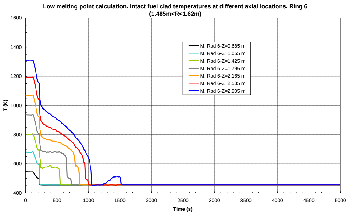
Figura 45: Calcolo con bassa temperatura di fusione (UO 2 e ZrO 2 ). Temperature del combustibile (intatto) a diverse quote nella regione fra 1.485 m e 1.62 m (maglia radiale 6)
