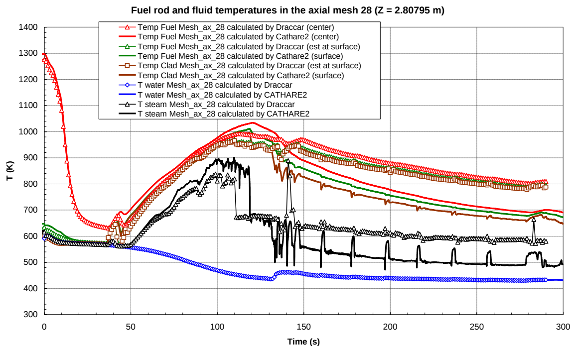
Figura 68: Temperature durante il transitorio alla quota di 2.80795 m (maglia assiale 28)
