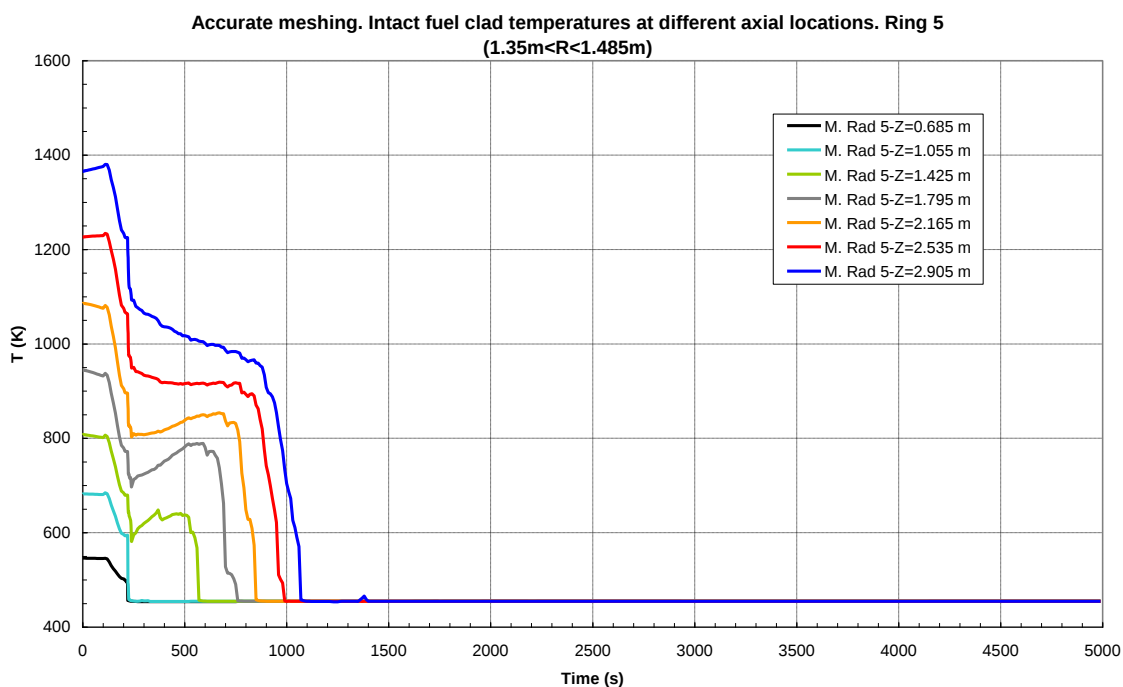
Figura 12: Calcolo base (nodalizzazione accurata). Temperature del combustibile (intatto) a diverse quote nella regione fra 1.35 m e 1.485 m (maglia radiale 5)
