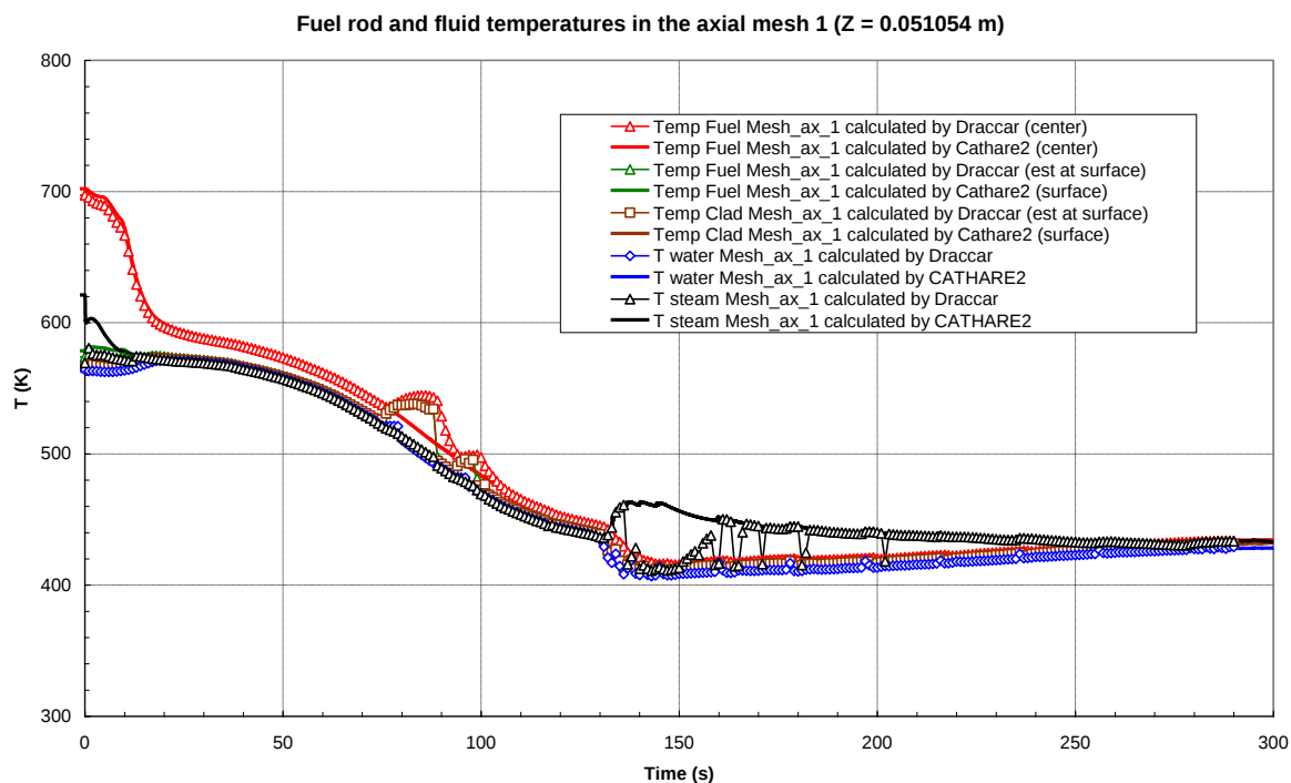
Figura 58: Temperature durante il transitorio alla quota di 0.051054 m (maglia assiale 1)
