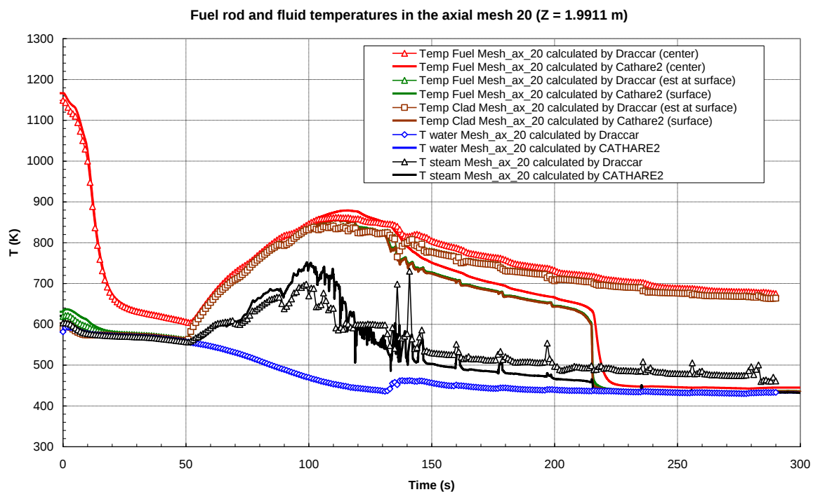
Figura 66: Temperature durante il transitorio alla quota di 1.9911 m (maglia assiale 20)
