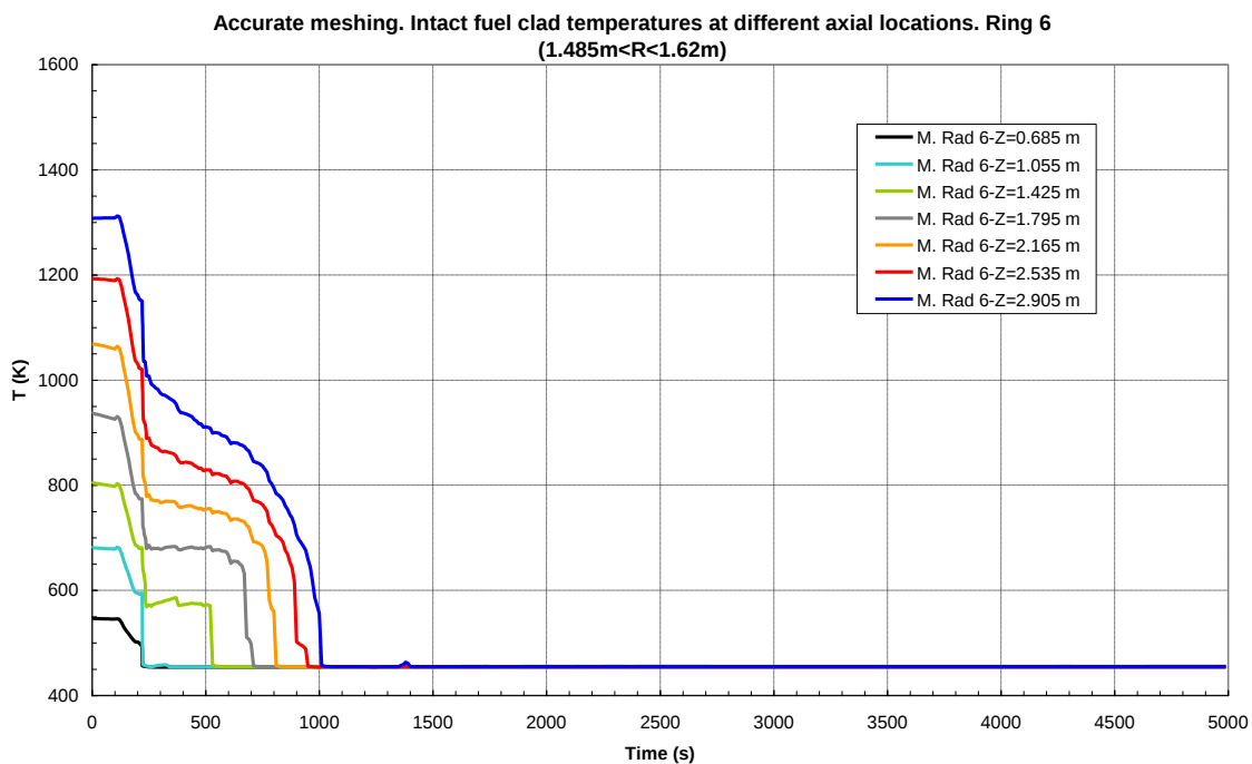
Figura 13: Calcolo base (nodalizzazione accurata). Temperature del combustibile (intatto) a diverse quote nella regione fra 1.485 m e 1.62 m (maglia radiale 6)
