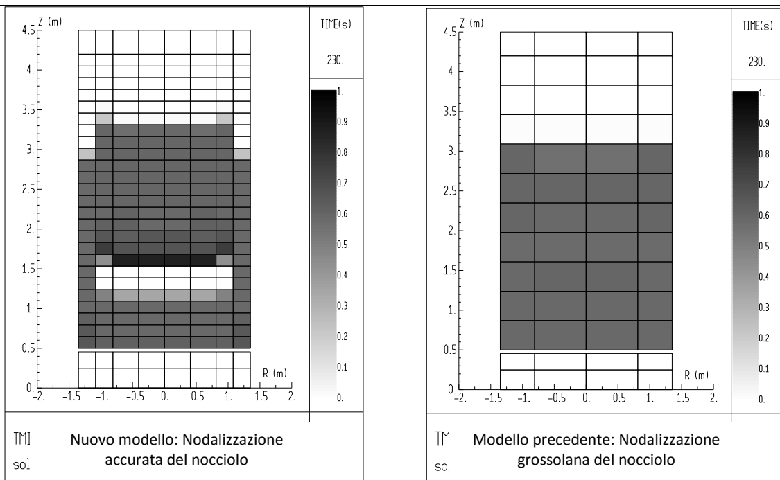
Figura 7: Calcolo base. Frazione volumica di corium (liquido+solido) a 230 s (subito dopo la formazione ed il collasso del debris bed)
