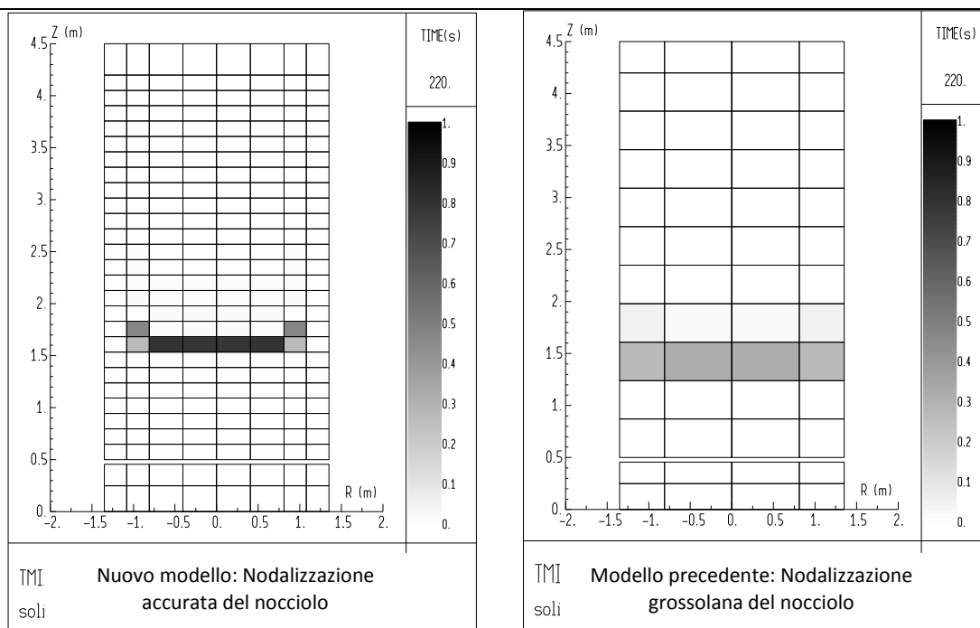
Figura 3: Calcolo base. Frazione volumica di corium (liquido+solido) a 220 s (prima della formazione del debris bed)
