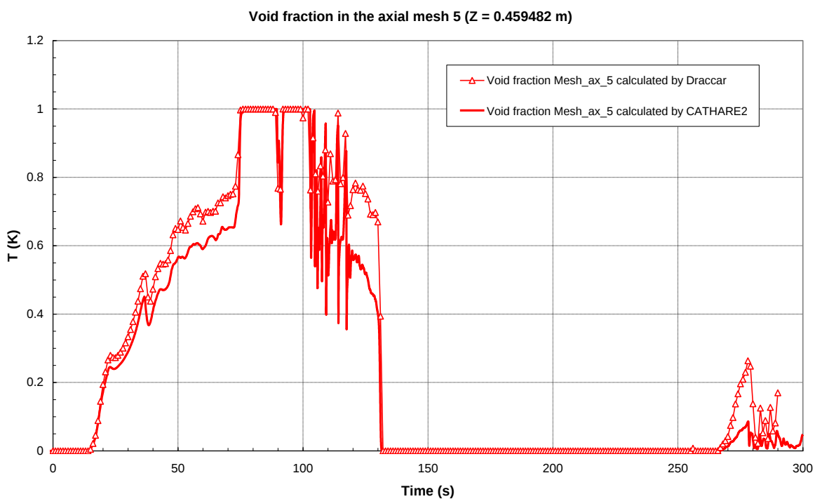
Figura 61: Frazione di vuoto durante il transitorio alla quota di 0.459482 m (maglia assiale 5)
