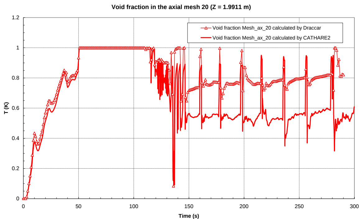
Figura 67: Frazione di vuoto durante il transitorio alla quota di 1.9911 m (maglia assiale 20)
