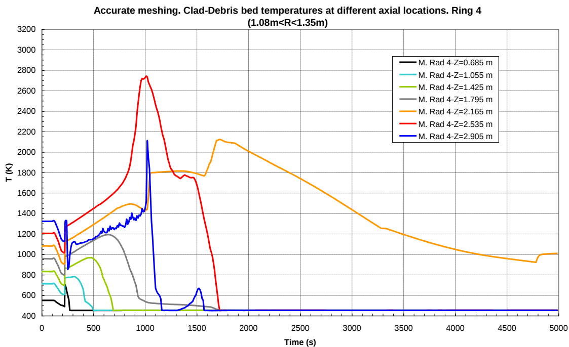
Figura 25: Calcolo senza le barre di controllo (nodalizzazione accurata). Temperature del combustibile a diverse quote nella regione fra 1.08 m e 1.35 m (maglia radiale 4)
