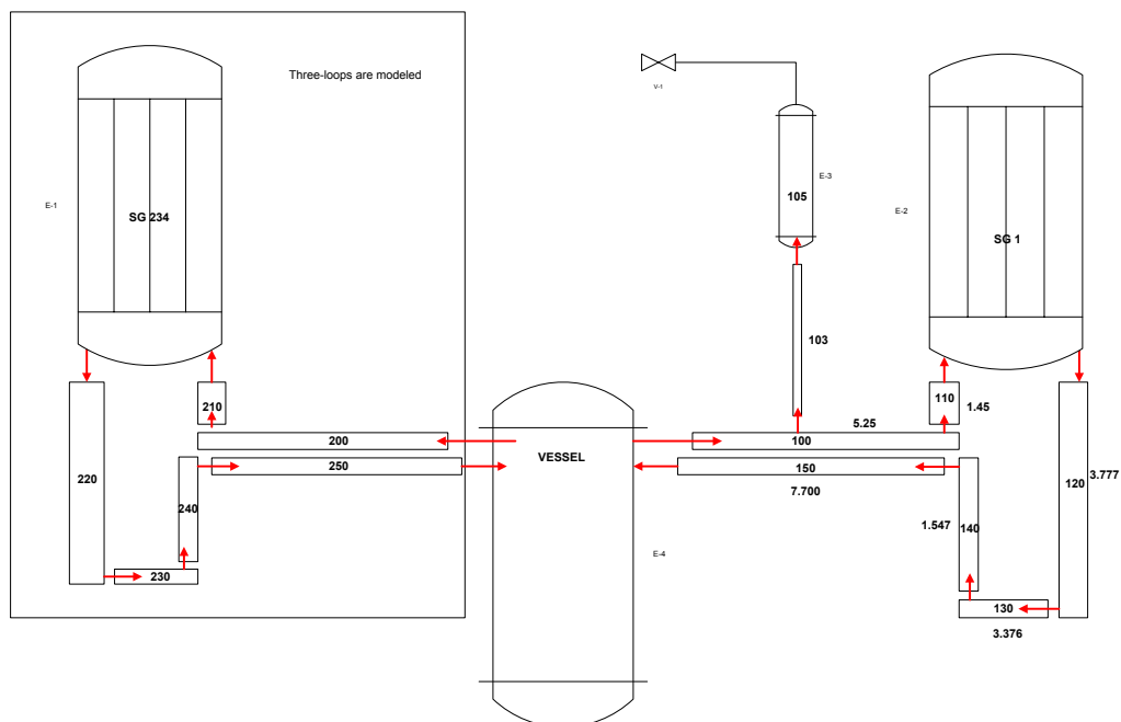
Figura 10.nodalizzazione del sistema primario del Mille600 per MELCOR
