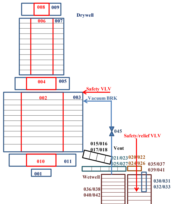
Figura 6. – Nodalizzazione contenimento
