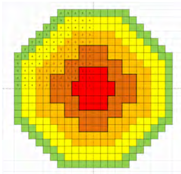
Figura 7.– Nodalizzazione Core
