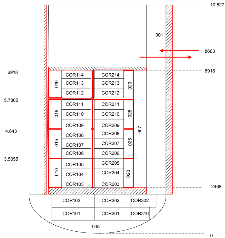
Figura 9. nodalizzazione del core del Mille600 per MELCOR
