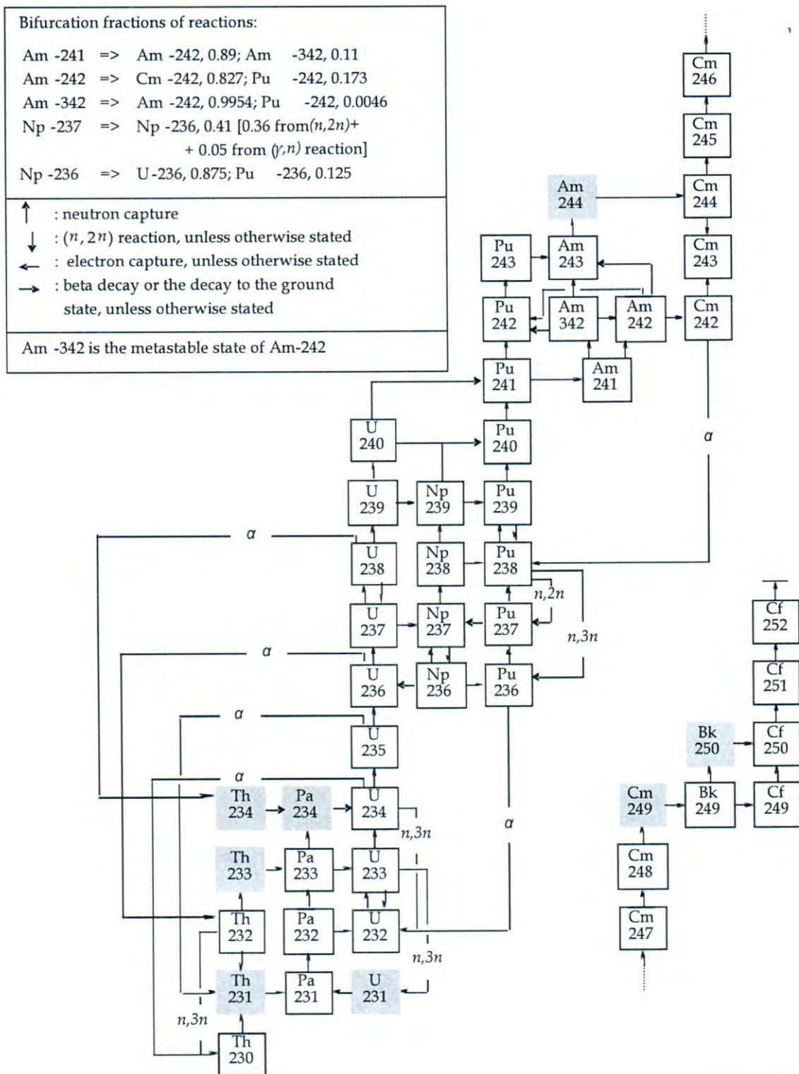
Figura 30. Heavy-metal chains
