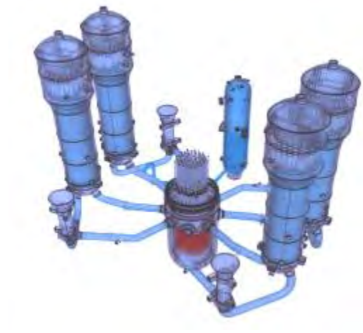
Figura 22. Il reattore PWR a quattro loop
