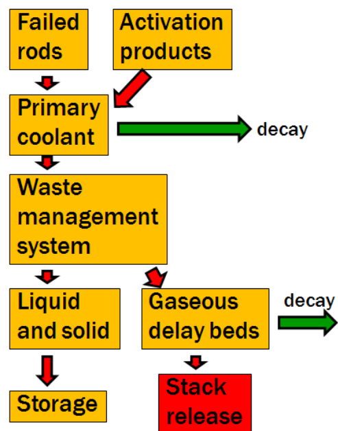
Figura 2. Sistema di trattamento delle scorie
