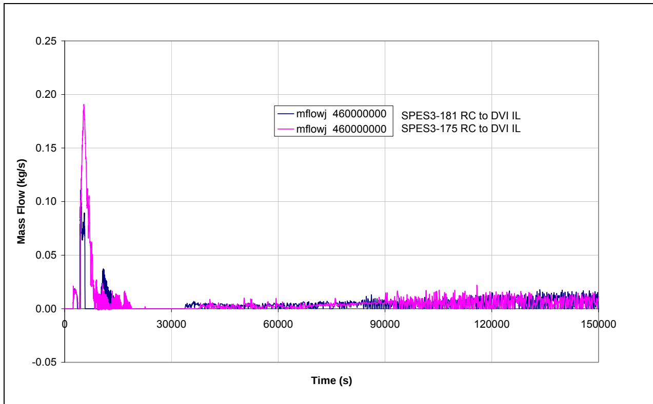
Fig.7. 37 - SPES3-181 and SPES3-175 RC to DVI mass flow IL
