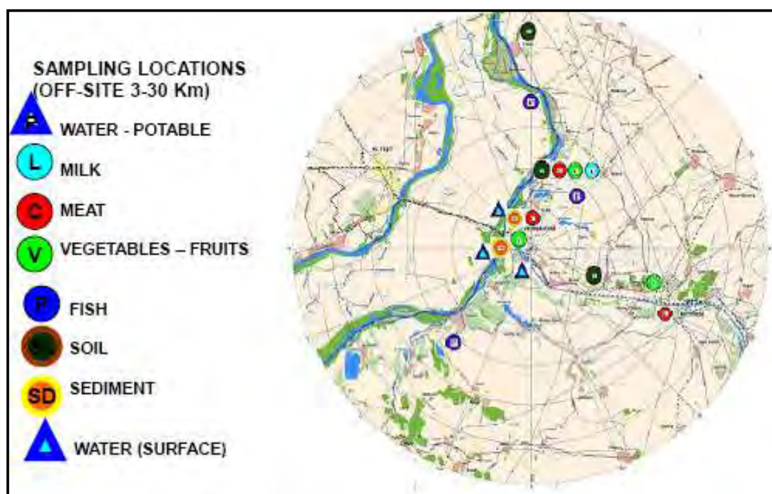
Figura 6. Punti di campionamento nella zona 3-30 km fuori dal sito di Cernovoda (Romania) (16).
