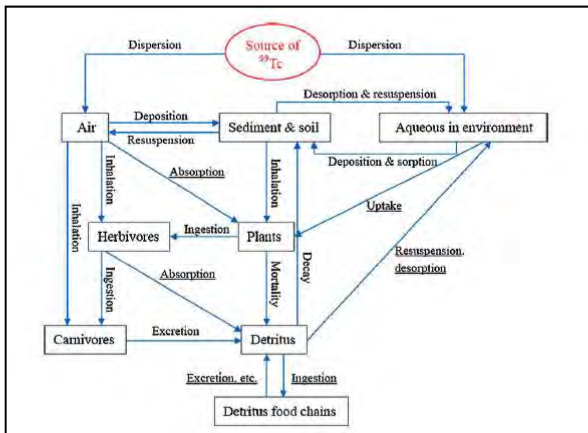
Figura 14. Possibili processi di trasporto del ^{99}\text{Tc} nell'ecosistema (21).
