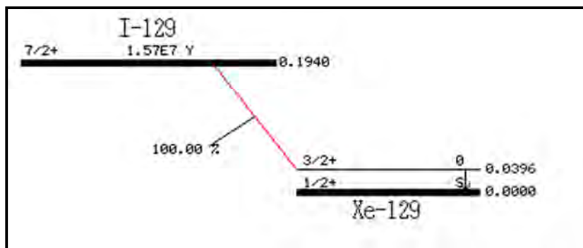
Figura 12. Decadimento dello iodio 129 (fonte: INFN).
