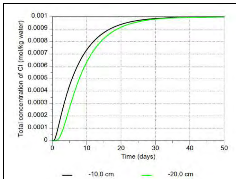
Figura 1. Andamento della concentrazione di Cloro in funzione del tempo per profondità differenti [24].
