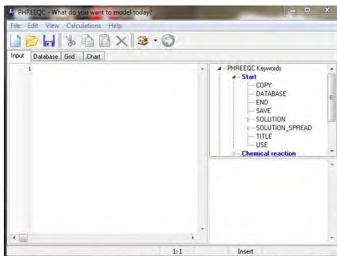
Figura 9. Schermata principale codice PHREEQC.
