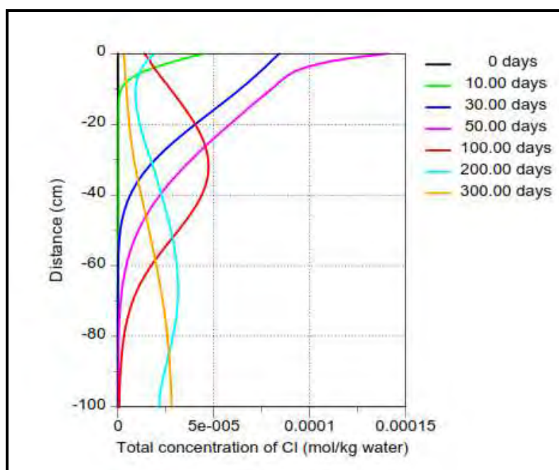
Figura 2. Andamento della concentrazione del Cloro in funzione della profondità dalla sorgente per differenti tempi [24].
