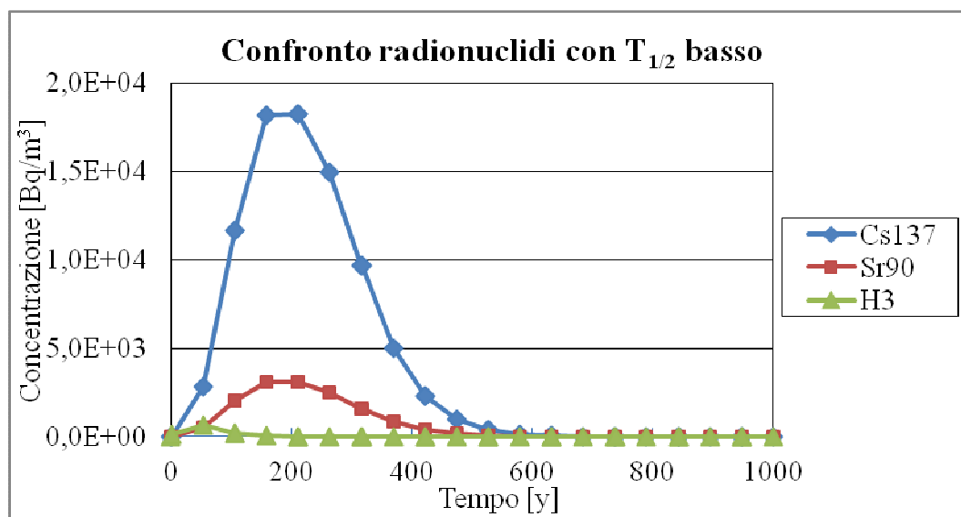
Figura 17. Confronto concentrazioni ^{137}\text{Cs} , ^{90}\text{Sr} e ^3\text{H} ad una distanza di 250 m dal deposito.
