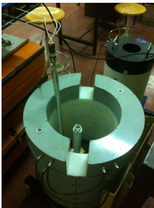
Fig. 3 - Configurazione sperimentale utilizzata per la determinazione della curva caratteristica del rivelatore.
