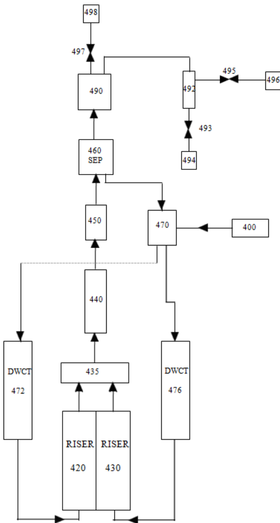
Fig. 3: Nodalizzazione Relap del secondario del generatore di vapore del loop A di SPES – 99.
