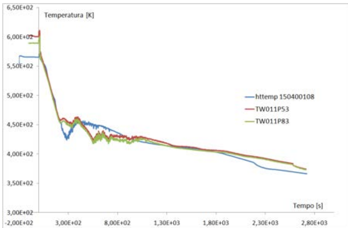
Fig.7: Andamento della temperatura di parete nella parte bassa del canale scaldante.
