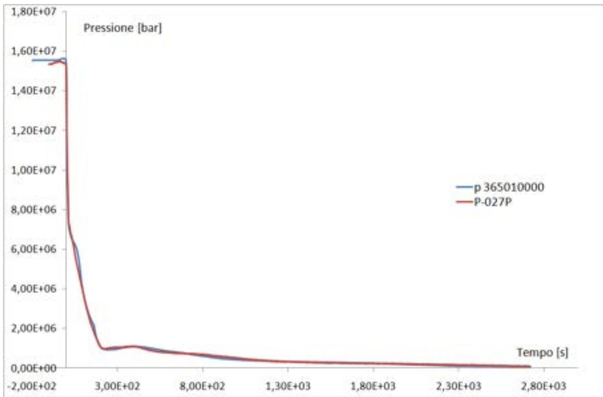
Fig. 4: Andamento della pressione nel pressurizzatore.
