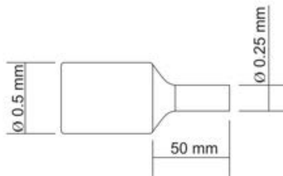
Figura 9 Sketch delle termocoppie rastremate che verranno fissate sulla barrette.
