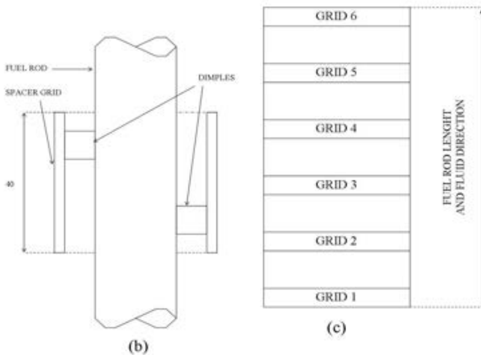
Figura 1.3: (a) Vista dall'alto del sottocanale con; (b) vista laterale del sottocanale con griglietta (notare il posizionamento sfalsato delle dimples); (c) posizione delle grigliette sulla lunghezza della barretta (le misure sono in millimetri).
