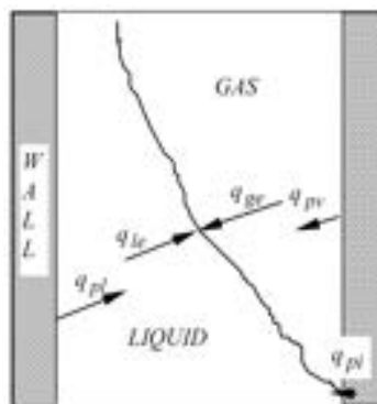
Figura 6 – Termini di trasferimento della massa e dell'energia.
