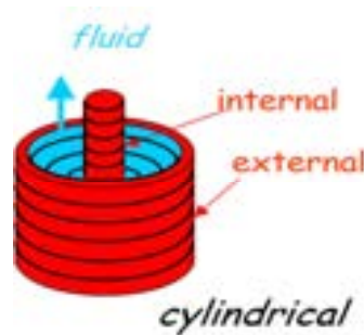
Figura 4 – Accoppiamento tra pareti in geometria cilindrica e fluido.
