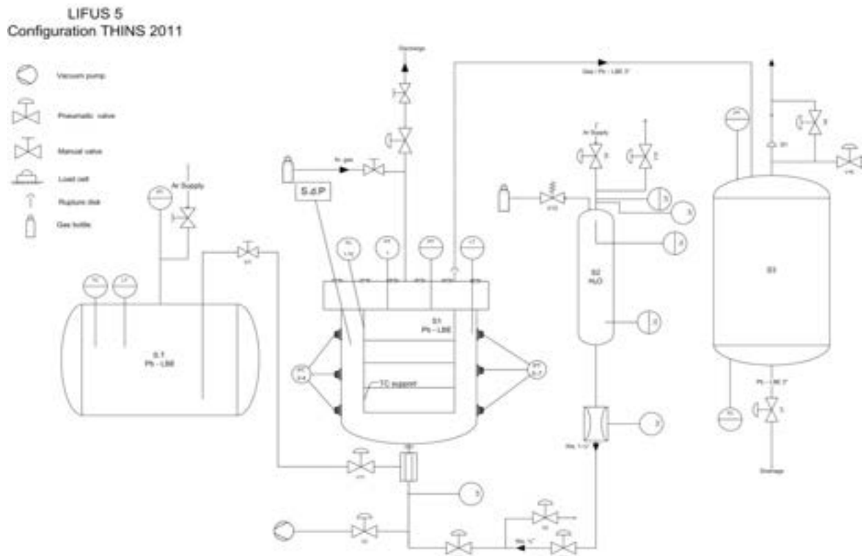
Figura 2.1. P&I dell'apparecchatura LIFUS 5.
