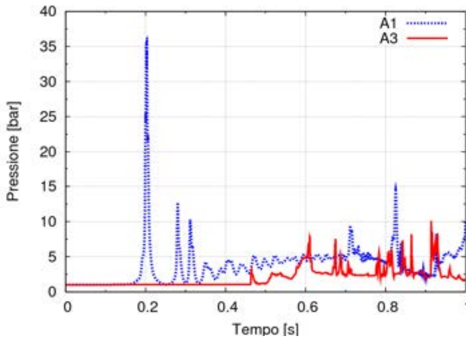
Figura 5.24. Confronto tra gli andamenti di pressione relativi ai test A1 e A3.
