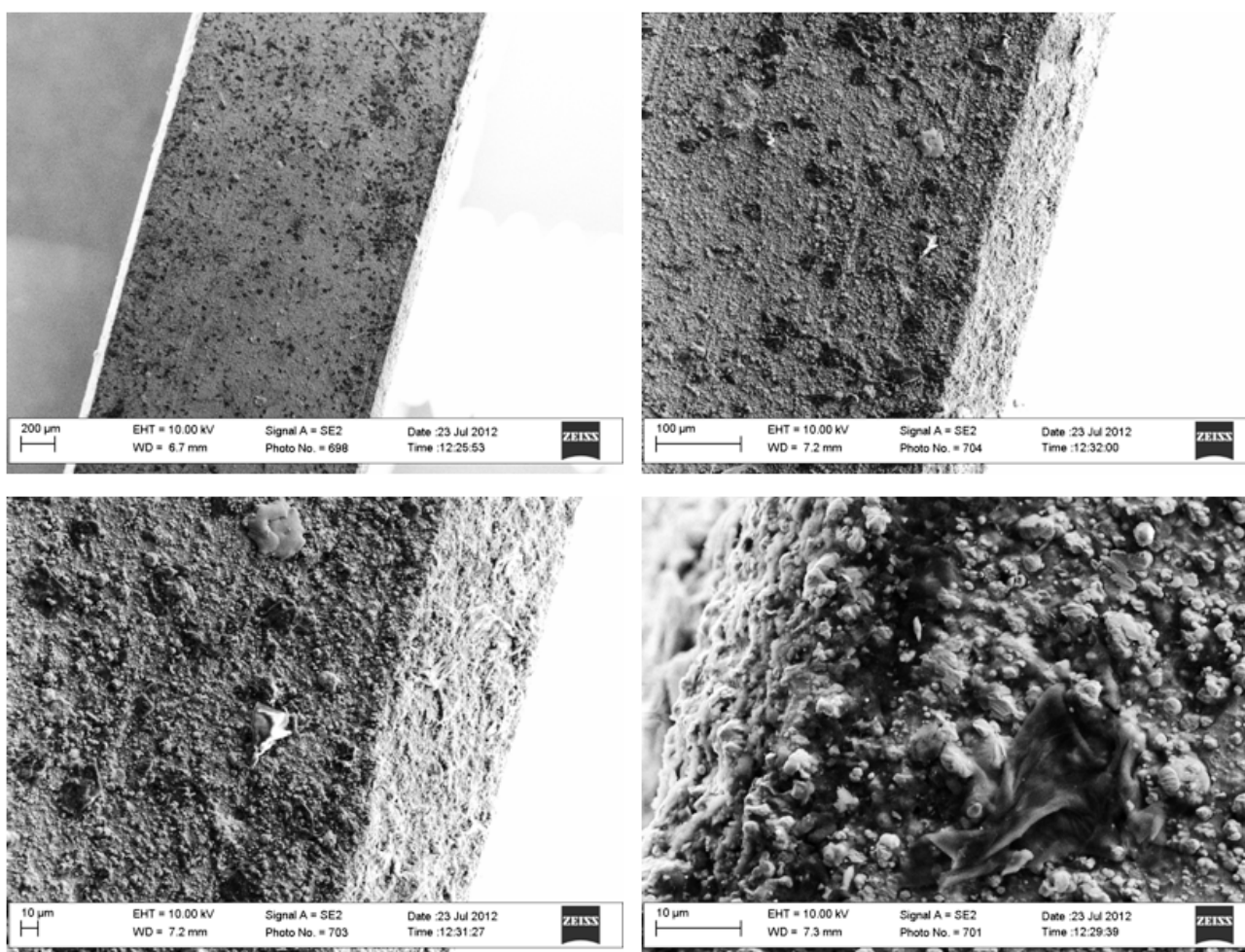
Figura 51. Micrografie SEM del rivestimento 66/12 (i.e. FeCrAl) sul substrato 316 dopo prova di flessione, freccia massima 1.5 mm.
