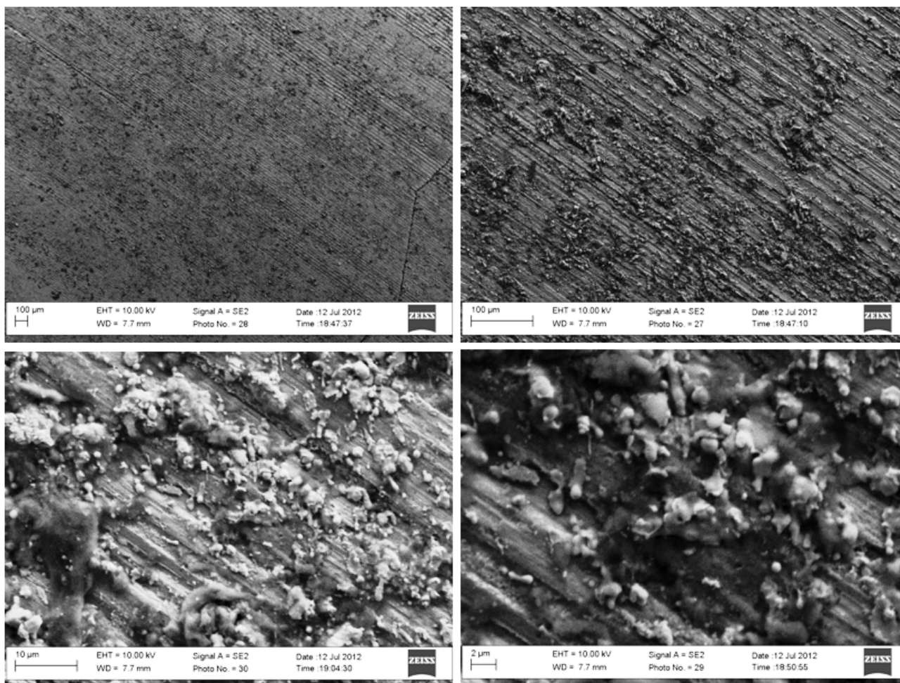
Figura 27. Micrografie SEM della superficie della sorgente FeAl.
