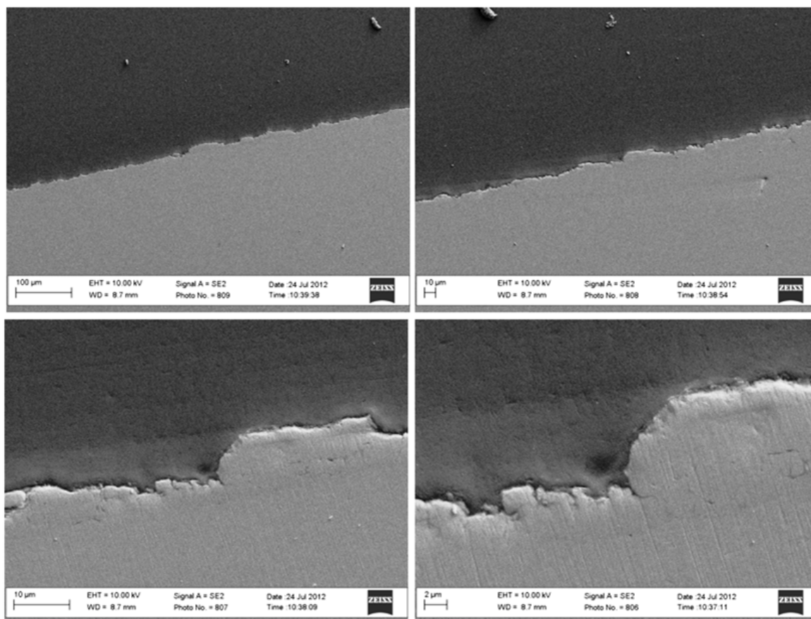
Figura 49. Micrografie SEM della cross section del provino 66/12 su P91.
