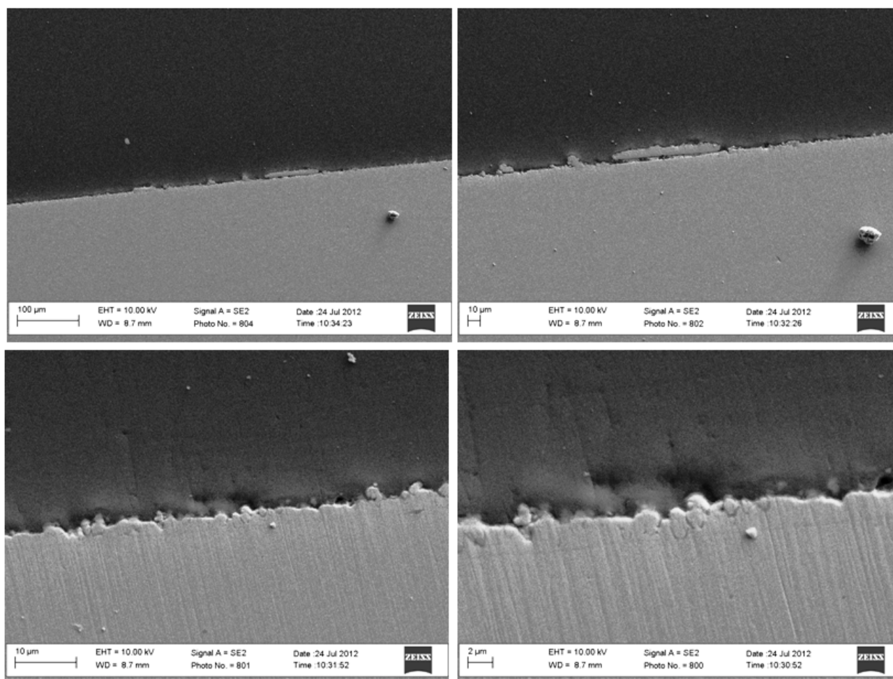
Figura 50. Micrografie SEM della cross section del provino 66/12 su 316.
