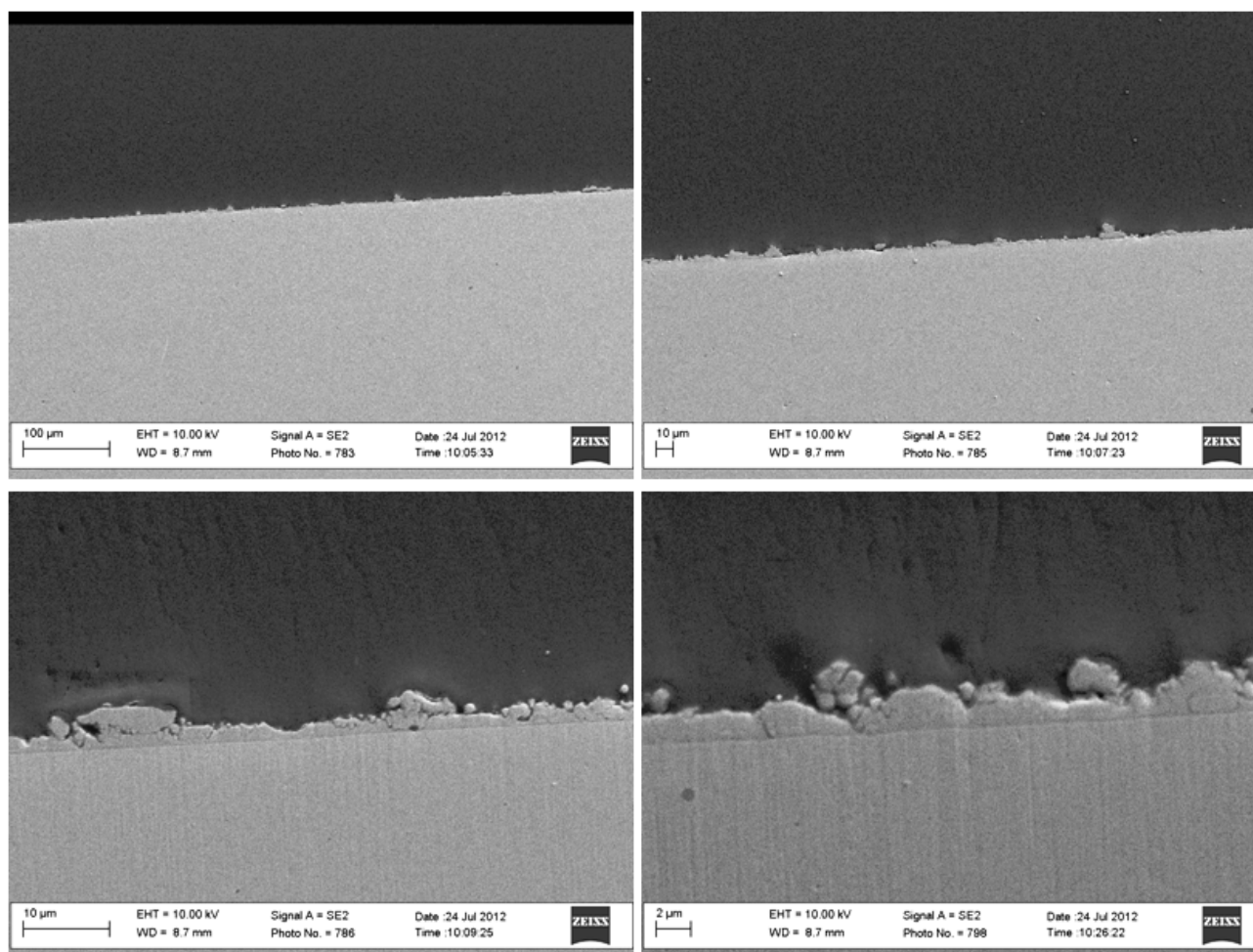
Figura 36. Micrografie SEM della cross section del provino 64/12 su 316.
