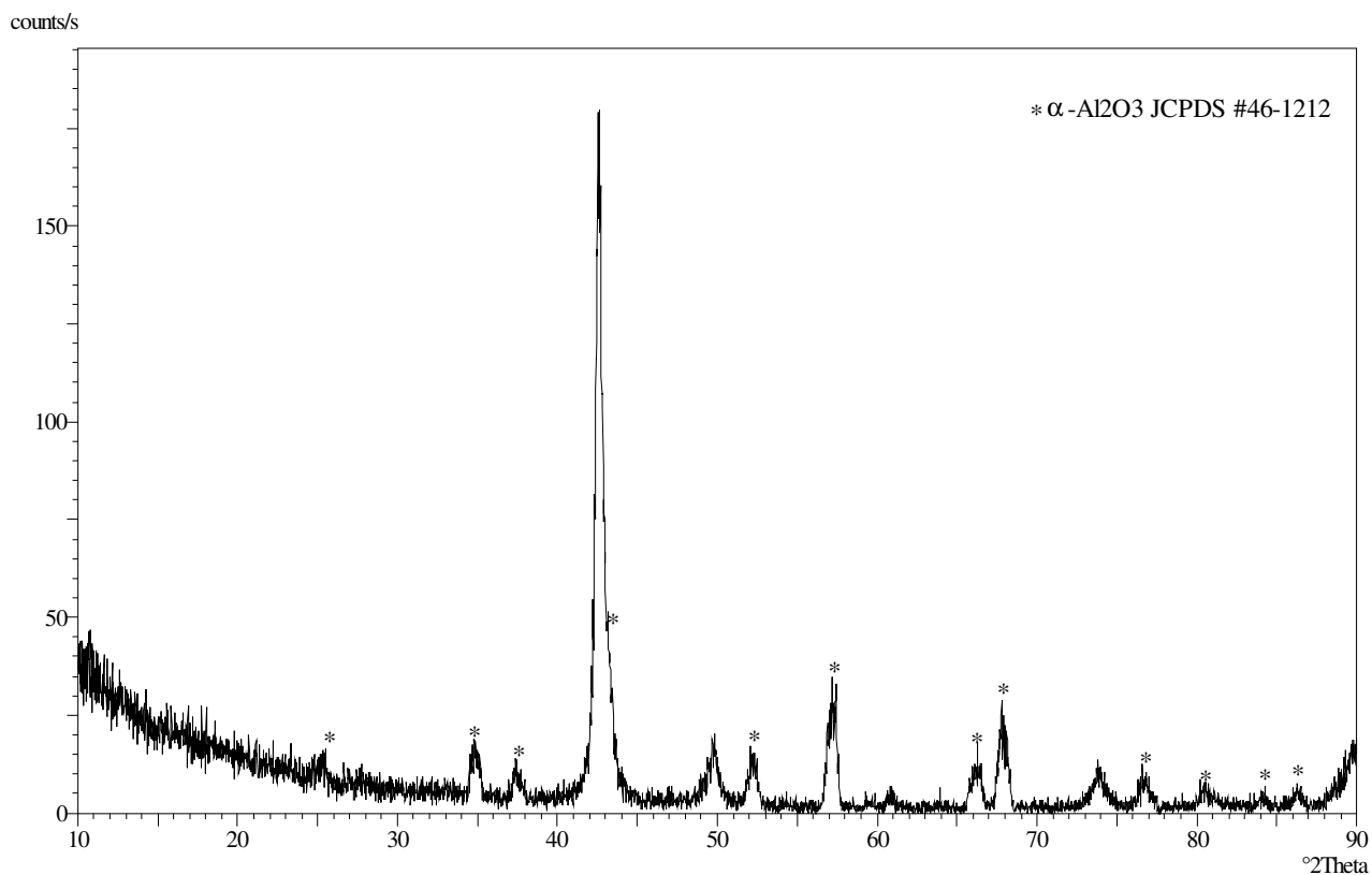
Figura 40. Pattern XRD del target FeCrAl sottoposto a analisi termica fino a 1600 °C.
