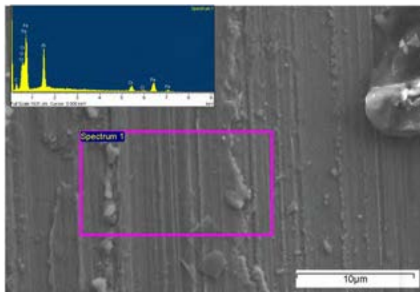
Figura 43. Micrografia SEM e spettro EDS della superficie della sorgente FeCrAl.
