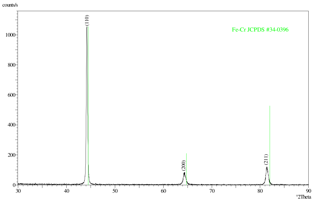
Figura 41. Pattern di diffrazione XRD della sorgente FeCrAl.
