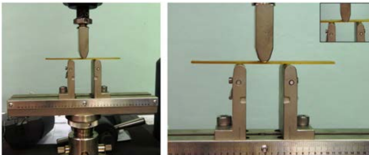
Figura 1. Set-up sperimentale della prova di bending a tre punti.
