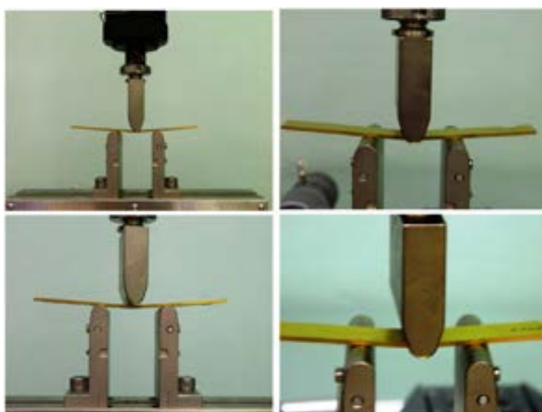
Figura 18. Foto digitali del substrato 316 rivestito con TiN dopo prova di bending a tre punti.
