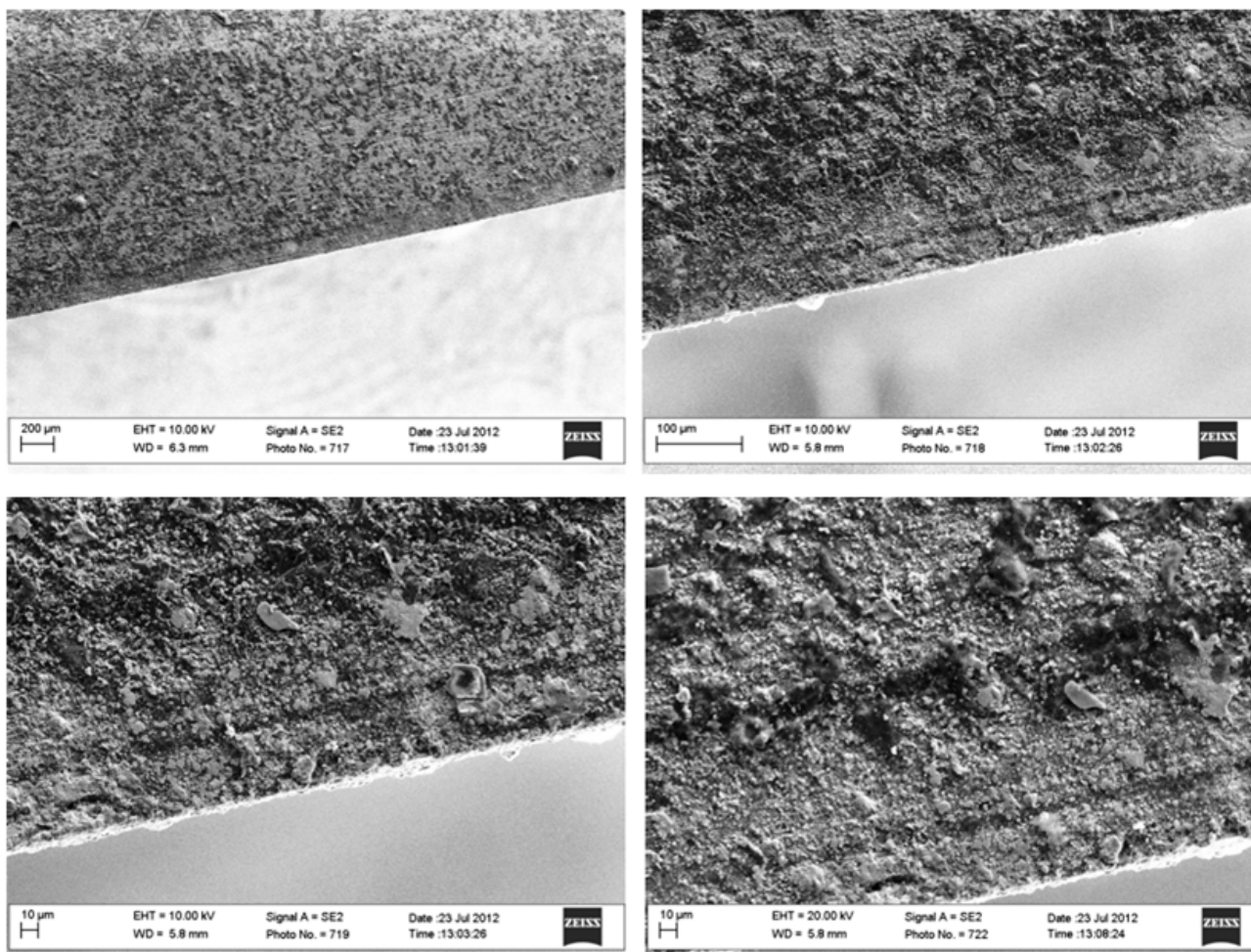
Figura 37. Micrografie SEM del rivestimento 64/12 (i.e. FeAl) sul substrato 316 dopo prova di flessione, freccia massima 1.5 mm.
