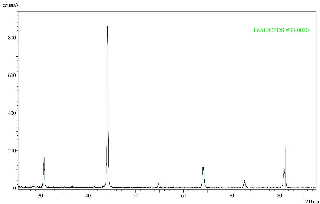
Figura 26. Pattern di diffrazione XRD della sorgente FeAl.
