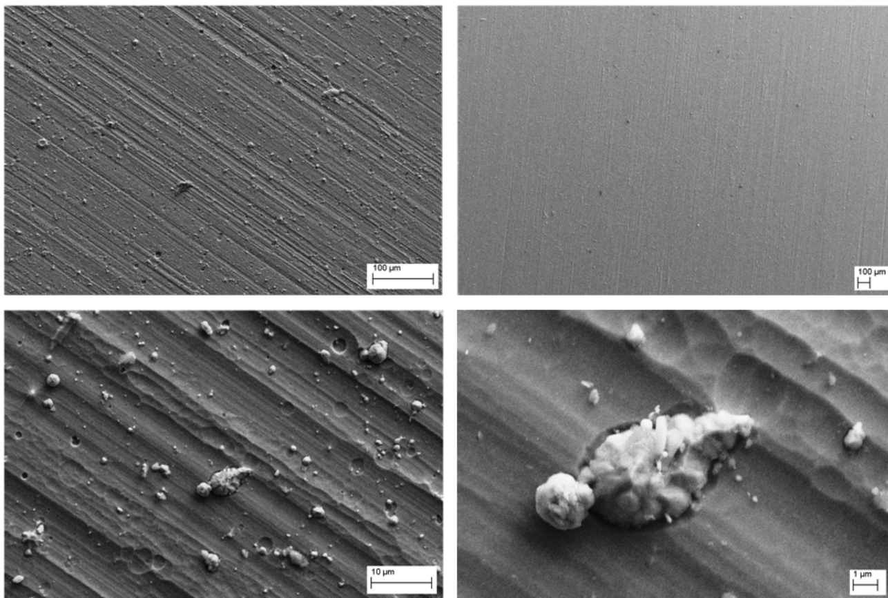
Figura 9. Micrografie SEM del coating di TiN 58/12 su 304.
