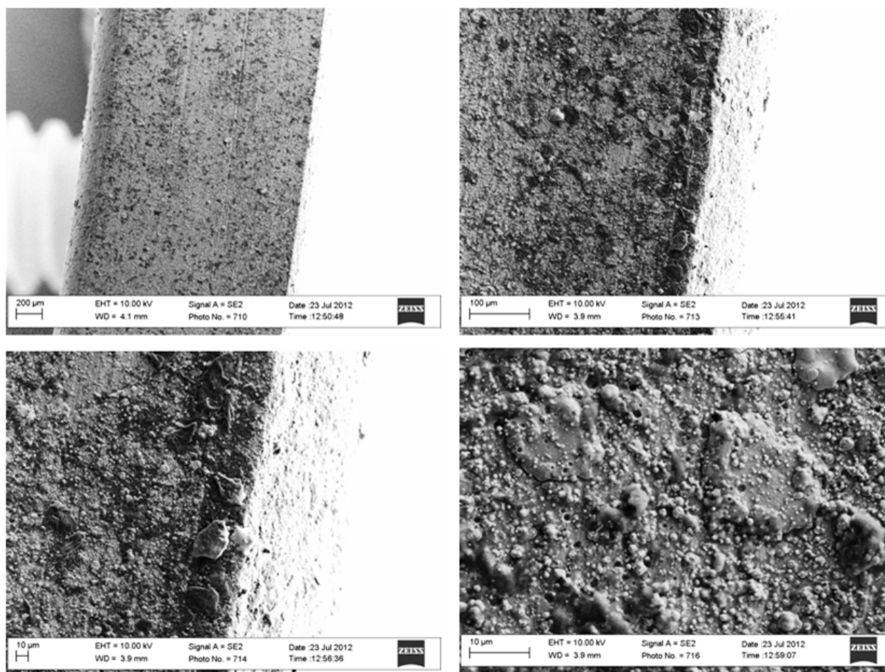
Figura 38. Micrografie SEM del rivestimento 64/12 (i.e. FeAl) sul substrato 316 dopo prova di flessione, freccia massima 2.0 mm.
