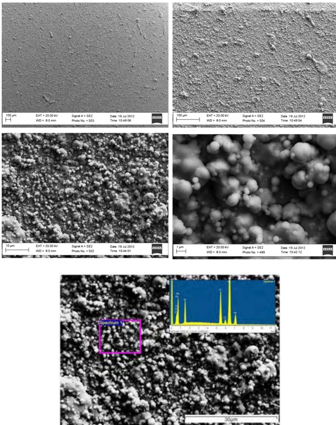
Figura 49. Micrografie SEM e analisi EDS del coating di FeCrAl 66/12 su 441.
