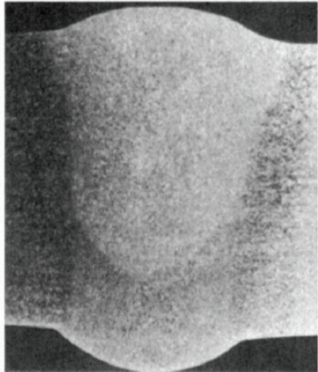
Fig. 17 – Confronto fra le zone di saldatura delle tecniche Laser e TIG: a sinistra la zona della tecnica LASER, a destra quella TIG.
