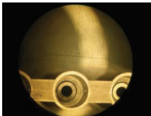
Fig. 26 – Visione del canale laterale che collega le 4 posizioni (a sinistra), accoppiamento barretta/griglia prima della saldatura interna: si nota che la parte superiore del provino barretta deve essere a filo del piano interno della griglia in cui viene effettuata la saldatura (a destra)
