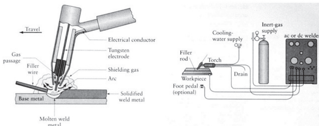
Fig. 16 – Schematizzazioni della saldatura TIG
