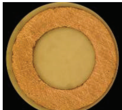
Fig. 40 – Particolare della finitura della guarnizione in rame realizzata per tornitura e lucidata (visione ingrandita al microscopio ottico)
