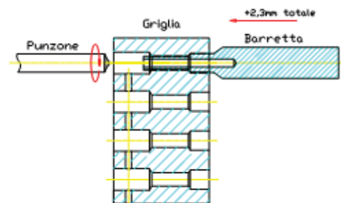
Fig. 36 - Sequenza fasi per ottenere giunto per "imbutitura"
