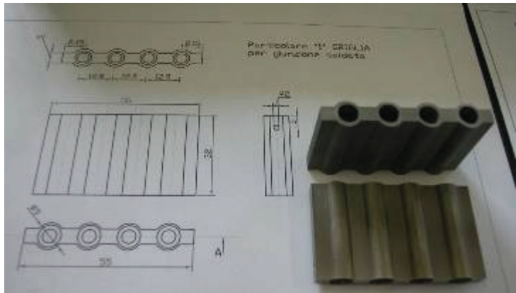
Fig. 22 - Griglie per saldatura (stringhe da 4 fori, dis. J 50 0119)
