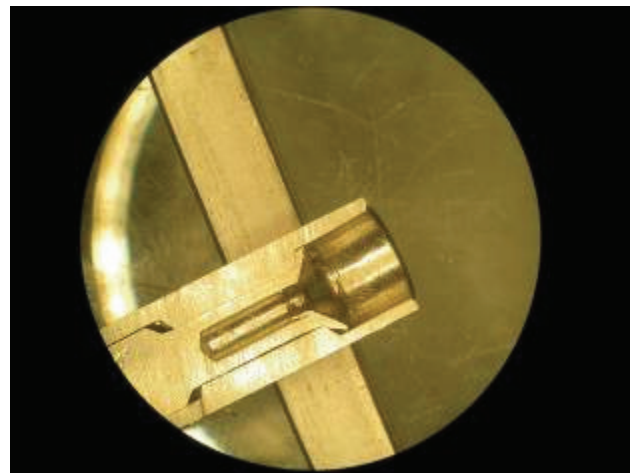
Fig. 33 – Foto in alto: provino PPB-1 tagliato in sezione per verificare l'accoppiamento della deformazione del provino barretta rispetto alla griglia; in basso visioni al microscopio ottico di tale accoppiamento non ancora ottimale
