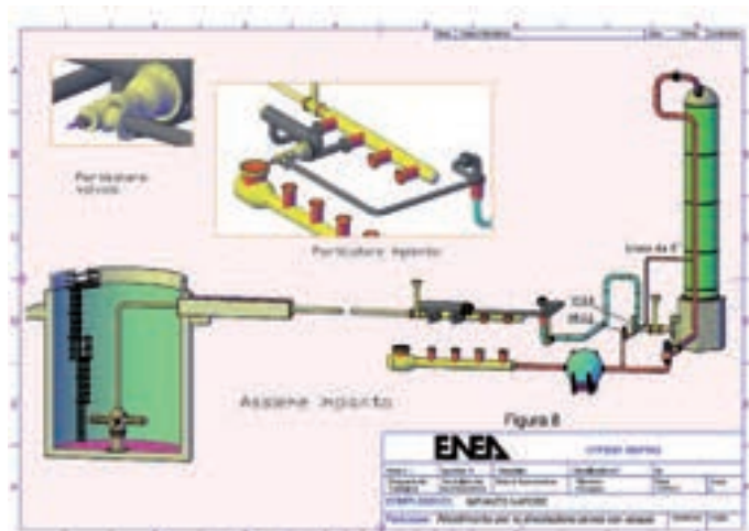
Schema (in scala) dell'installazione della valvola prototipo su VAPORE per prove con miscela acqua-vapore
