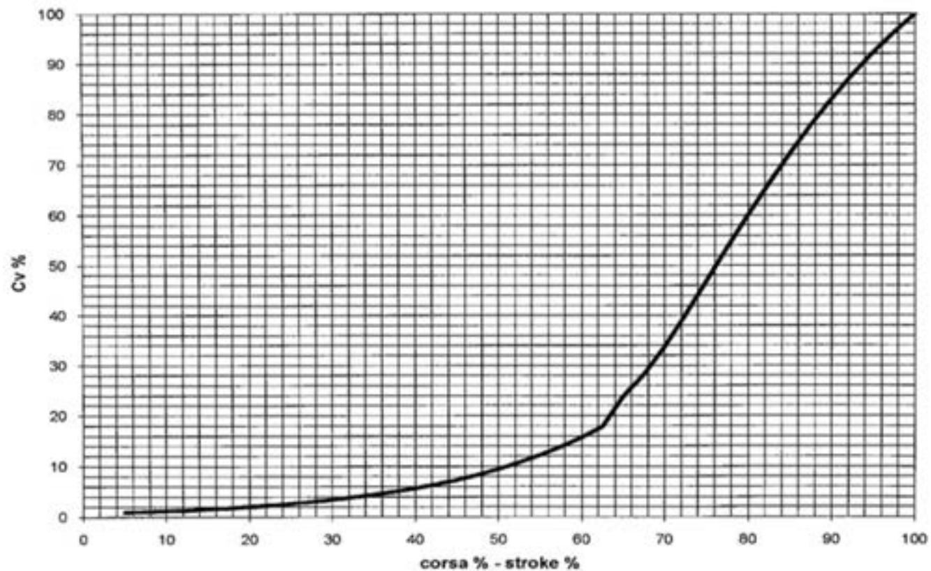
Fig. 9 : Curva caratteristica del prototipo da provare
