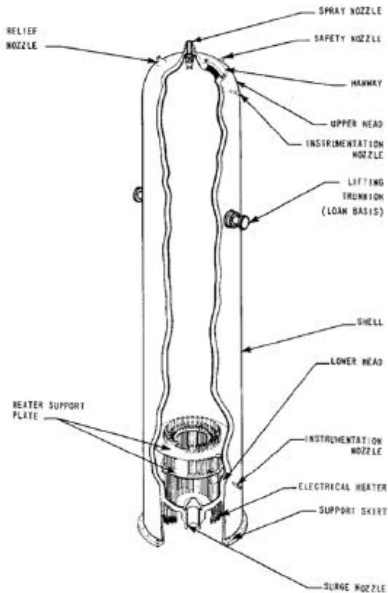
Fig. 2 : esempio tipico di pressurizzatore per reattori PWR, completo di resistenze elettriche scaldanti
