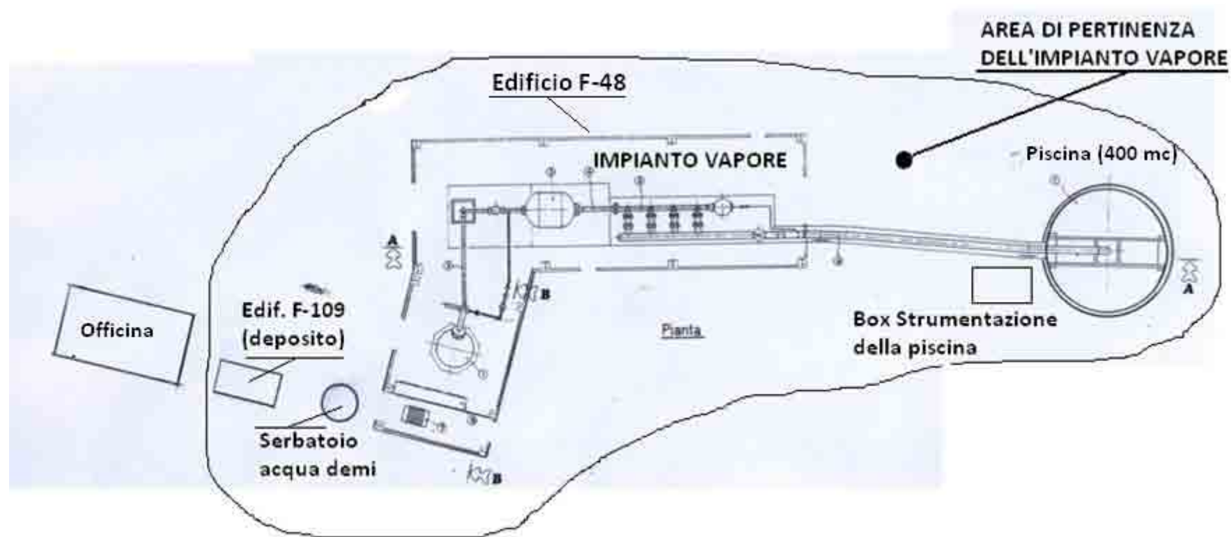
Fig. 20 : Area di competenza dell'impianto VAPORE (schema indicativo)
