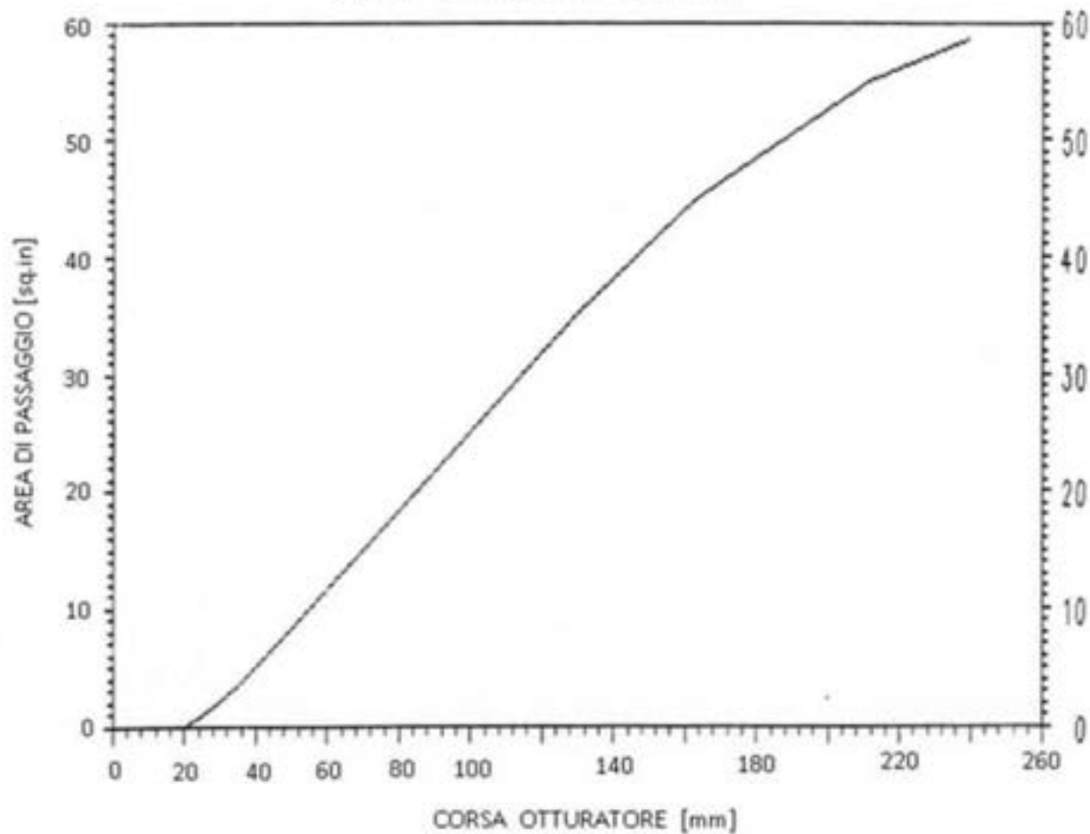
Fig. 12 – A : Valvola VL 1; relazione tra flow area e corsa otturatore
