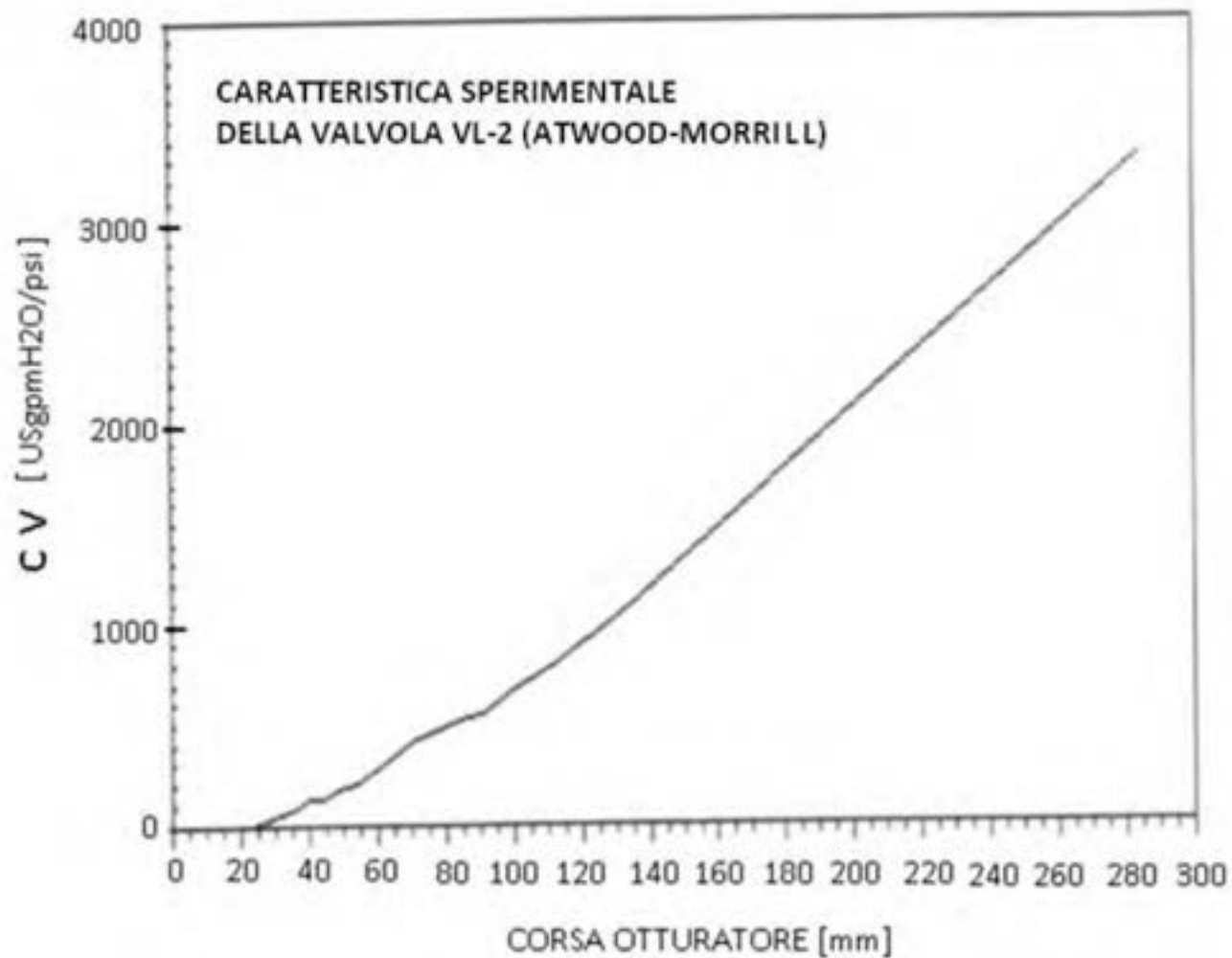
Fig. 12-B : Valvola VL2 ; caratteristica di regolazione
