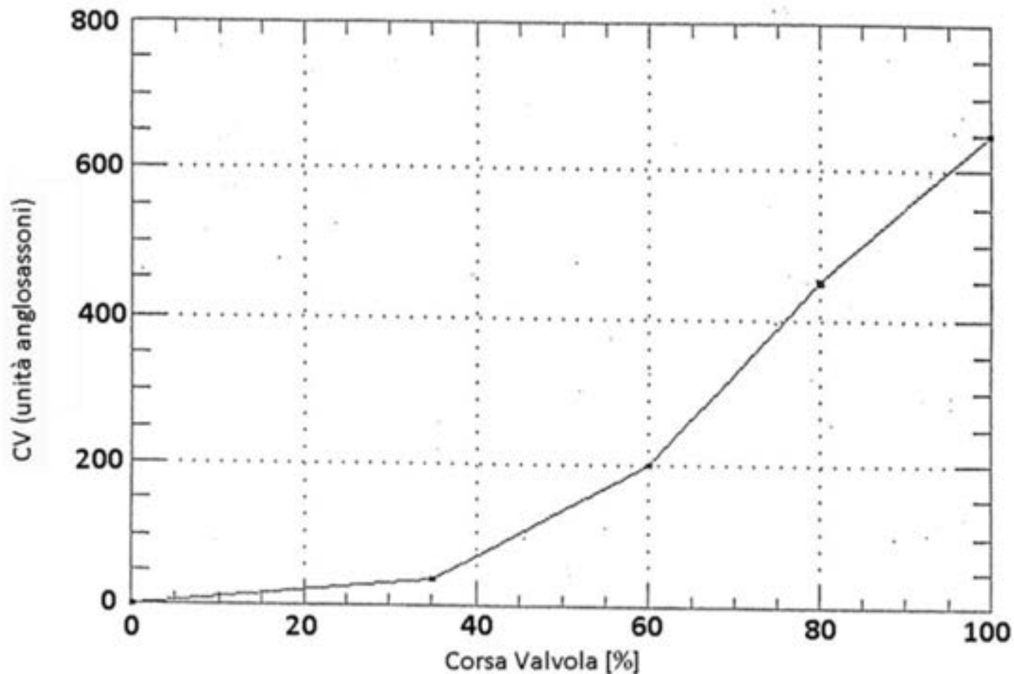
Fig. 10 : CV della valvola di regolazione principale VR 1.1 dell'impianto VAPORE. Andamento ottenuto da elaborazione di dati sperimentali
