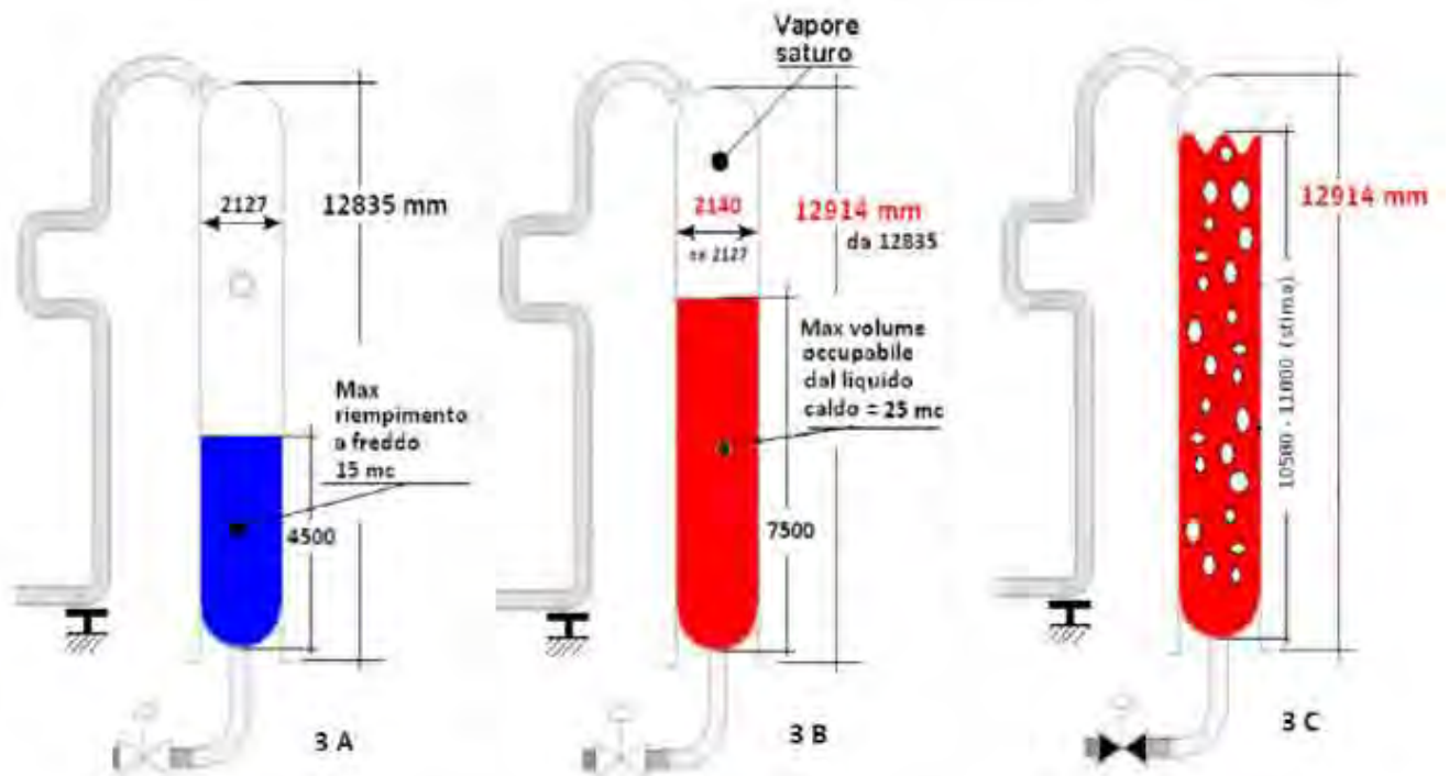
fig 3 : fasi operative tipiche per la corretta gestione del pressurizzatore dell'impianto VAPORE: A= riempimento a freddo; B= situazione al raggiungimento della max condizione di esercizio ( 180 bar e T = 365 °C ) ; C= scarico di alta portata di vapore con swelling dell'acqua
