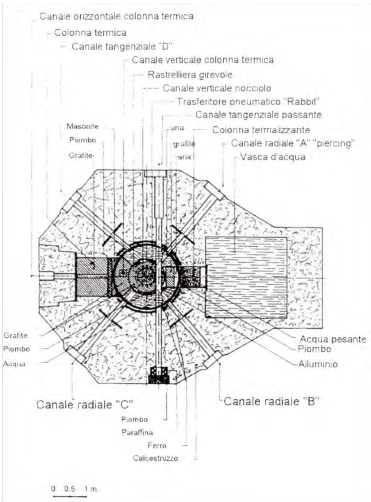
Figura 1 - Sezione orizzontale del reattore TRIGA RC-1
