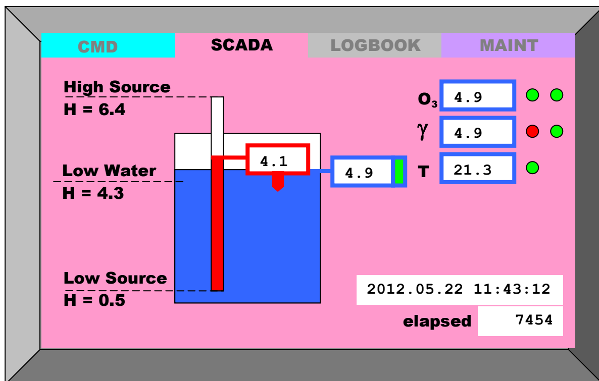
Fig. 37: Schermata SCADA
