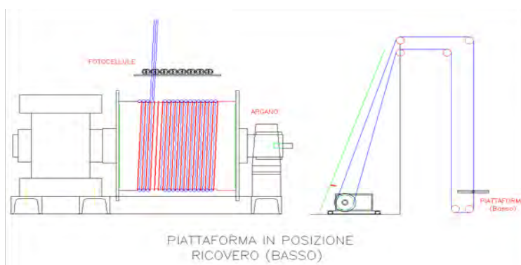
Fig. 54: Sistema di fotocellule ed argano (schema e foto seguenti) con piattaforma in posizione di ricovero
