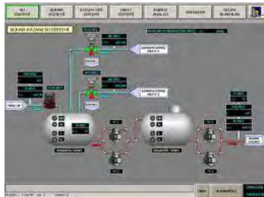
Fig.10: Interfaccia SCADA
