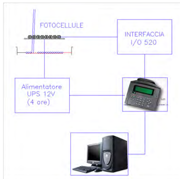
Fig. 53: Schema a blocchi del sistema di monitoraggio ed acquisizione
