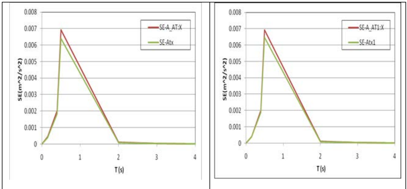
Figura 53 - Asse X - marker AT:Y, AT1Y(sistema 3DVision) - accelerometri Aty e Aty1(STEX)
