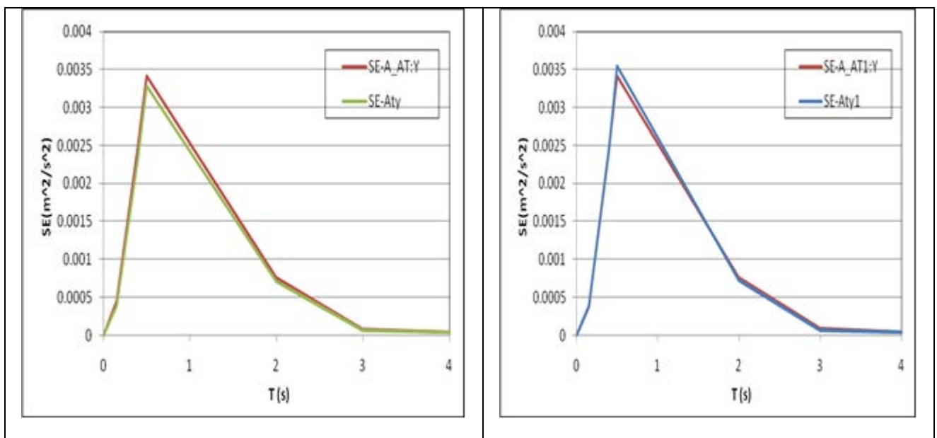
Figura 54 - Asse Y - marker AT:X, AT1X(sistema 3DVision) - terne accelerometri Atx e Atx1(STEX)
