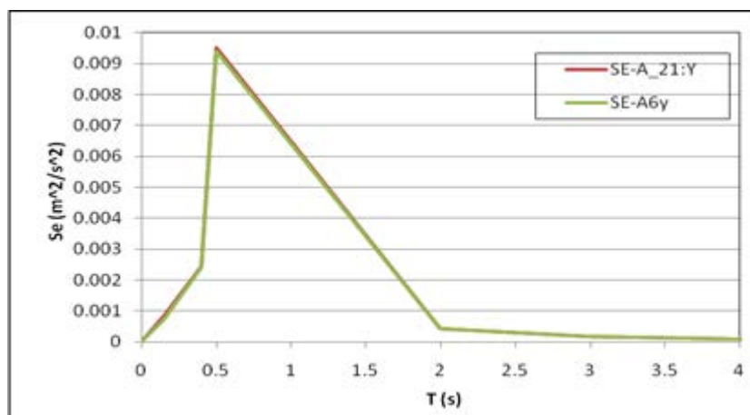
Figura 90 - Confronto ai diversi livelli marker (sistema 3DVision) – accelerometri
