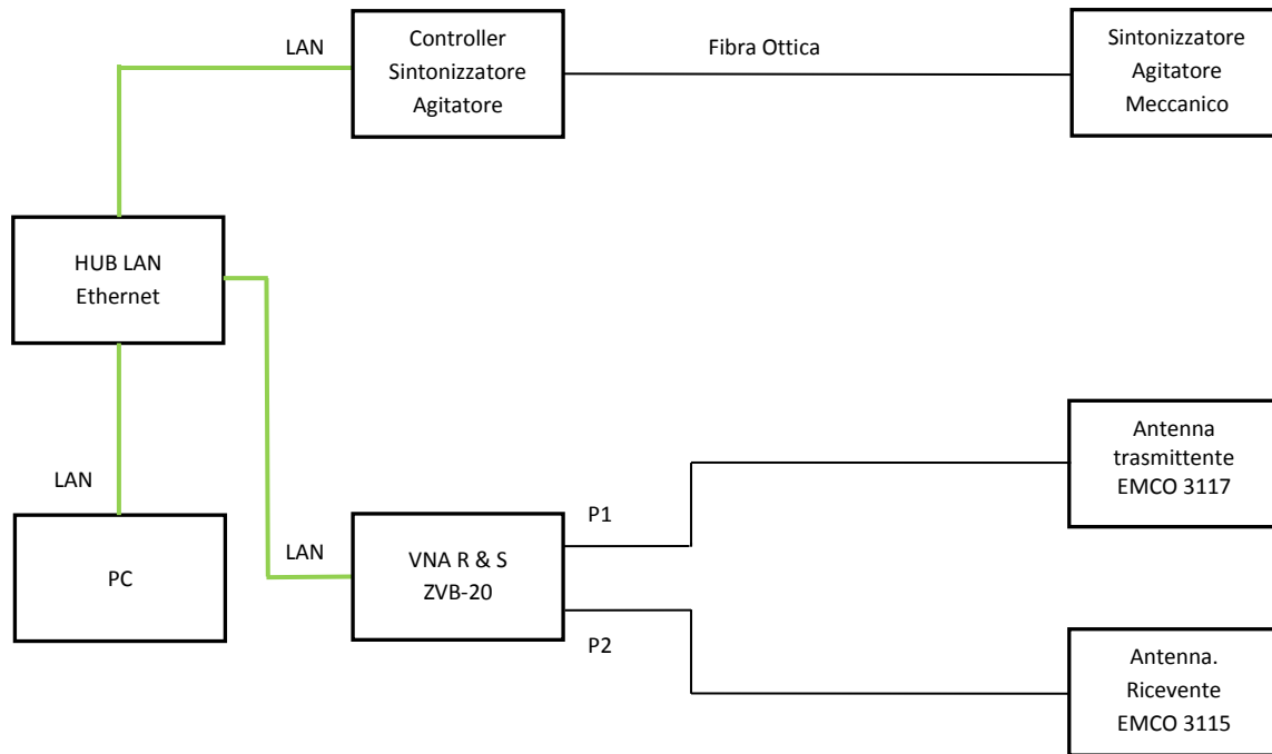
Figura 6 - Schema a blocchi della catena sperimentale per la taratura della camera reverberante nella banda 1 GHz – 18 GHz.
