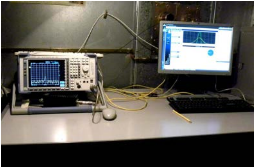
Figura 7 - Viste parziali del banco di misura
