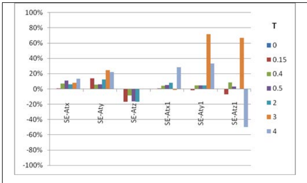
Figura 68 - Confronto in termini % dello spettro di energia Se(T, ζ) per i periodi T tra marker AT - terna accelerometrica At e marker AT1-terna accelerometrica At1
