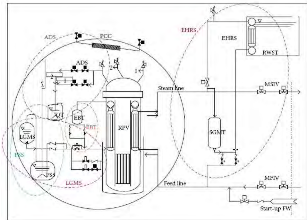
Figura 4-3: Schema del contenimento e dei sistemi di sicurezza tipici del reattore IRIS.
