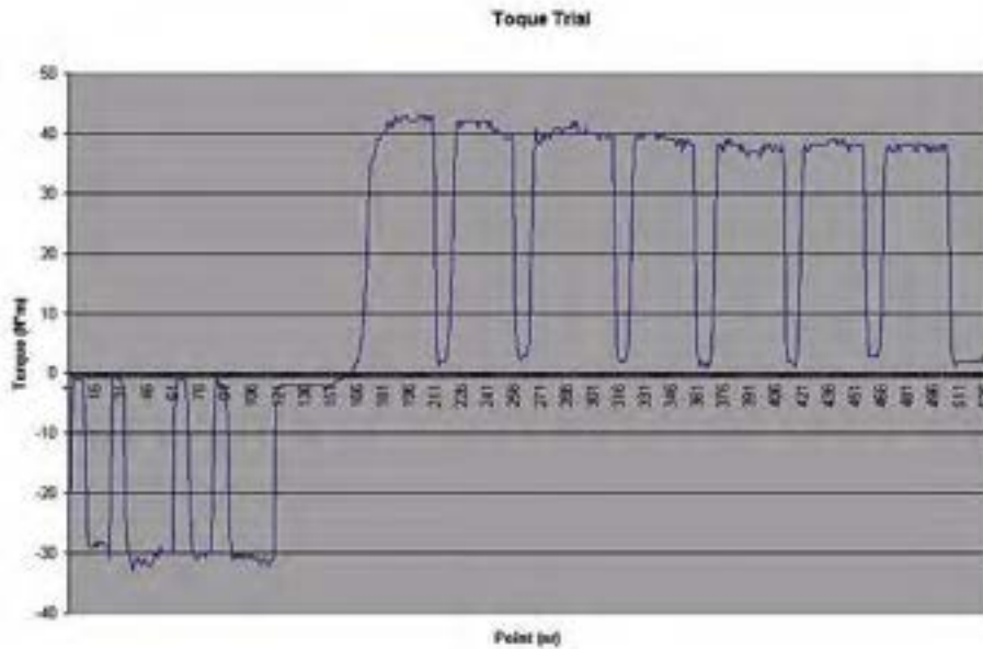
Fig. 36 Monitoraggio coppia di serraggio pattino
