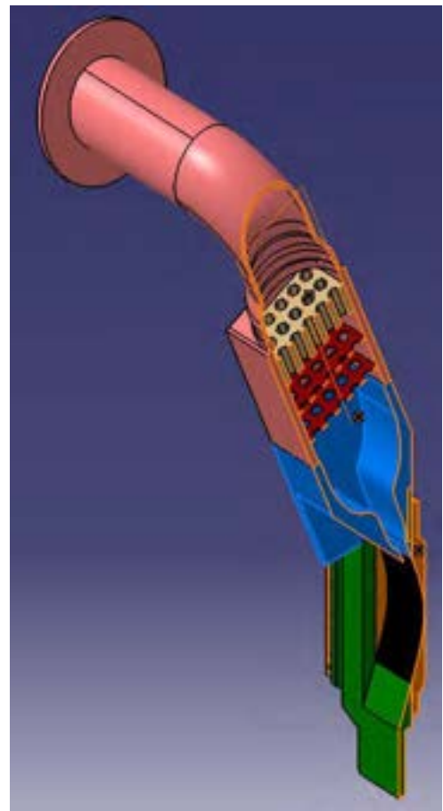
Fig. 2 Sezione del modello 3D del Target
