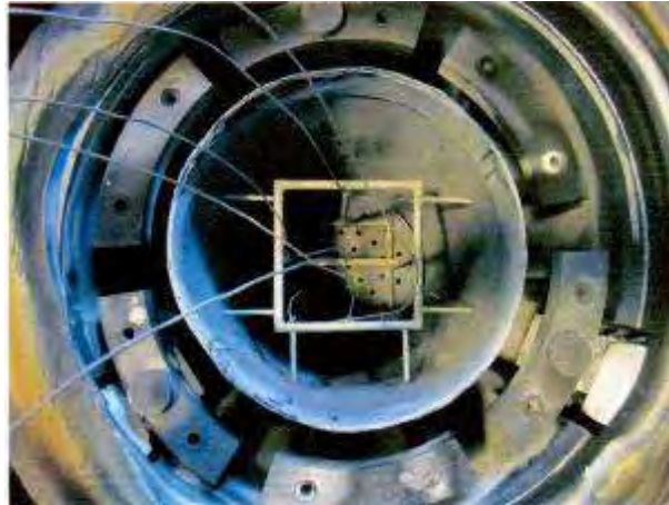
Figura 2- Particolare telaio acciaio con sensori temperatura
