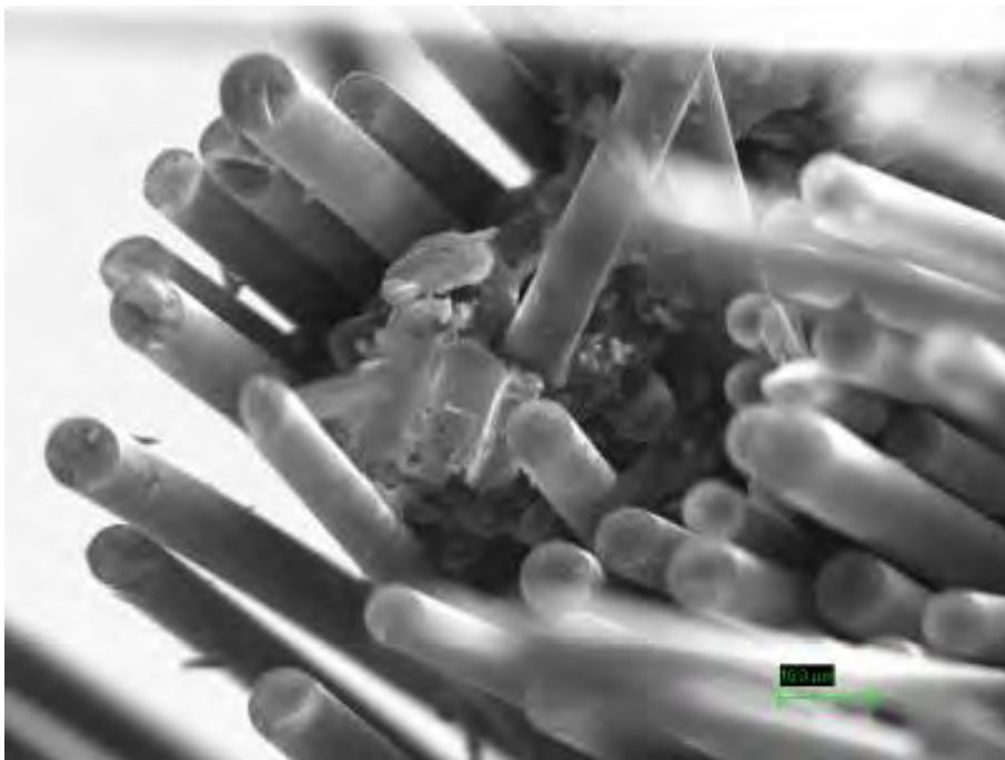
Figura 8 – Ingrandimento 2.50 kX
