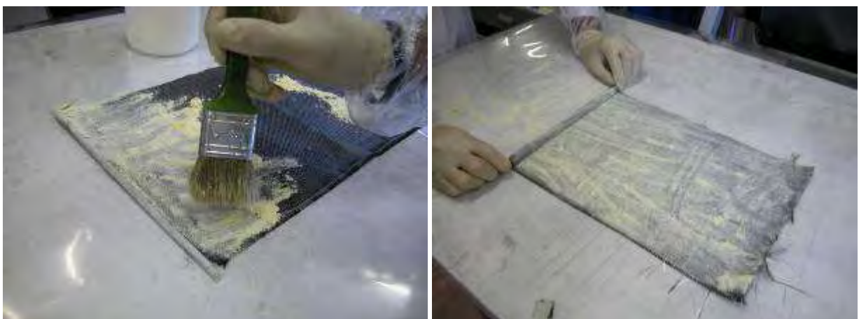
Figura 12 – Impregnazione con resina fenolica in polvere e avvolgimento tubo
