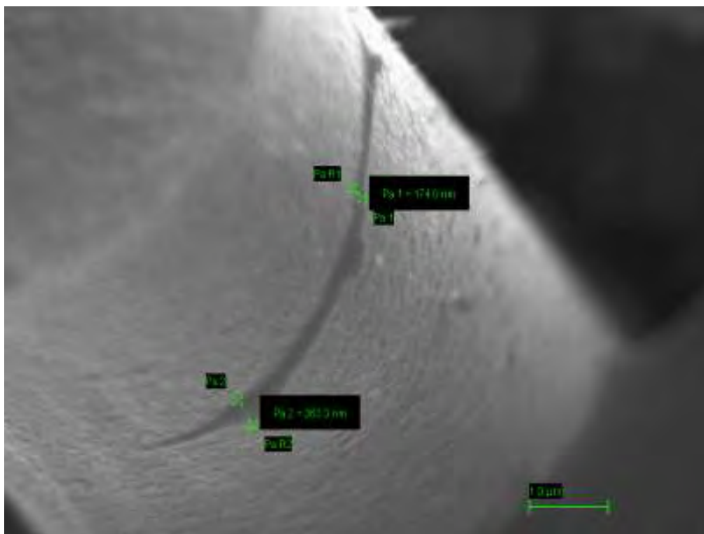
Figura 6 – Ingrandimento 30.00 kX
