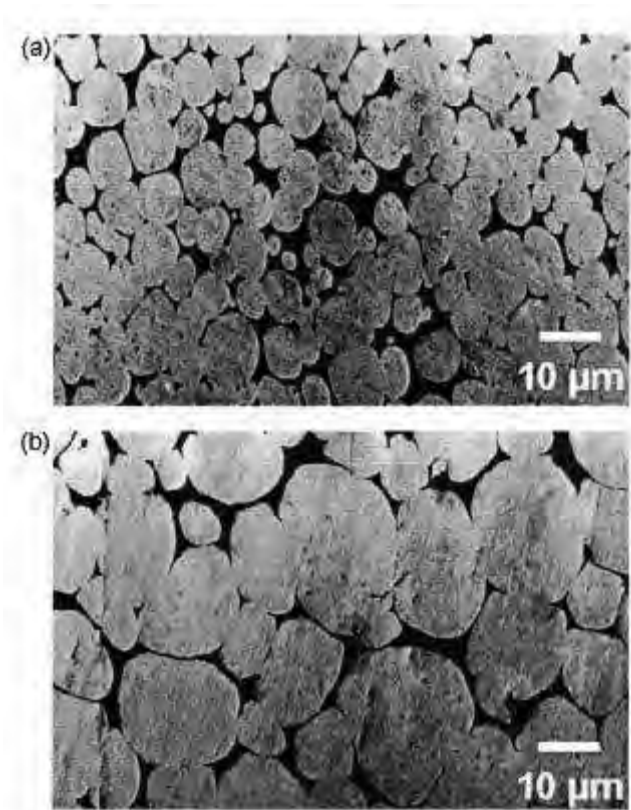
Fig. 6 – Microstrutture leghe W-Ni-Fe a confronto: (a) sinterizzazione a microonde, (b) sinterizzazione convenzionale
