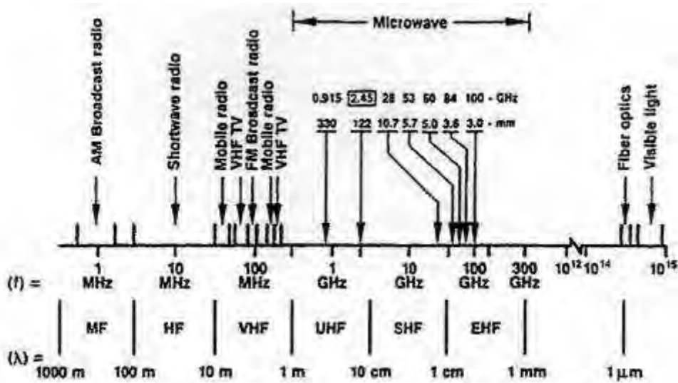
Fig. 1 – Spettro elettromagnetico e frequenze impiegate nei processi a microonde
