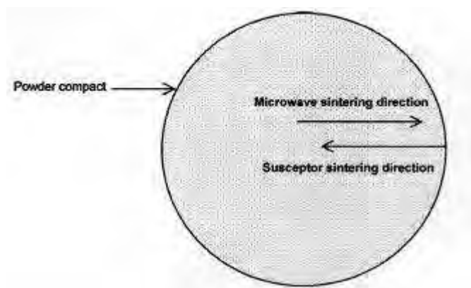
Fig. 3 – Direzioni delle due sorgenti di calore nel sistema di riscaldamento ibrido
