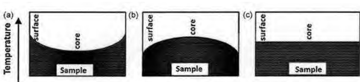
Fig. 2 – Profilo di temperatura entro il campione: a) riscaldamento convenzionale, b) riscaldamento a microonde, c) trattamento ibrido
