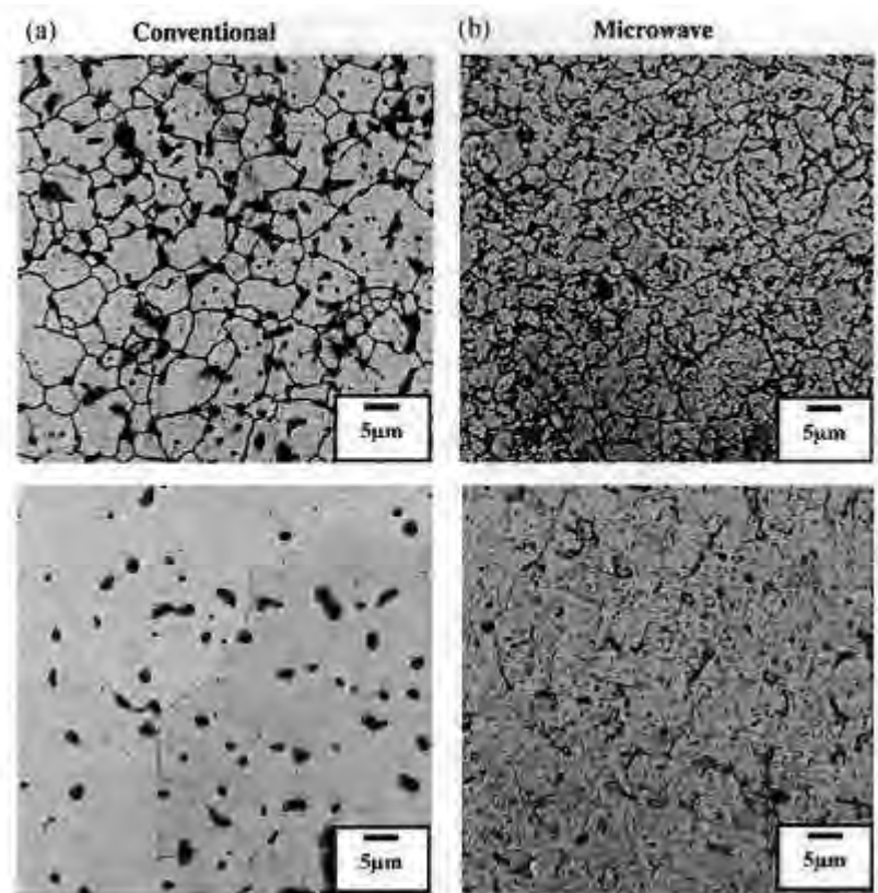
Fig. 5 – Confronto fra microstrutture di campioni in acciaio sinterizzati in modo convenzionale (a) e a microonde (b)
