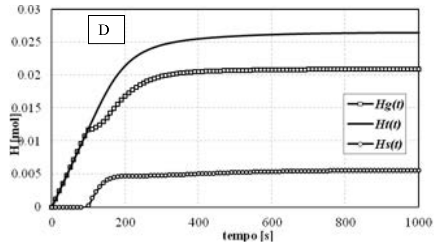
Figura 17: Hold-up di CO 2 nella fase gas dell'intero sistema H_G(t) , nell'idrotalcite H_s(t) e H_t(t) dei campioni A, B, C, D
