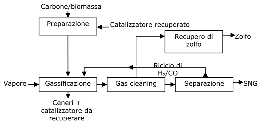
Figura1: Processo Exxon 1
