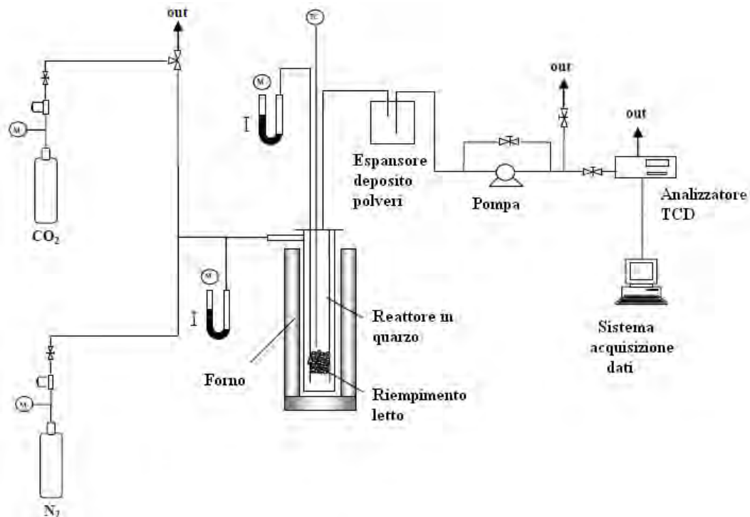
Figura 7: Schema d'impianto
