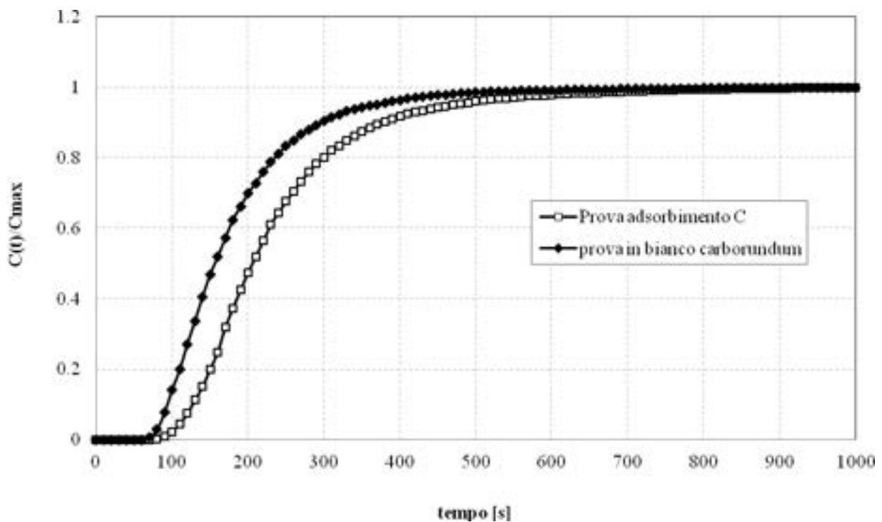
Figura 15: Confronto test di risposta a gradino con concentrazioni di CO 2 normalizzate prova adsorbimento e prova in bianco
