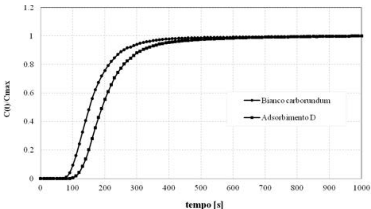
Figura 11: Confronto curve di risposta della concentrazione di CO_2 normalizzata della prova in bianco con Carborundum a condizioni ambiente di pressione e temperatura e della curva di risposta della concentrazione di CO_2 durante la prova di adsorbimento campione D.
