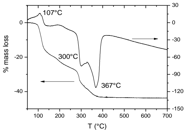
Figura 4 TG-DTA di CZ50 sol2 eseguita in aria fino a 700°C
