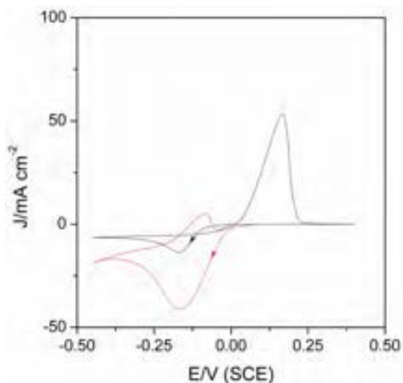
Fig 4. Ciclovoltammetria della soluzione 0.05 M di \text{CuSO}_4 e 0.25M di \text{H}_2\text{SO}_4 con elettrodi di Ni (linea rossa) e di Pt (linea nera) con velocità di scansione 10 \text{mV s}^{-1}
