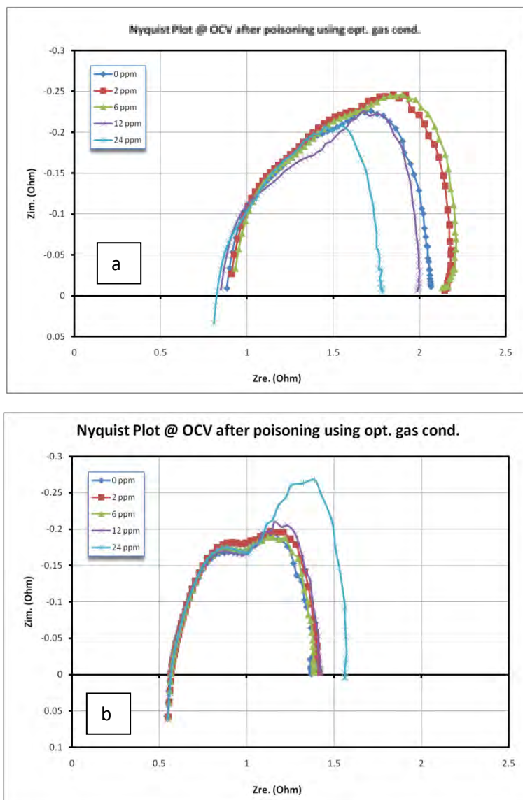
Fig.15 - Diagramma di Nyquist di anodi (a) Ni-Cr e (b) Ni-ceria a OCV durante avvelenamento con 2,6,12,24 ppm di H 2 S.
