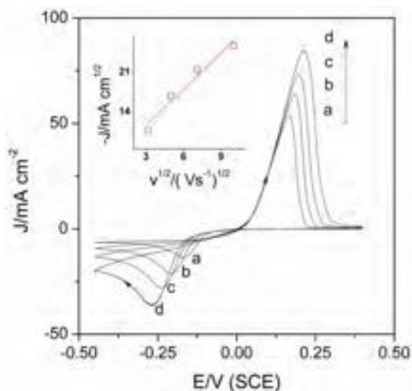
Fig 3. Ciclovoltammetria della soluzione 0.05 M di \text{CuSO}_4 e 0.25 M di \text{H}_2\text{SO}_4 con elettrodi di Pt a diverse velocità di scansione: 10 \text{mV s}^{-1} a); 25 \text{mV s}^{-1} b); 50 \text{mV s}^{-1} c); 100 \text{mV s}^{-1} d). L'inserto in figura mostra l'andamento dell'intensità del picco catodico in funzione del reciproco della velocità quadratica di scansione v^{1/2} .
