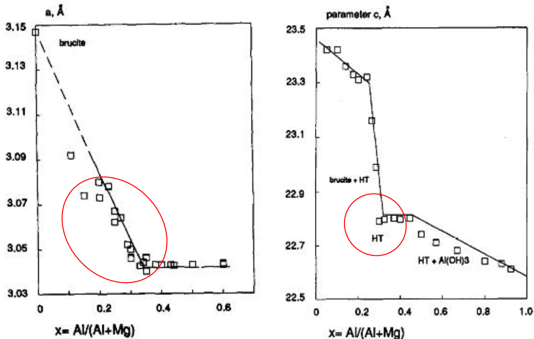
Fig 5: Parametri di cella HT in funzione del rapporto x = \text{Al}^{3+}/(\text{Al}^{3+} + \text{Mg}^{2+}) . (Vaccari et al.)
