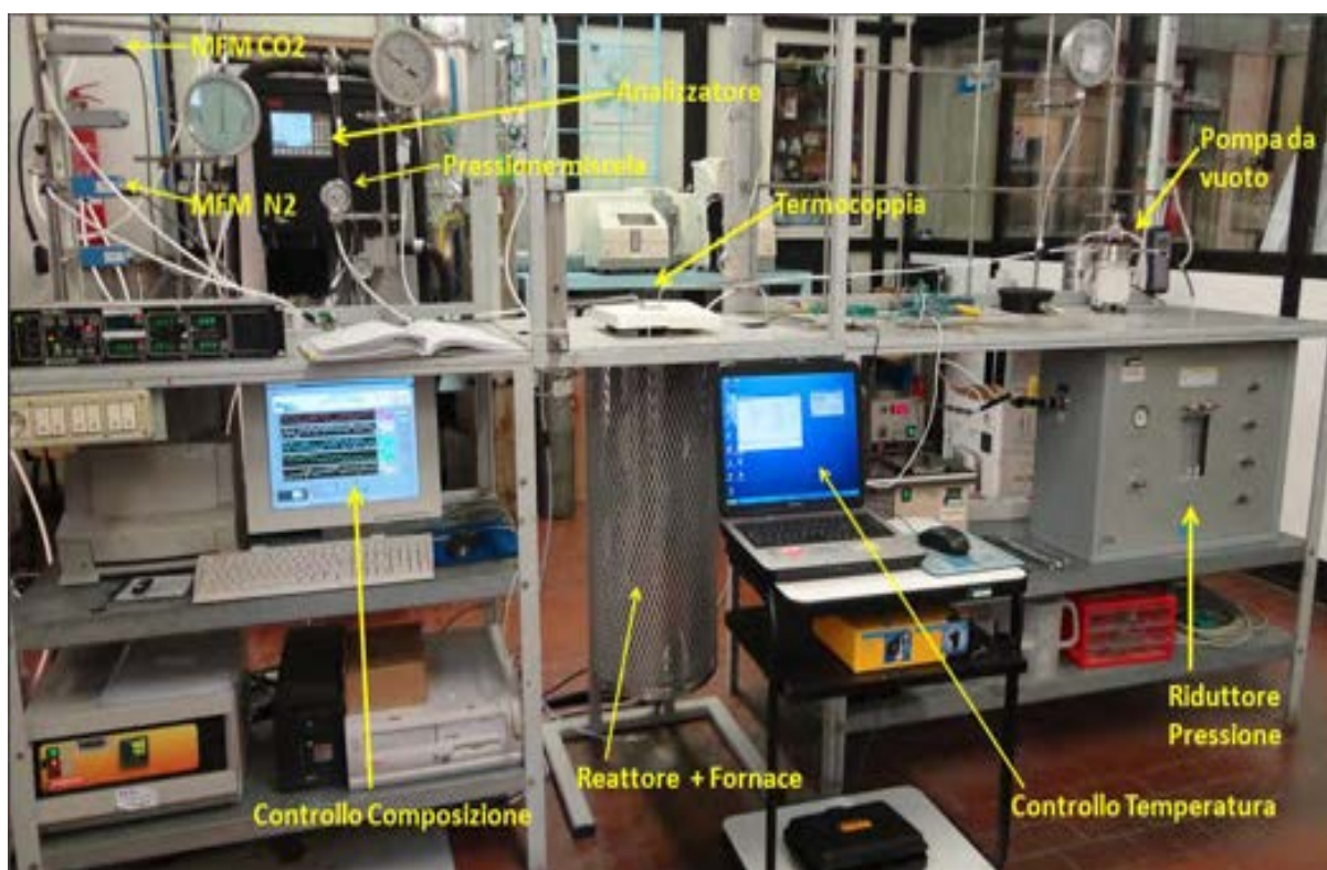
Fig.12: Impianto in scala di laboratorio per la cattura della CO 2 con micro-reattore
