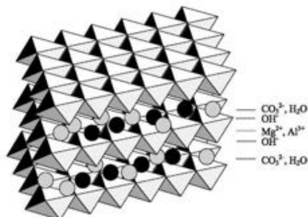
Fig. 2: Struttura dell'idrotalcite
