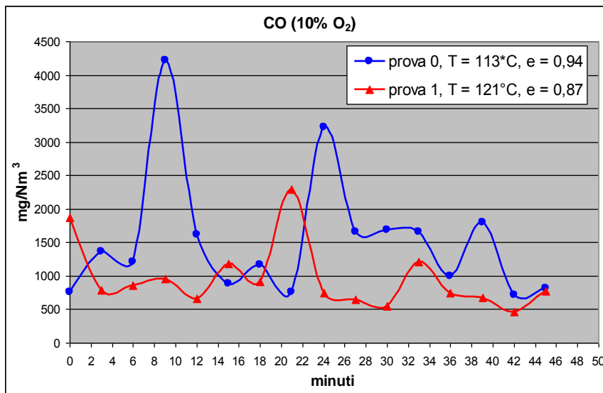
Figura 23: concentrazioni di CO a valle della linea di campionamento (T forno = 600 °C)
