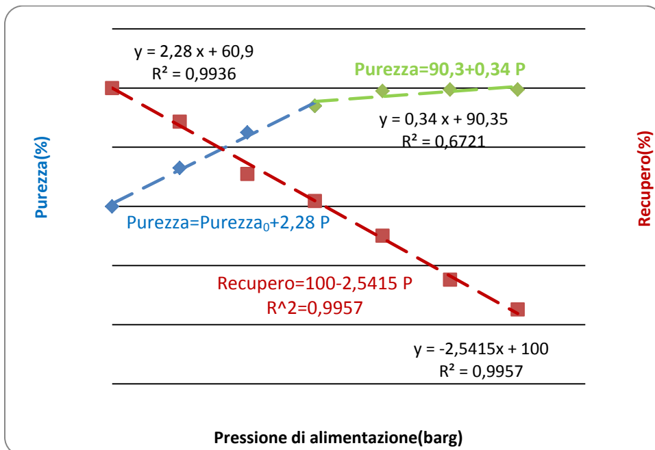
Figura 30 - Influenza della pressione di alimentazione sulla purezza e recupero del metano: Alimentazione al modulo 40kg/h
