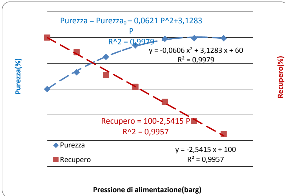
Figura 29 - Influenza della pressione di alimentazione sulla purezza e recupero del metano: Alimentazione al modulo 40 kg/h
