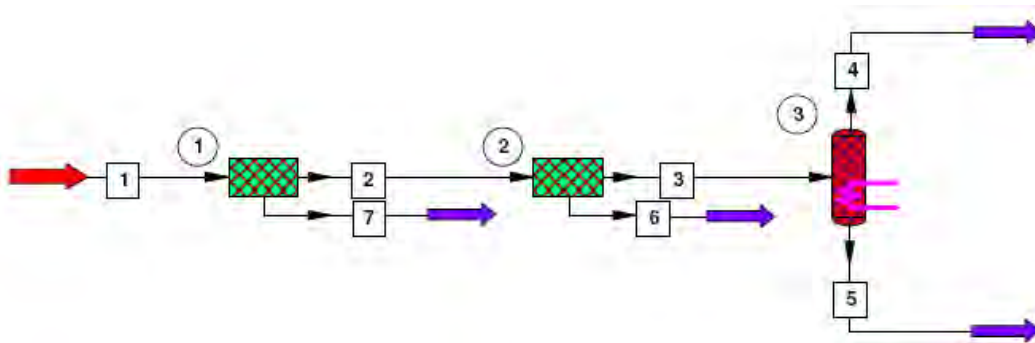
Figura 40 - Possibile configurazione impiantistica per gli impianti ibridi ammine/membrane[22]
