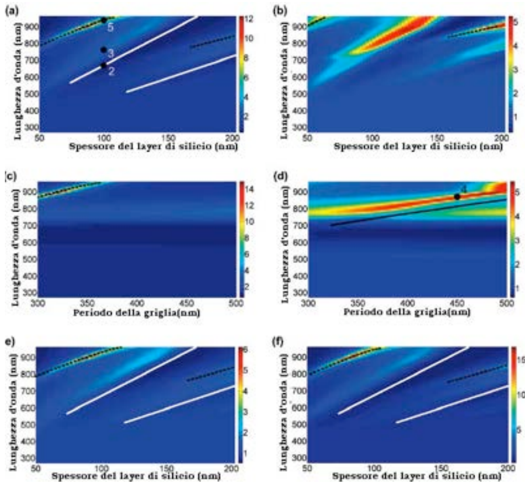
Figura 5 – Mappatura della funzione di enhancement in diversi casi: (a) polarizzazione TE con d_2=50\text{nm} (b) polarizzazione TM con d_2=50\text{nm} (c) polarizzazione TE con d_2=50\text{nm} (d) polarizzazione TM con d_2=50\text{nm} (e) polarizzazione TE con d_2=25\text{nm} (f) polarizzazione TE con d_2=100\text{nm} . In tutti i casi il periodo è P=300\text{nm}
