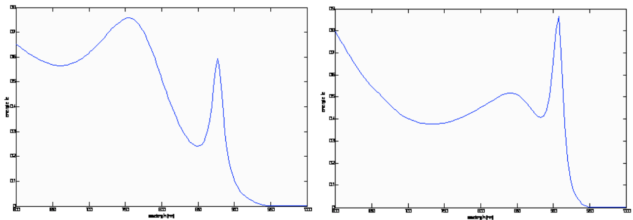
Figura 11 - Spettri di assorbimento per polarizzazioni TE nel caso in cui d_3=100\text{nm} e d_3=130\text{nm}
