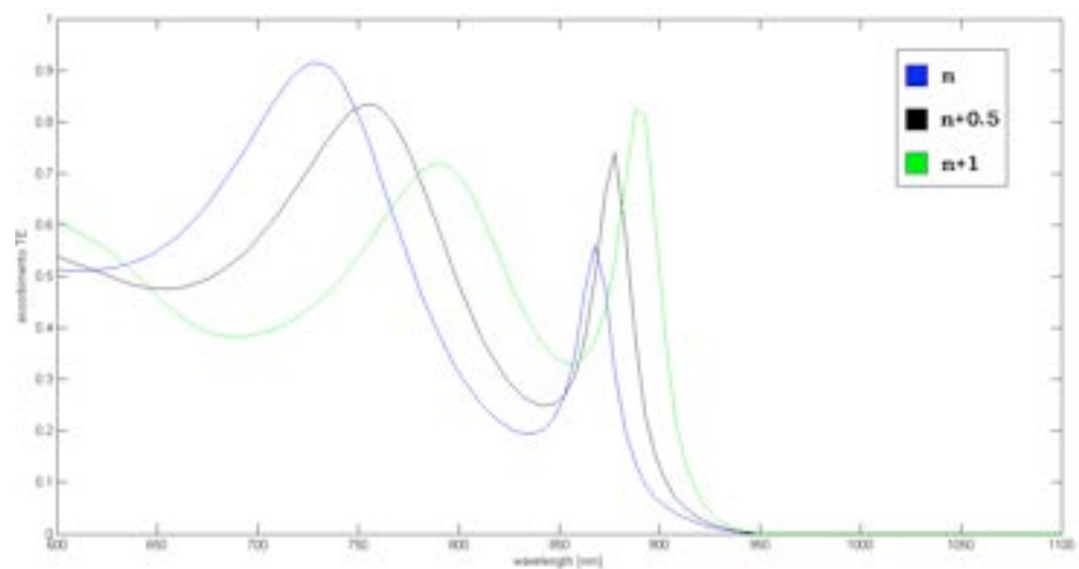
Figura 15 - Spettro di assorbimento per polarizzazioni TE in seguito a shift dell'indice di rifrazione dello ZnO
