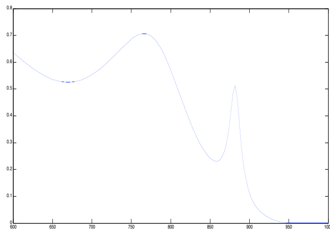
Figura 18 - Spettro di assorbimento per polarizzazione TE quando d_3=10\text{nm}
