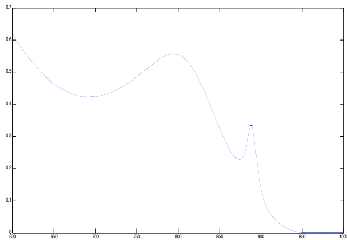
Figura 19- Spettro di assorbimento per polarizzazione TE quando d_3=50\text{nm}
