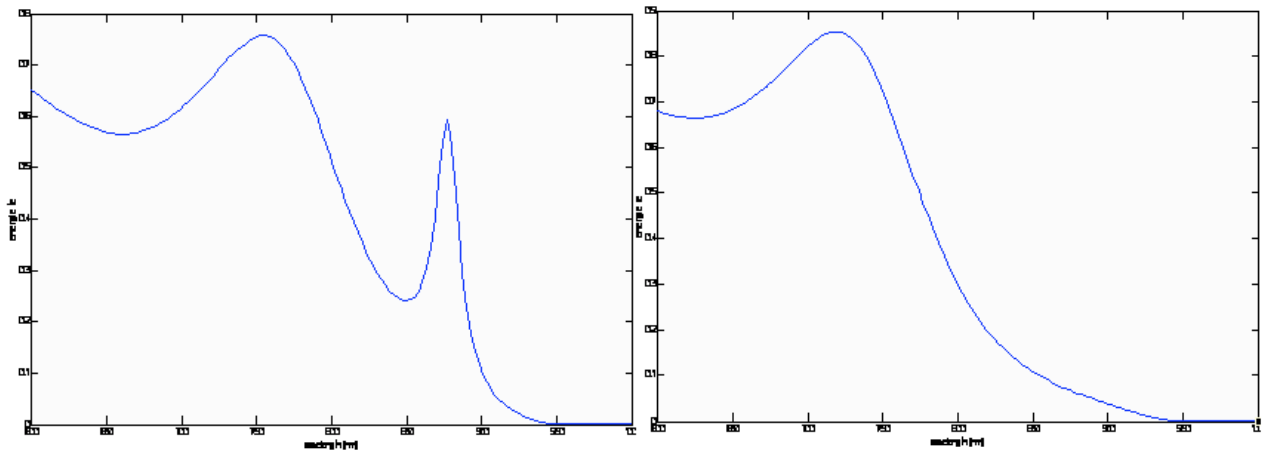
Figura 9 - Spettri di assorbimento per polarizzazioni TE nel caso in cui la struttura presenta la nanogriglia e nel caso in cui alla nanogriglia è sostituita uno strato omogeneo con opportuno indice di rifrazione
