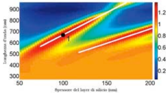
Figura 4 – rapporto tra l’assorbimento di una cella base composta da silicio e elettrodi di ITO con spessore d_3 = 100\text{nm} normalizzato rispetto ad un layer di silicio (spessore di 2-3 \mu\text{m} )
