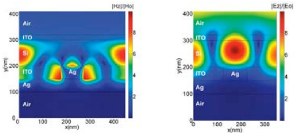
Figura 7 – Mappe del modulo del campo magnetico (nella cella unitaria) normalizzato riferite al punto 4 della figura (d) e quelle del modulo del campo elettrico normalizzato riferite al punto 5 della figura (a).
