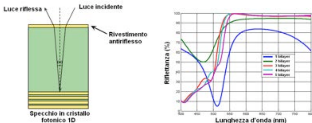
Figura 1 – (a) Schematizzazione di una cella solare a film sottile con back reflector a PC 1D; (b) Riflettanza del PC 1D in funzione del numero di strati.
