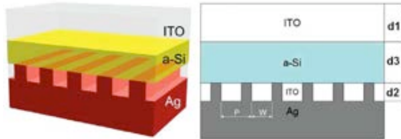
Figura 3 – schematizzazione di cella solare con back reflector ibrido metallo-dielettrico
