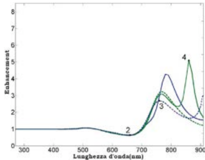
Figura 6 - Enhancement per polarizzazioni TM (linee continue) e TE (linee tratteggiate) per valori di periodo P=300\text{nm} (linee blu) e P=400\text{nm} (linee verdi)
