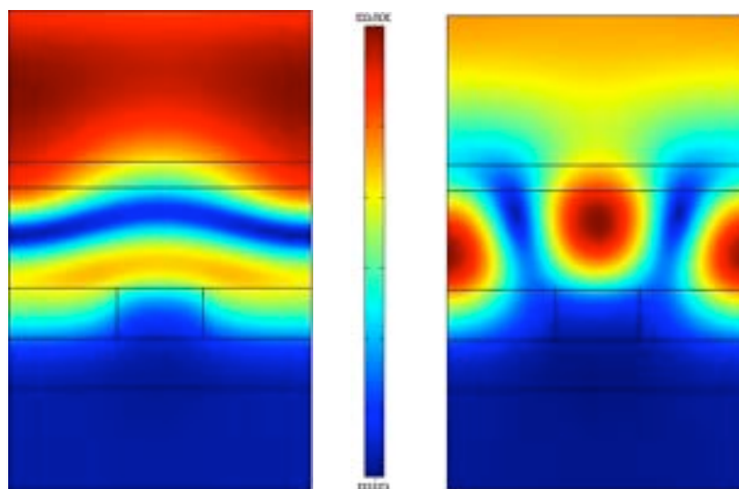
Figura 14 – Mappe del modulo campo elettrico dovuto a fenomeni di risonanza FP (sinistra) e a modi guidati (destra). Abbiamo successivamente ipotizzato una variazione dell'indice di rifrazione prima di 0.5 e in seguito di 1 per capire come questo cambiamento influenzasse gli spettri di assorbimento. La
