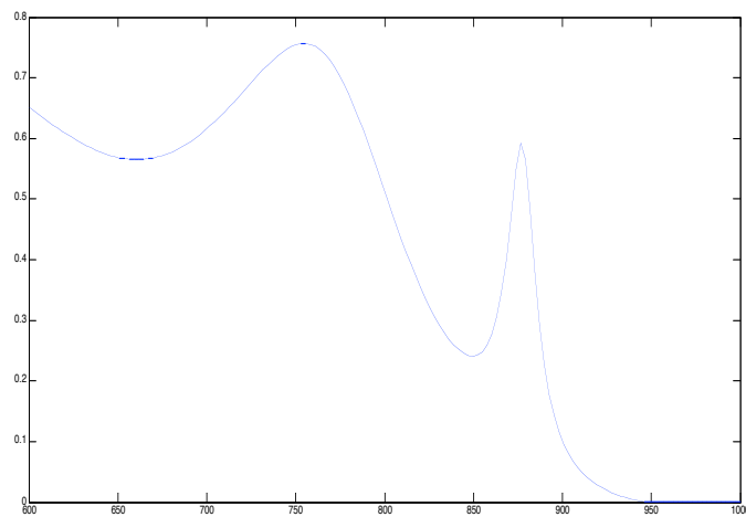
Figura 17- Spettro di assorbimento per polarizzazione TE quando d_3=0\text{nm}
