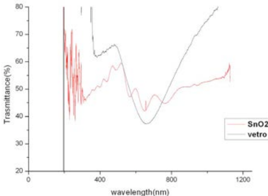
Fig.8 Evaporazione radente su vetro ed \text{SnO}_2 rugoso usato come supporto per una giunzione p-i-n da ENEA-TER
