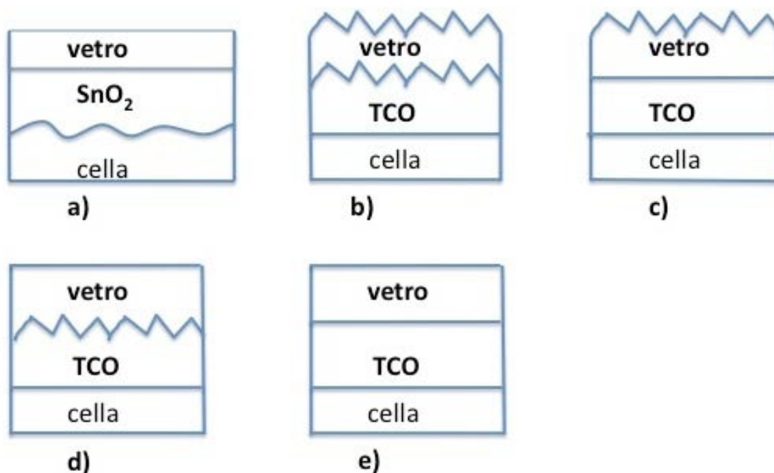
Fig.6 Schematizzazione dei dispositivi realizzati (disegni non in scala) da ENEA su: a) substrato commerciale di \text{SnO}_2 ; b)-d) substrati nanostrutturati a Genova; e) substrato vetro flat.
