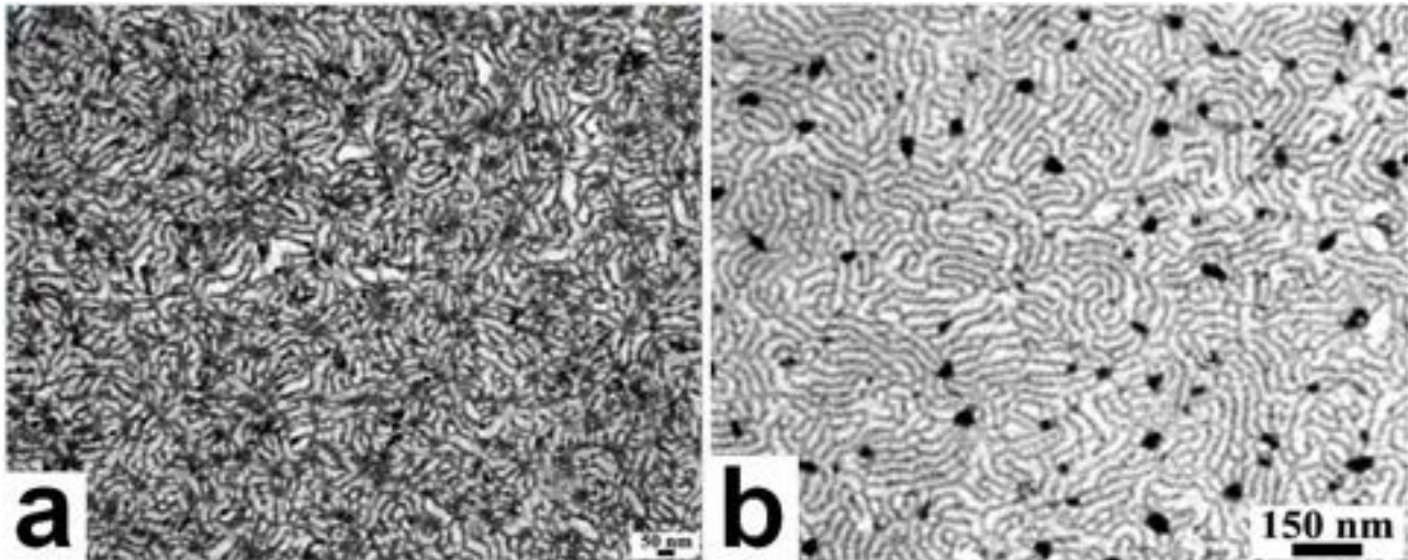
Figura 1. Immagini TEM bright-field di un film sottile (70 nm) di PS- b -PMMA depositato su substrato di ITO mediante spin-coating (3000 rpm, 30s) di una soluzione al 2% in peso in toluene (a) e di un film sottile di PS- b -PMMA depositato su substrato di ITO mediante drop-casting di una soluzione allo 0.5% in peso in toluene (b).
