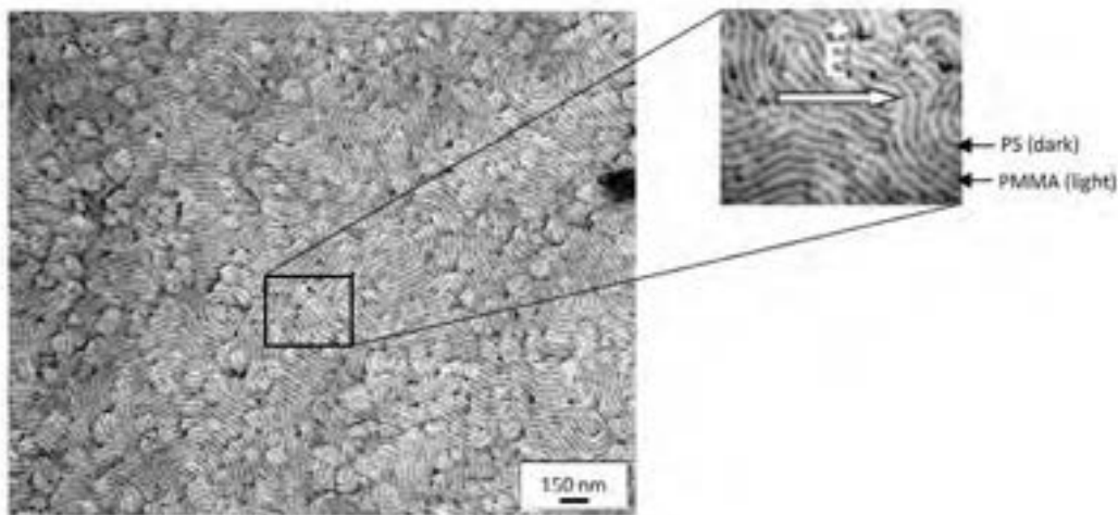
Figura 3. Immagine TEM di un film sottile di PS- b -PMMA ottenuto mediante spin-coating e sottoposto ad annealing termico sotto campo elettrico.
