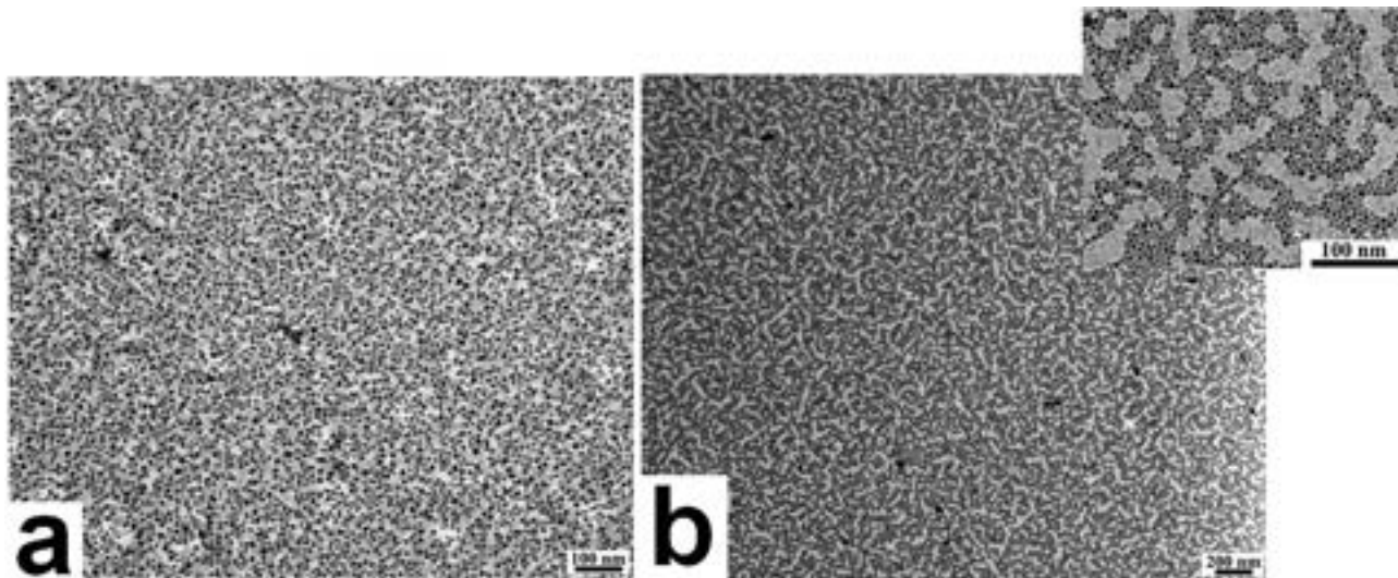
Figura 2. Immagini TEM di un film sottile di PS- b -PMMA depositato su substrato di ITO mediante spin-coating, trattato con RuO 4 , e decorato con nanoparticelle di oro (a), e dopo annealing a 150 °C per sei ore in vuoto (b). Viene mostrata l'immagine b ad elevato ingrandimento.
