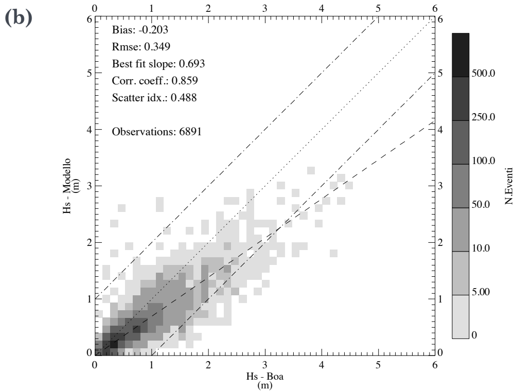
Figura 16: Scatter plot delle altezze significative (Hs) in metri della simulazione SIM_ECMWF (a) e del Centro Europeo ECMWF (b) rispetto ai dati relativi alla boa di Monopoli per il periodo 2001-2007.
