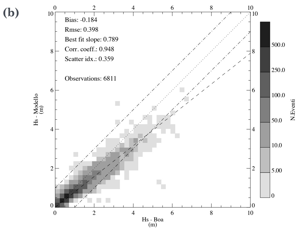
Figura 8: Scatter plot delle altezze significative (Hs) in metri della simulazione SIM_ECMWF (a) e del Centro Europeo ECMWF (b) rispetto ai dati relativi alla boa di Alghero per il periodo 2001-2007.
