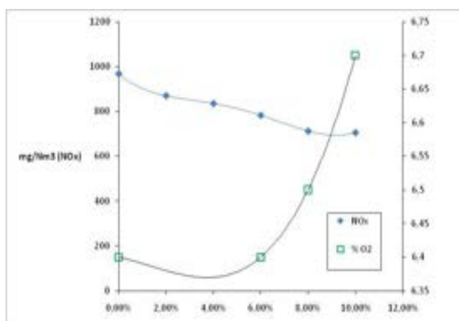
Fig. 21 – Emissioni di \text{NO}_x vs tenore di \text{O}_2 allo scarico in funzione della \%\text{H}_2
