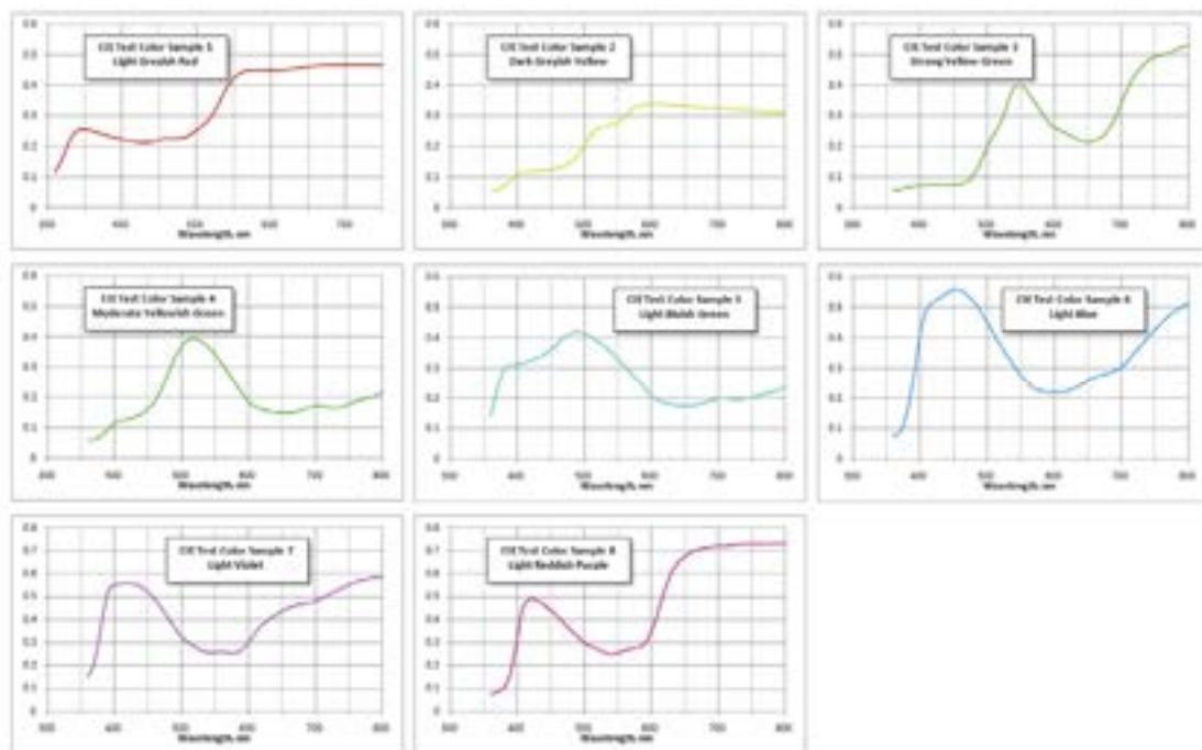
fig. 2 Coefficienti di riflessione spettrale dei campioni utilizzati nel CRI
