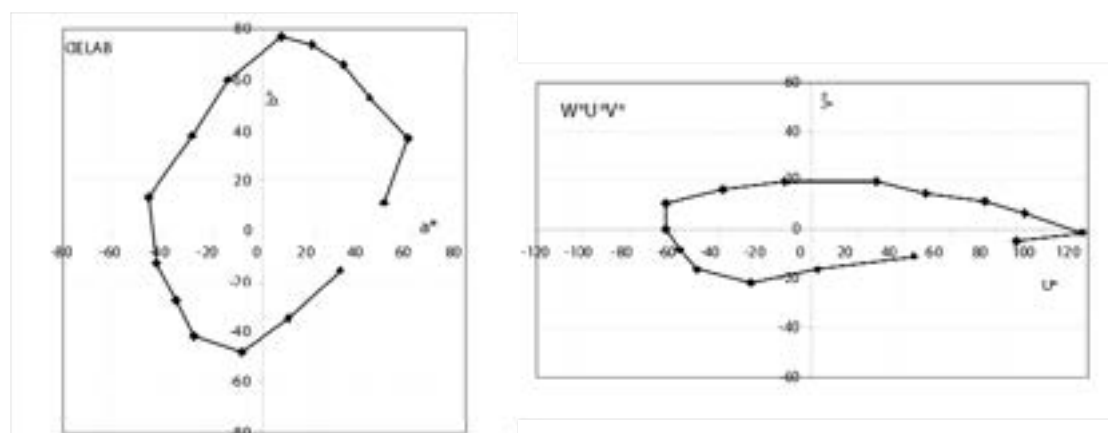
fig. 6 - I 15 nuovi campioni usati nel CQS nello spazio colore CIE 1976 L^*a^*b^* e CIE 1964 W^*U^*V^* .
