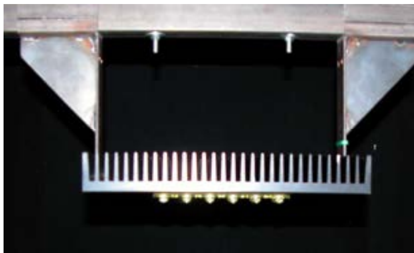
Figura 2 Dissipatore utilizzato per la misura dei moduli LED
