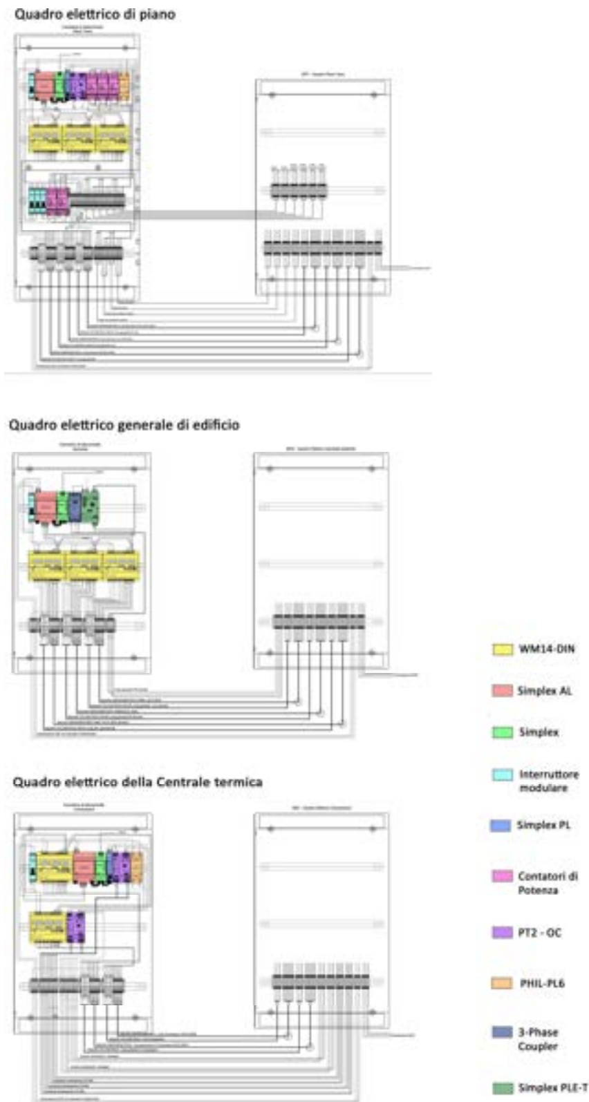
Figura 14: schema centralina di telecontrollo installata accanto ai quadri elettrici esistenti, con evidenza degli elementi installati.
