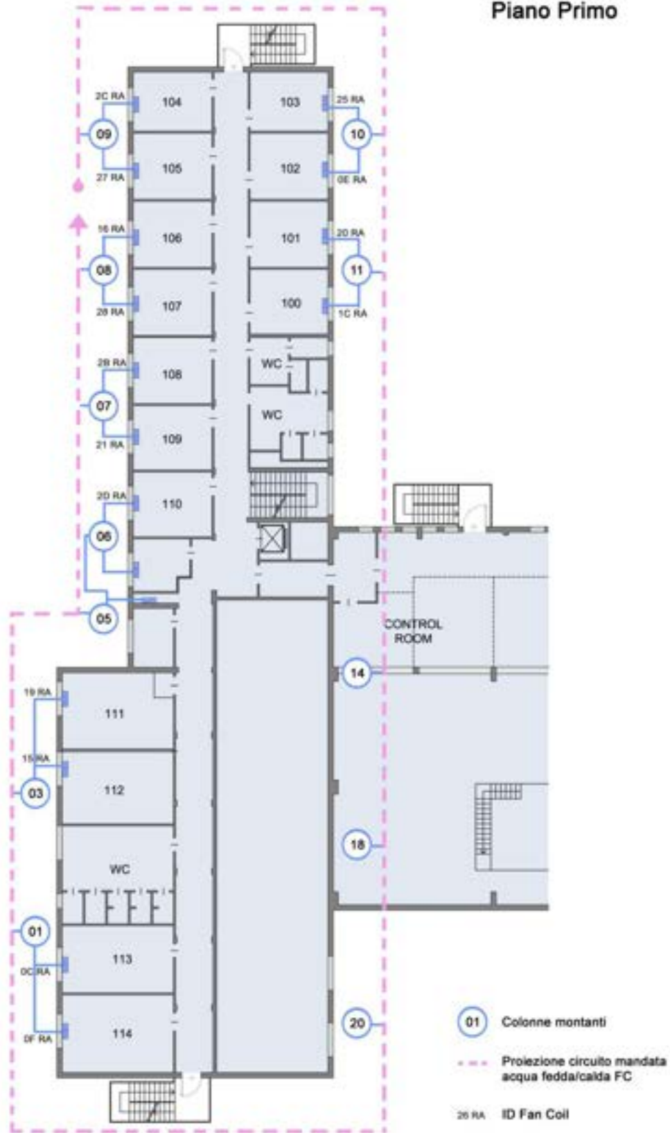
Figura A1.2: Circuito idronico a servizio dei fancoils: Piano Primo
