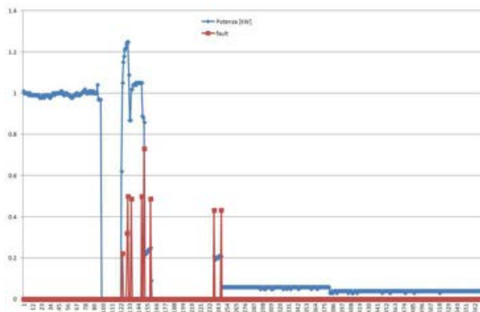
Figura 110 – Grado di allarme dell’indicatore in corrispondenza del fault.
