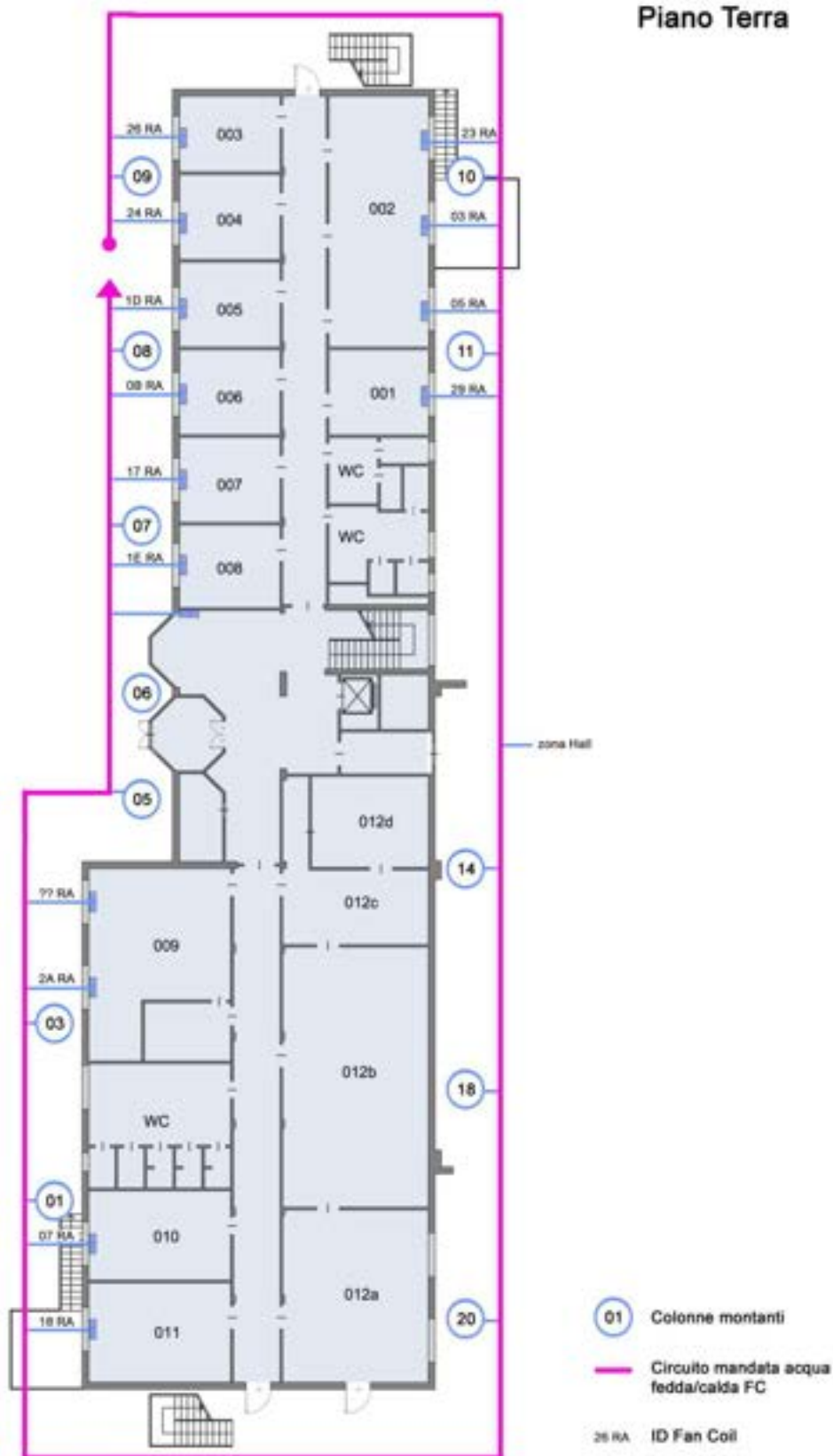
Figura A1.1: Circuito idronico a servizio dei fancoils: Piano terra
