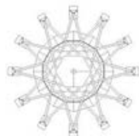
Sez D-D
