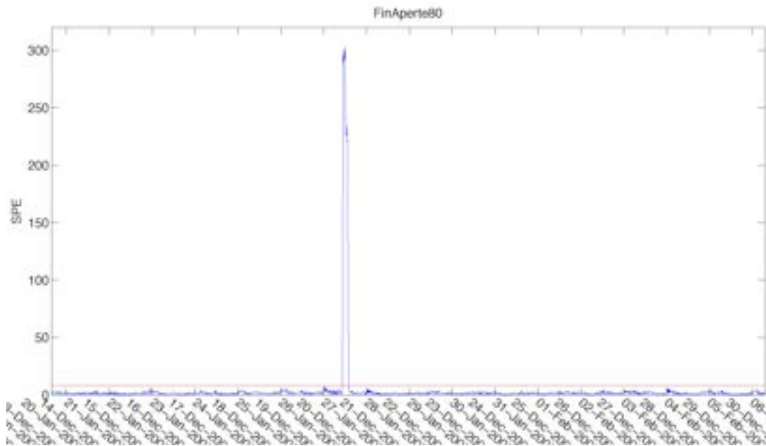
Apertura della finestra nella stanza 2 per 2 ore il 27 gennaio
