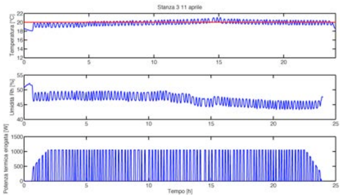
Parametri di una delle stanze non dotate di termostato
