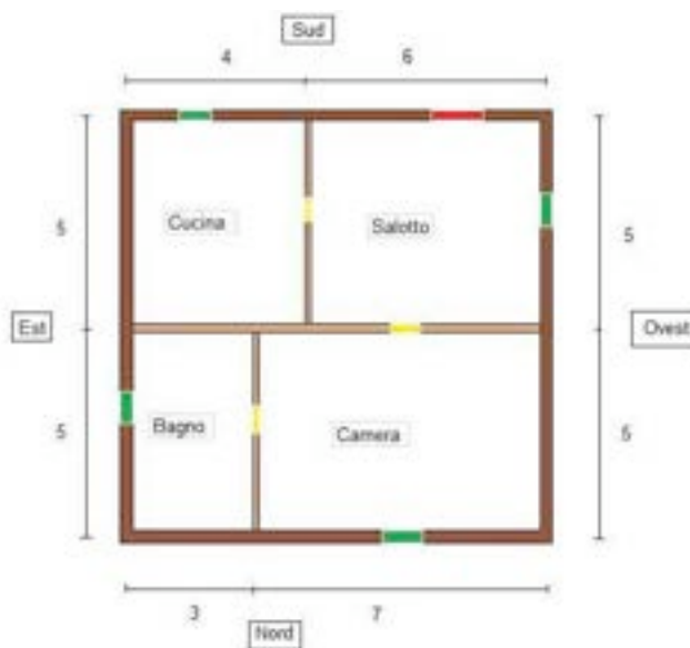
Figura - Realizzazione semplificata dell'edificio
