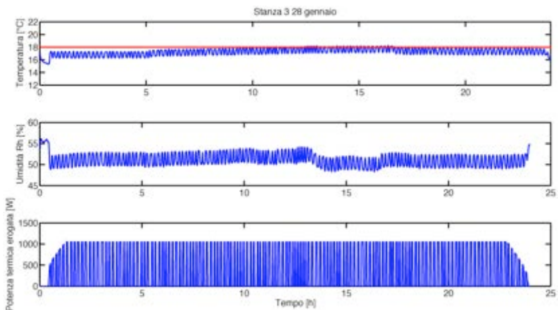
Parametri di una delle stanze non dotate di termostato
