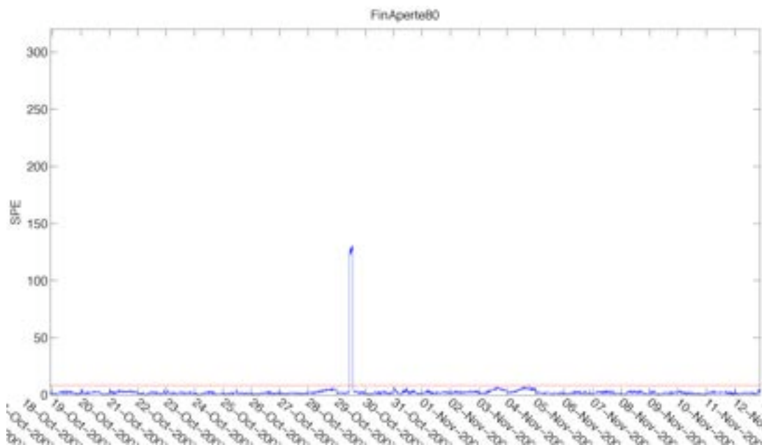
Apertura della finestra nella stanza 2 per 2 ore il 29 ottobre
