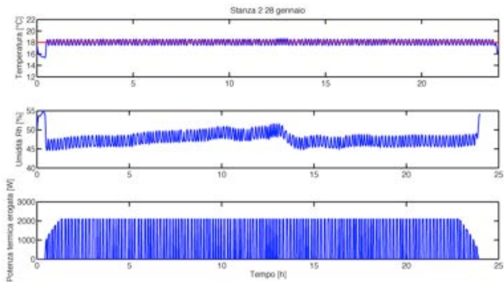
Parametri della stanza dotata di termostato (soggiorno)
