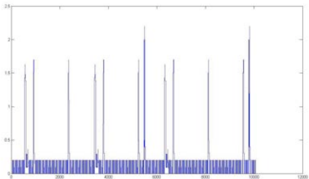
Curva di carico elettrico settimanale dell'unità abitativa
