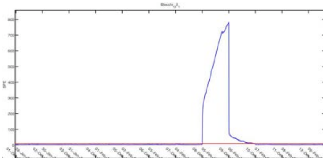
L'andamento dello SPE (l'indice di rilevazione del guasto) nel caso di blocco della valvola nella stanza 2
