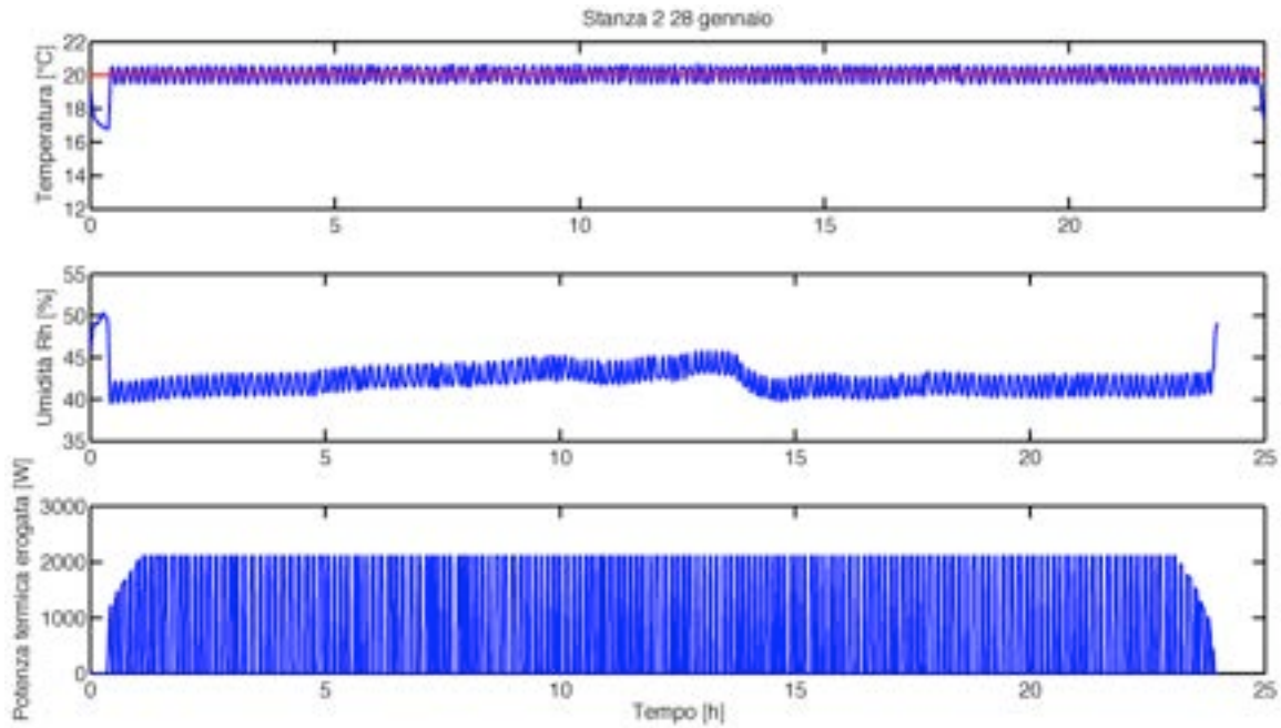
Parametri della stanza dotata di termostato (soggiorno)
