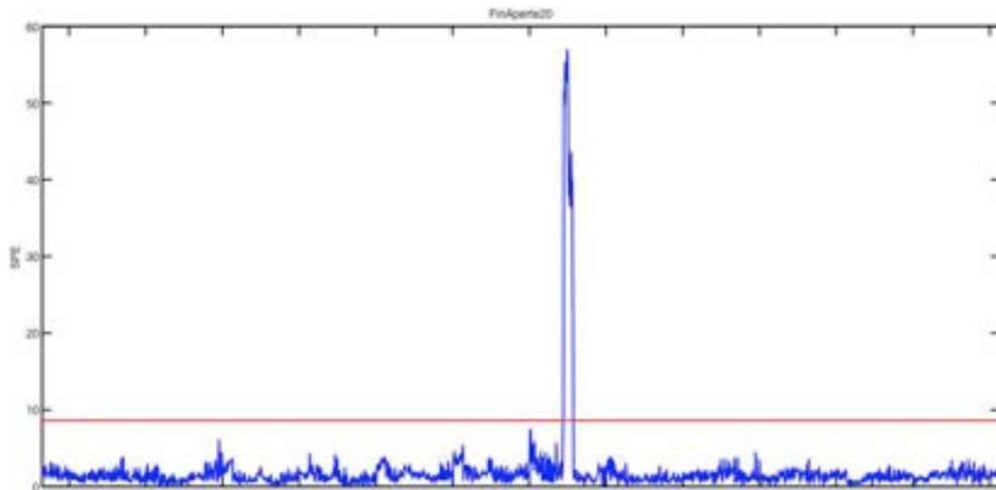
Apertura della finestra 2 del 20%.
