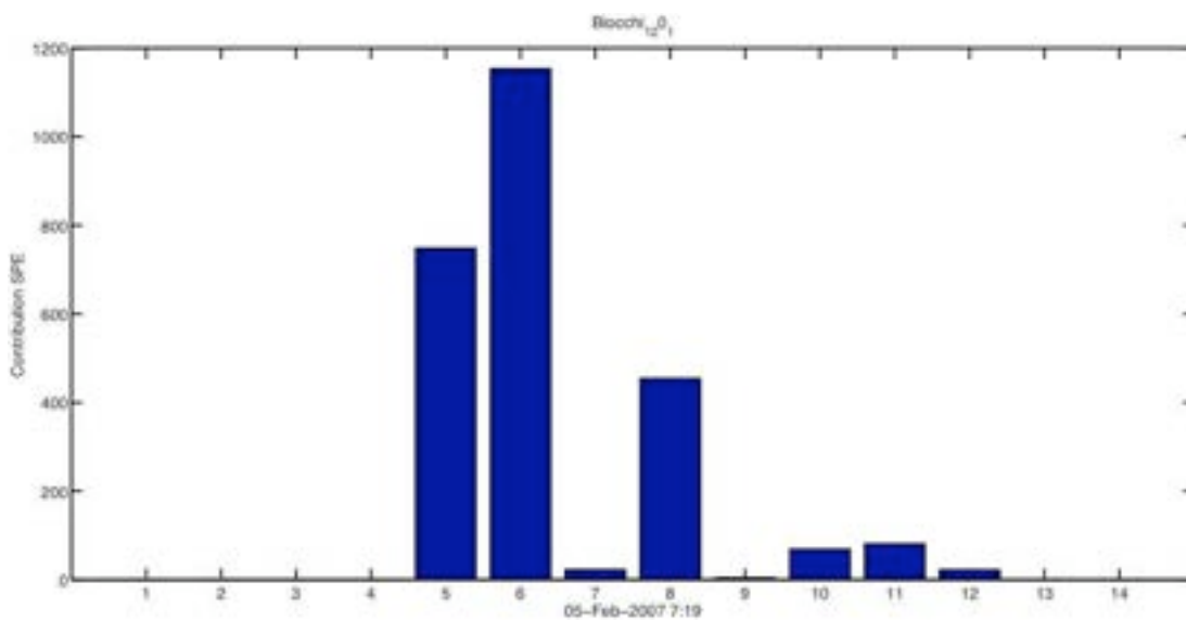
La firma del blocco valvola nella stanza 2.
