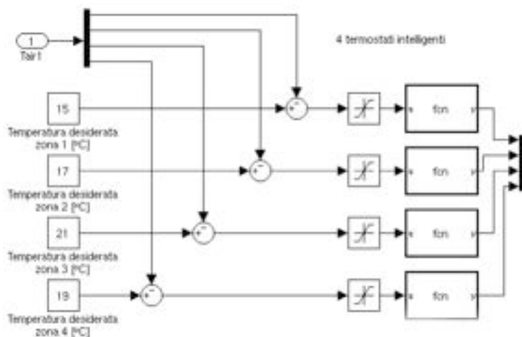
Blocchi Simulink dei termostati
