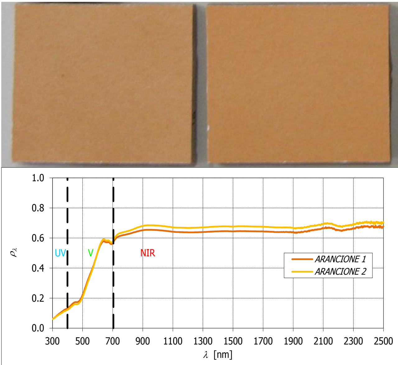
Figura 25. Fotografie e riflettività spettrali di cool color ceramici. Arancione 1 R=51%; Arancione 2 R=54%
