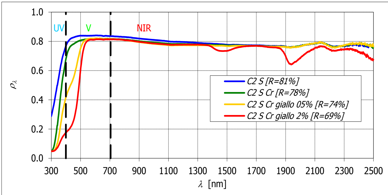
Figura 26. Riflettività spettrali e riflettanze solari dei cool colors gialli
