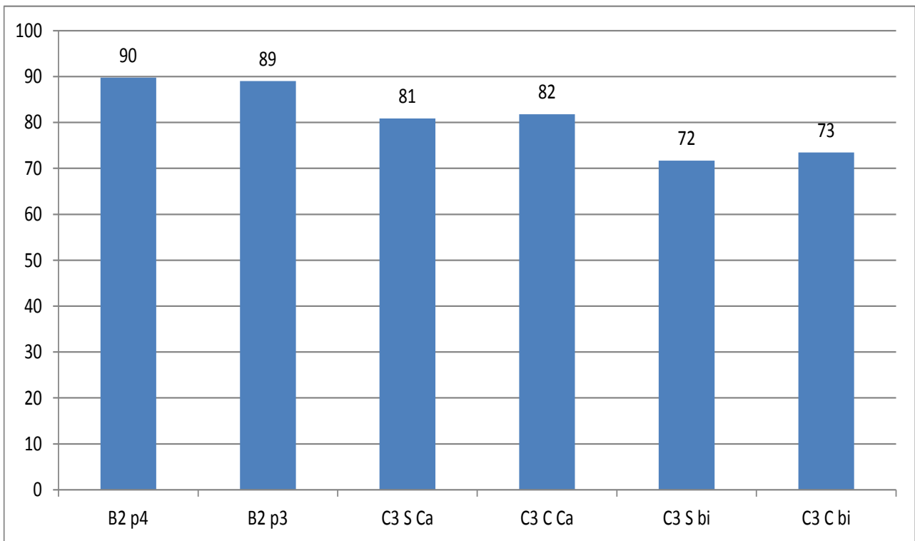
Figura 19. Riflettanza solare campioni Serie 4
