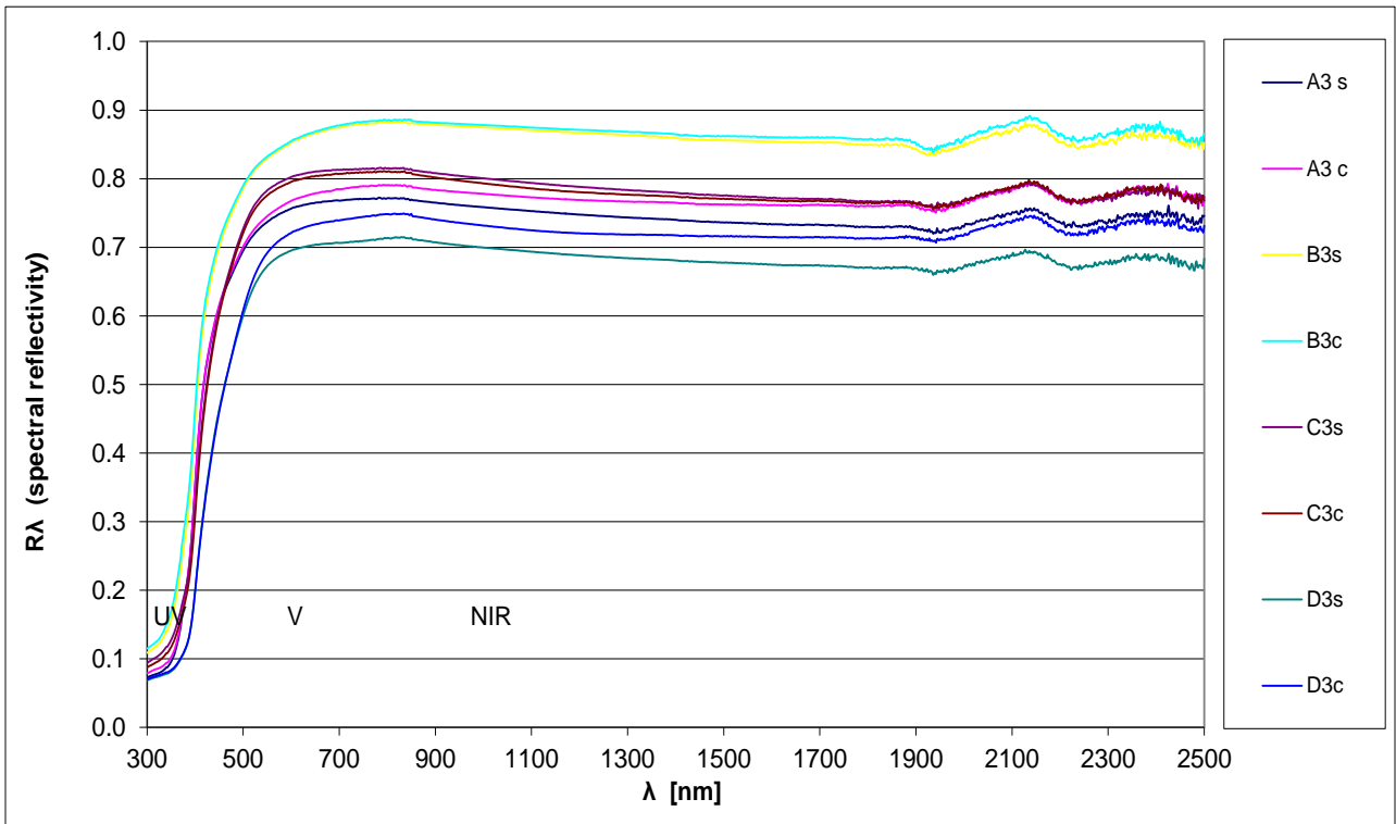
Figura 16. Riflettività spettrale campioni Serie 3
