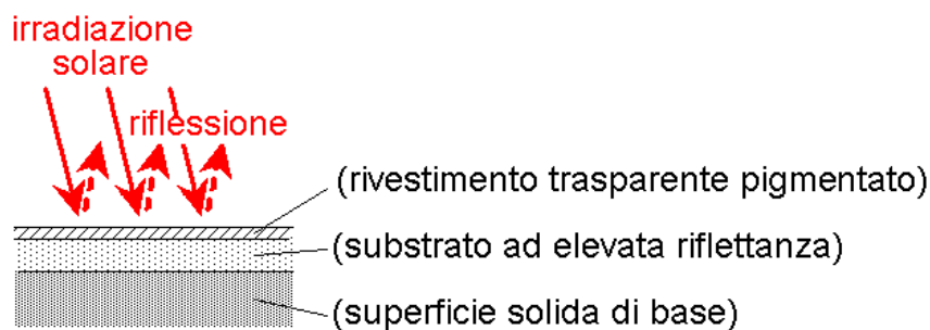
Figura 8. Schema stratigrafico di un rivestimento tipo cool color
