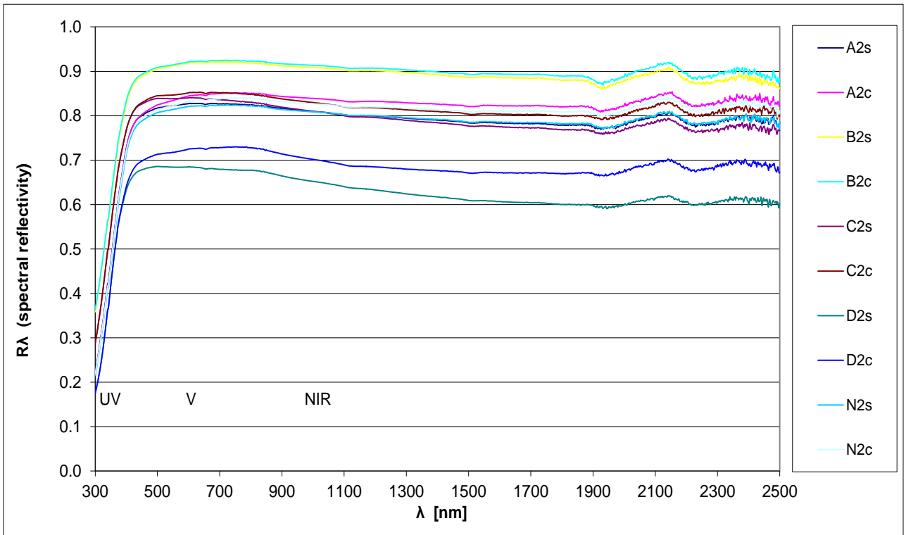
Figura 14. Riflettività spettrale campioni Serie 2
