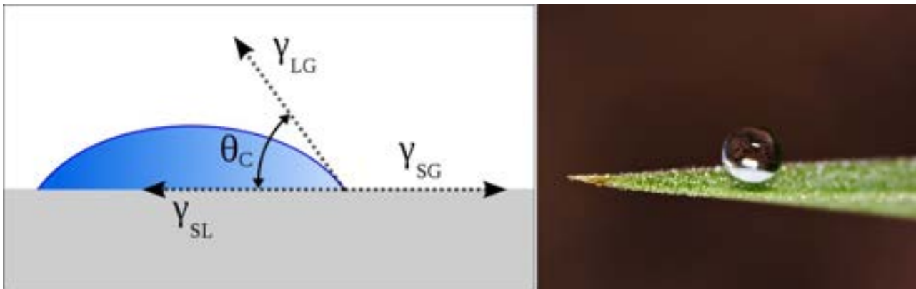
Figura 23. Angolo di contatto e superidrofobicità
