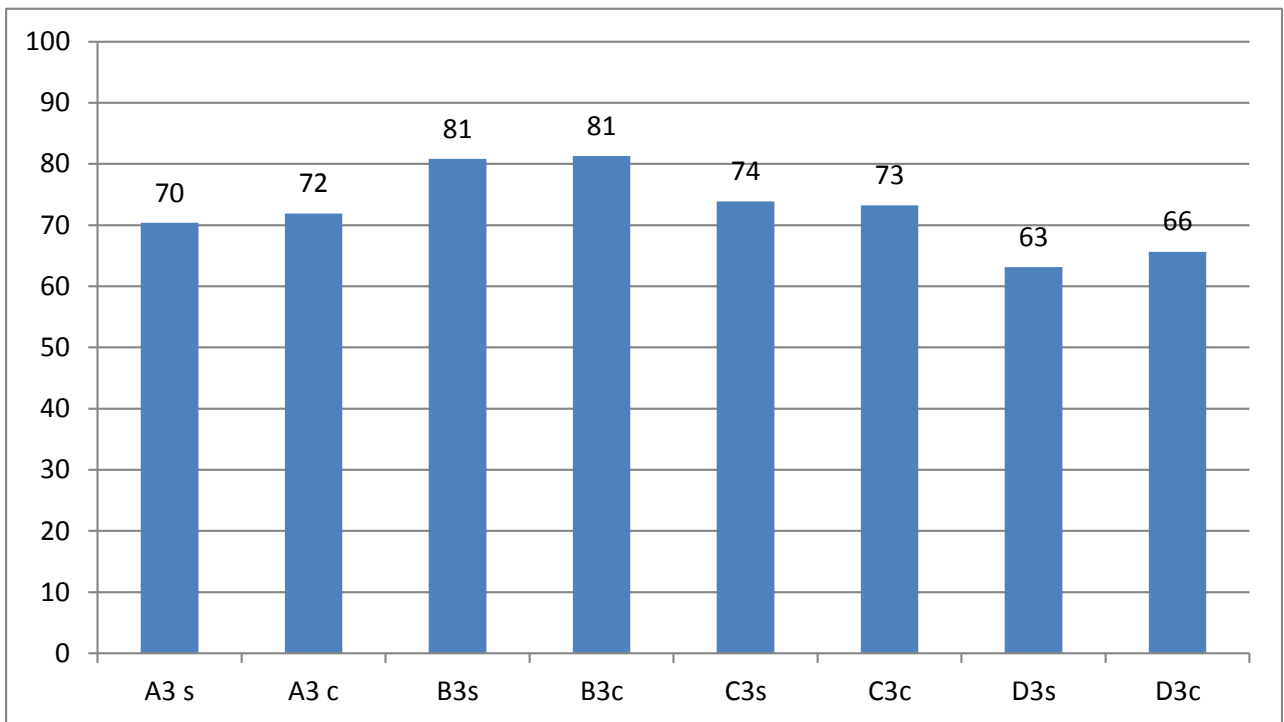
Figura 17. Riflettanza solare campioni Serie 3
