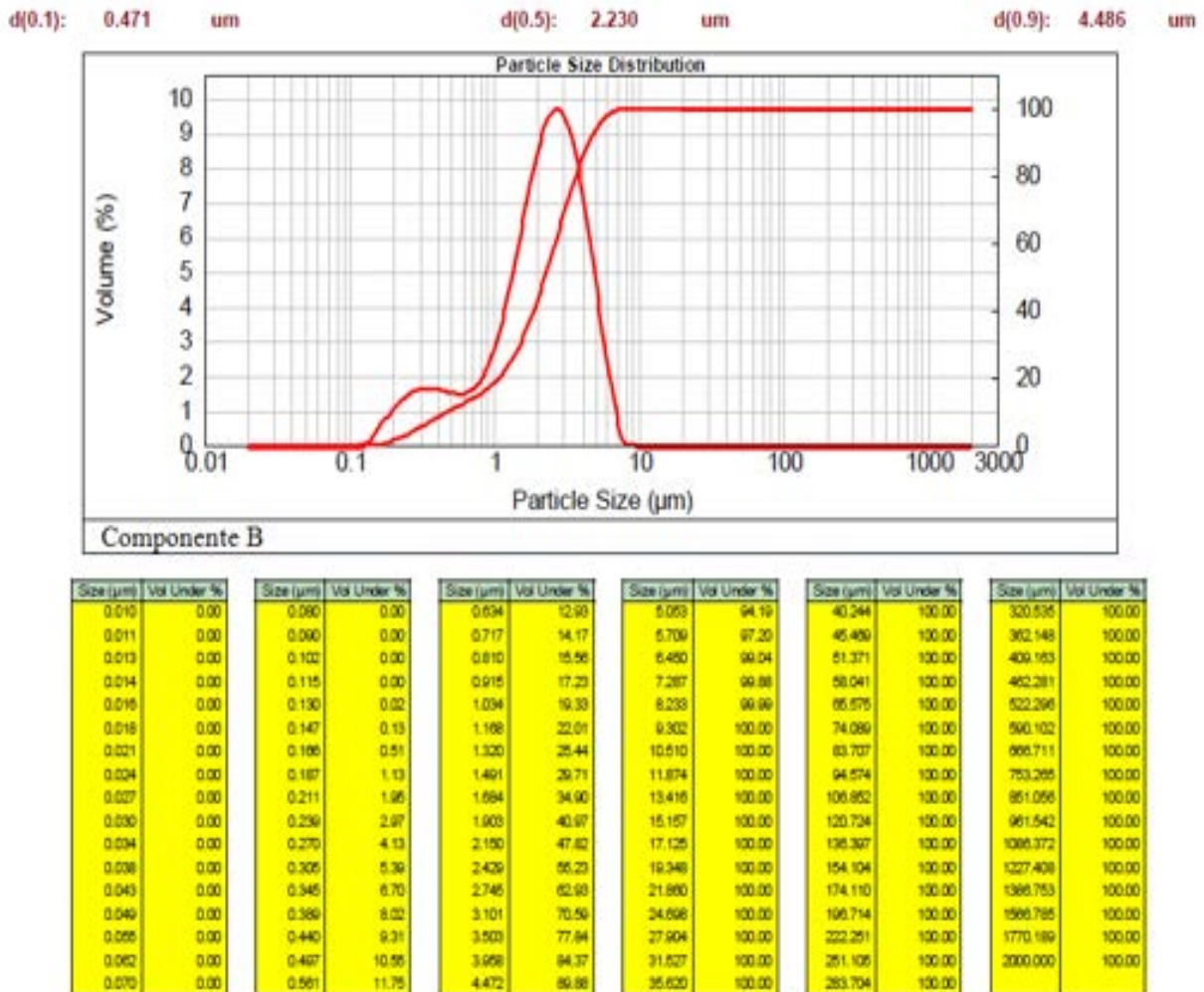
Figura 10. Risultati delle misure granulometriche sul Componente B
