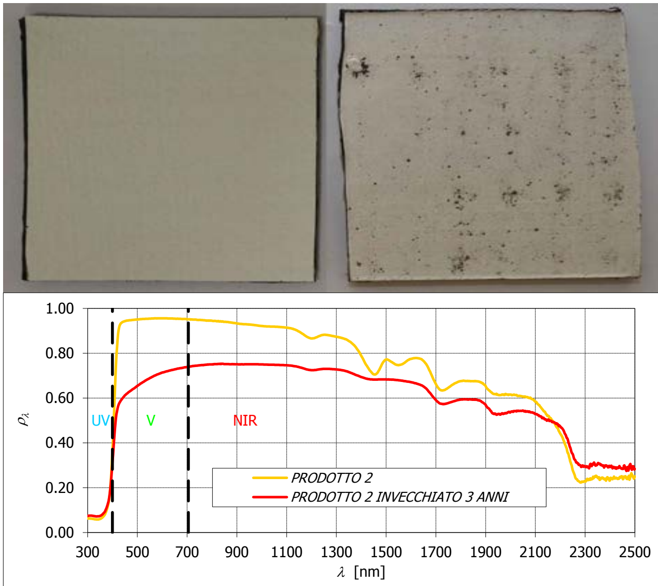
Figura 5. Vernice commerciale 2 per cool roof acrilica a nuovo (R=86%), esposta 3 anni (R=66%)
