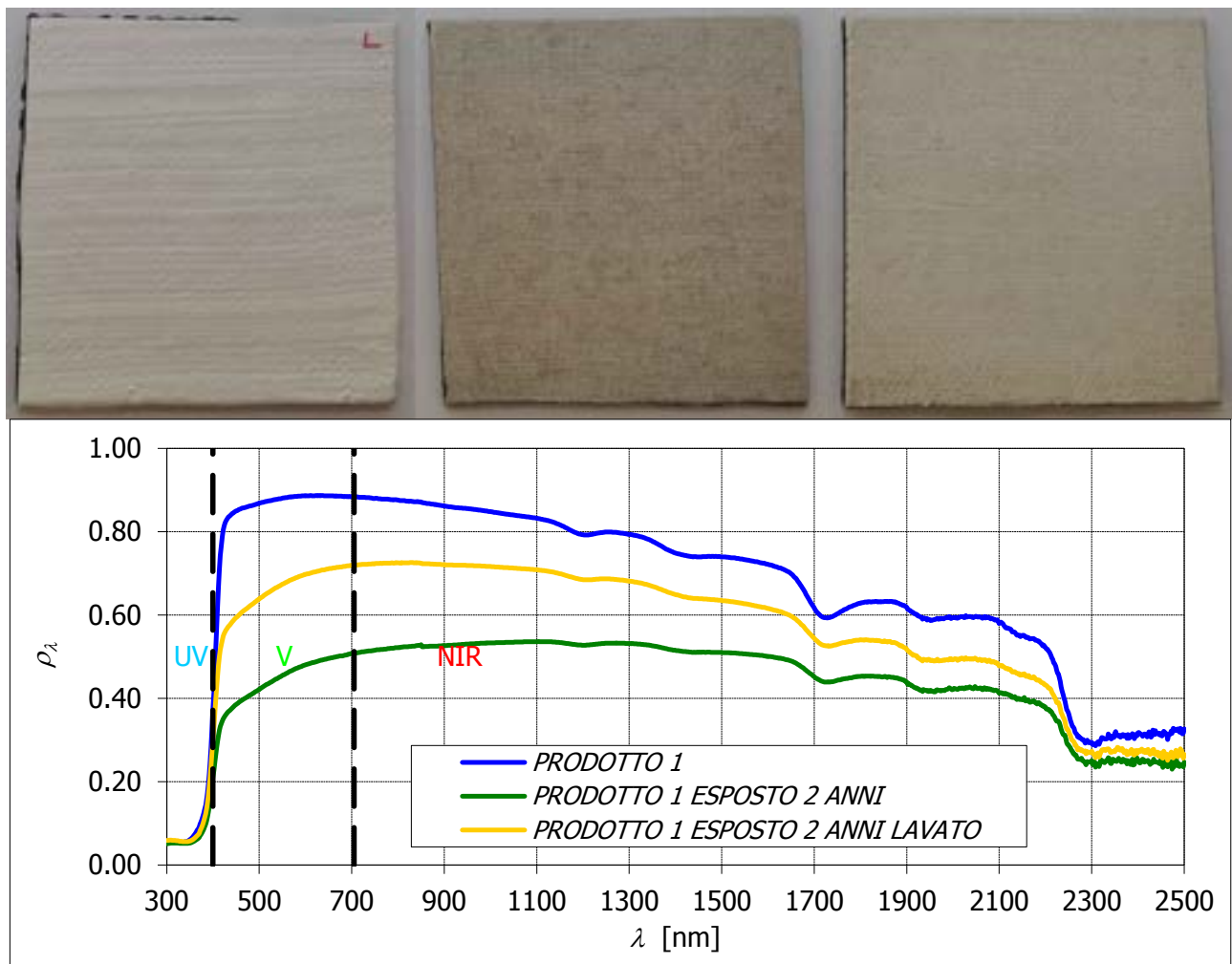
Figura 4. Vernice commerciale 1 per cool roof acrilica a nuovo (R=80%), esposta 2 anni (R=46%) ed esposta 2 anni e lavata con acqua (R=64%)
