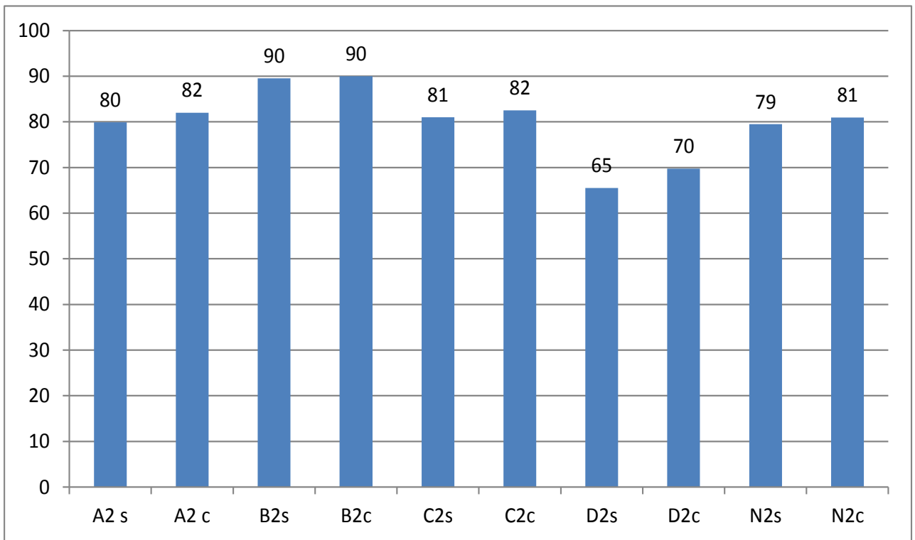
Figura 15. Riflettanza solare campioni Serie 3
