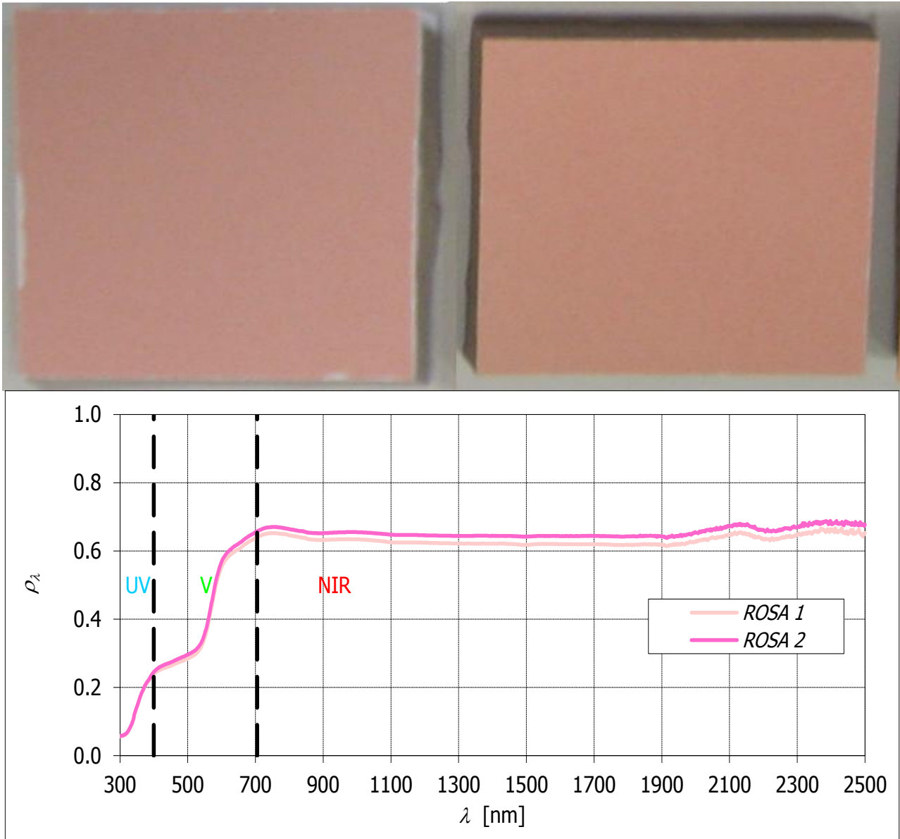
Figura 24. Fotografie e riflettività spettrali di cool color ceramici. Rosa 1 R=49%; rosa 2 R=51%
