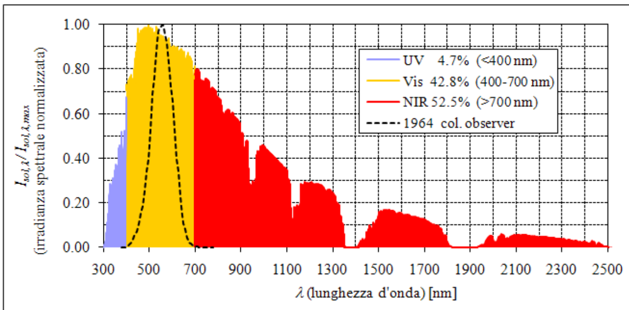
Figura 7. Spettro normalizzato della radiazione solare sulla superficie terrestre
