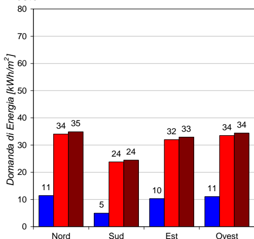
AGENZIA - Fabbisogno di Riscaldamento Trieste
