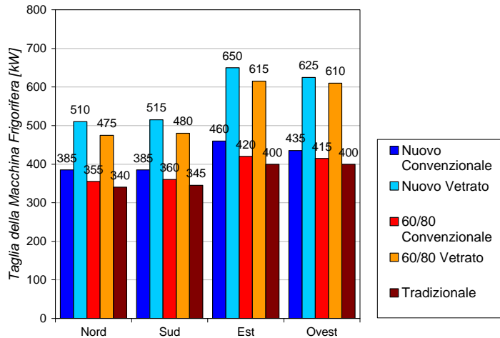
FILIALE - Taglia della Macchina Frigorifera Bolzano
