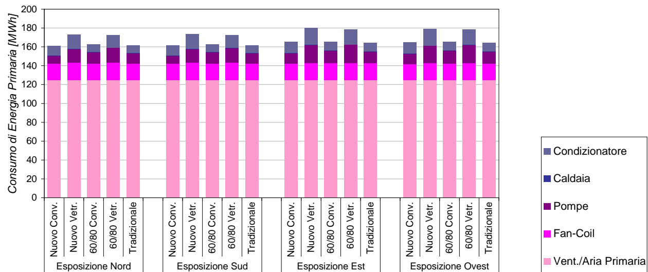
Figura 45. Composizione del consumo di energia primaria relativo agli ausiliari d’impianto per l’edificio ad uso filiale nella città di Milano.
