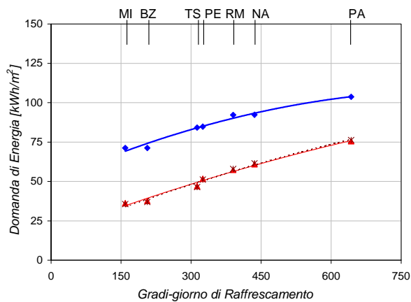
AGENZIA - Fabbisogno di Raffrescamento Esposizione Est
