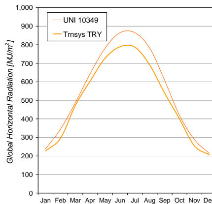
Figura 8. Valori medi mensili di temperatura dell'aria e di radiazione solare globale sull'orizzontale secondo norma UNI 10349 e derivati dal TRY fornito con TRNSYS. Città di Palermo.
