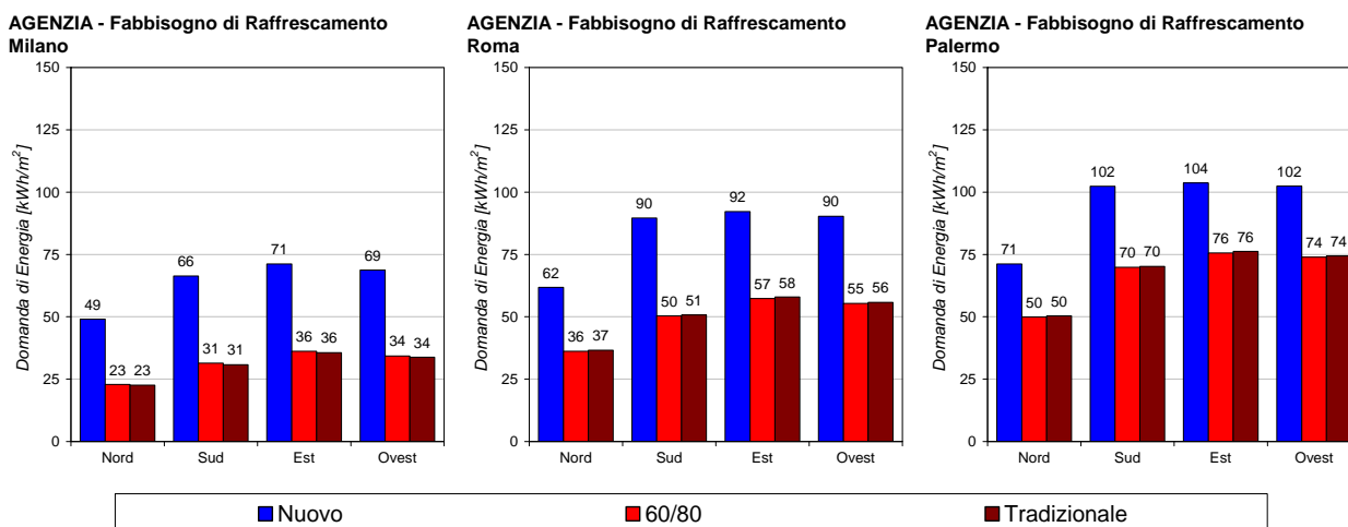
Figura 23. Fabbisogno di raffrescamento specifico relativo al piano agenzia nelle città di Milano, Roma e Palermo.
