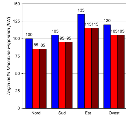
AGENZIA - Taglia della Macchina Frigorifera Palermo
