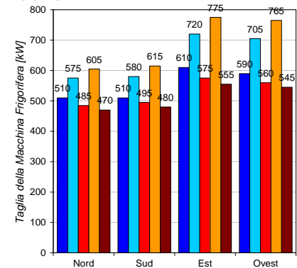
FILIALE - Taglia della Macchina Frigorifera Palermo
