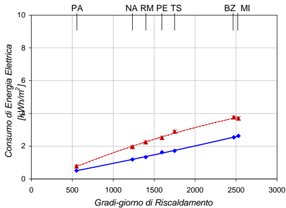
AGENZIA - Energia Elettrica per Riscaldamento Esposizione Est
