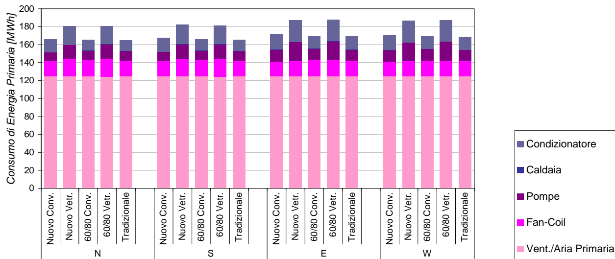
Figura 47. Composizione del consumo di energia primaria relativo agli ausiliari d’impianto per l’edificio ad uso filiale nella città di Roma.
