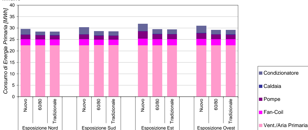
Figura 39. Composizione del consumo di energia primaria relativo agli ausiliari d'impianto per il piano agenzia nella città di Milano.
