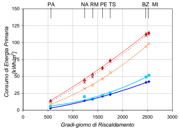
UFFICI - Energia Primaria per Riscaldamento Esposizione Est-Ovest
