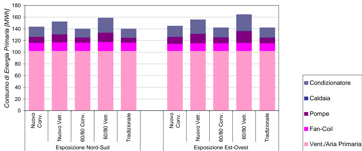
Figura 37. Composizione del consumo di energia primaria relativo agli ausiliari d'impianto per i piani adibiti ad uffici nella città di Palermo.
