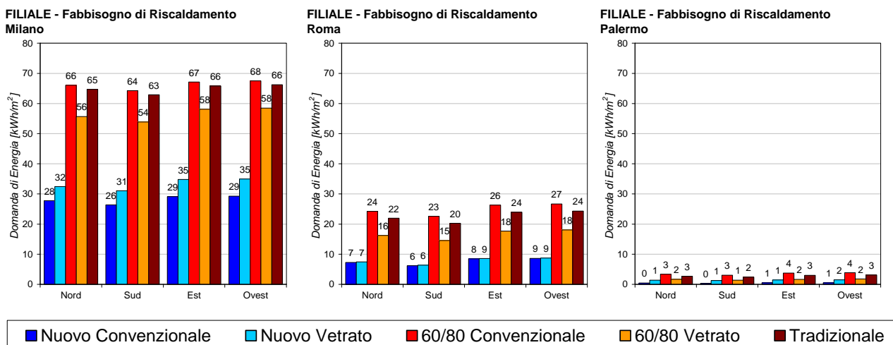
Figura 24. Fabbisogno di riscaldamento specifico relativo all’edificio ad uso filiale nelle città di Milano, Roma e Palermo.
