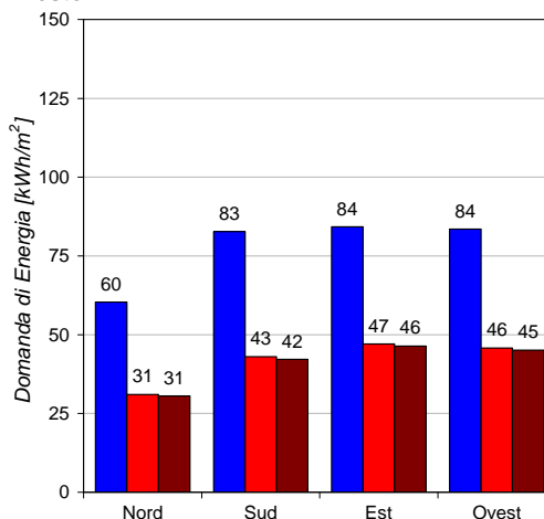
AGENZIA - Fabbisogno di Raffrescamento Trieste
