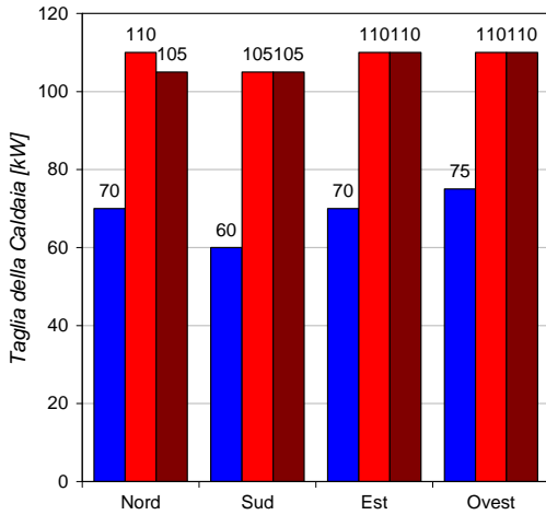
AGENZIA - Taglia della Caldaia Bolzano
