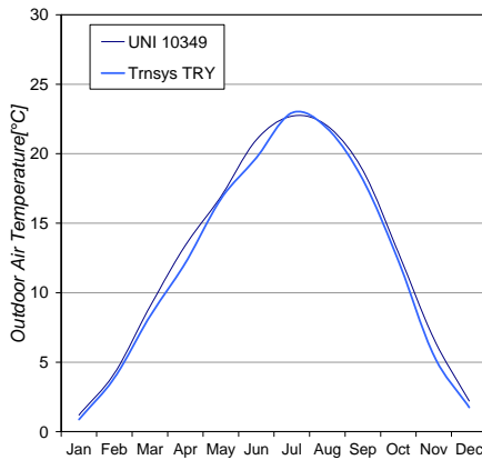
Figura 3. Valori medi mensili di temperatura dell'aria e di radiazione solare globale sull'orizzontale secondo norma UNI 10349 e derivati dal TRY fornito con TRNSYS. Città di Bolzano.
