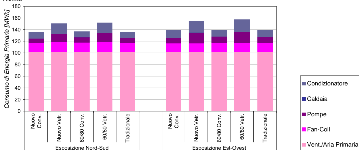
Figura 35. Composizione del consumo di energia primaria relativo agli ausiliari d’impianto per i piani adibiti ad uffici nella città di Roma.
