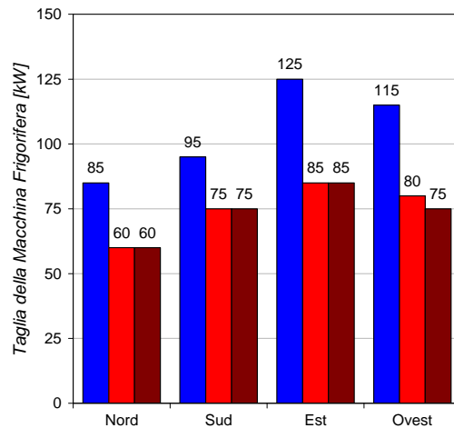
AGENZIA - Taglia della Macchina Frigorifera Trieste
