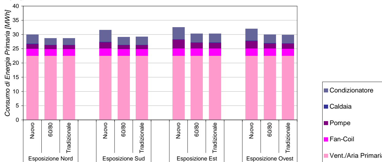
Figura 41. Composizione del consumo di energia primaria relativo agli ausiliari d'impianto per il piano agenzia nella città di Roma.
