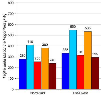
UFFICI - Taglia della Macchina Frigorifera Milano
