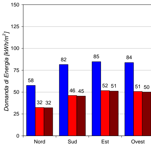
AGENZIA - Fabbisogno di Raffrescamento Pescara
