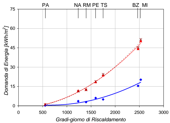
AGENZIA - Fabbisogno di Riscaldamento Esposizione Ovest
