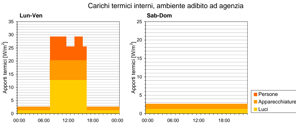
Figura 17: Profili orari dei carichi termici interni complessivi dell'agenzia.
