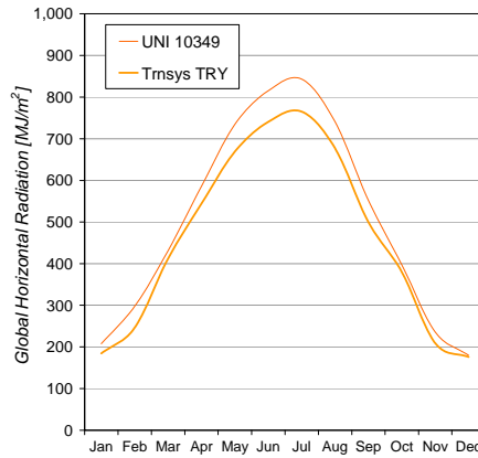
Figura 7. Valori medi mensili di temperatura dell'aria e di radiazione solare globale sull'orizzontale secondo norma UNI 10349 e derivati dal TRY fornito con TRNSYS. Città di Napoli.
