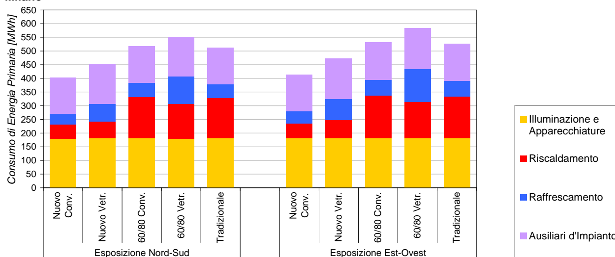
Figura 32. Composizione del consumo di energia primaria per i piani adibiti ad uffici nella città di Milano.
