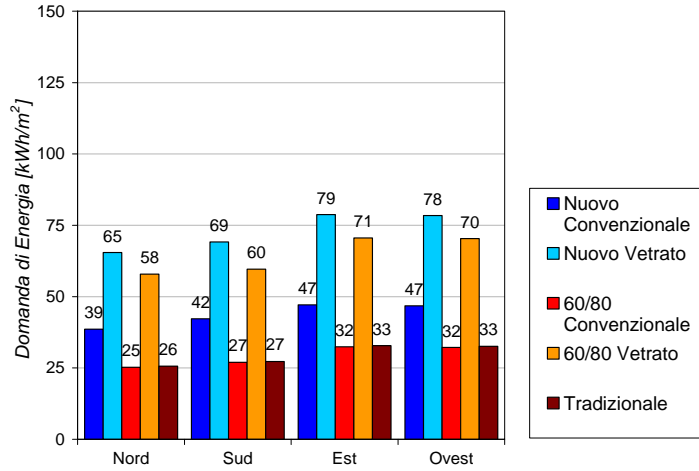
FILIALE - Fabbisogno di Raffrescamento Bolzano
