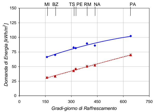
AGENZIA - Fabbisogno di Raffrescamento Esposizione Ovest
