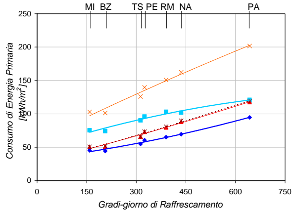
UFFICI - Energia Primaria per Raffrescamento Esposizione Est-Ovest
