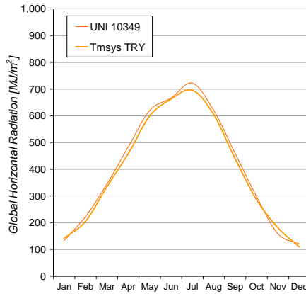
Figura 4. Valori medi mensili di temperatura dell'aria e di radiazione solare globale sull'orizzontale secondo norma UNI 10349 e derivati dal TRY fornito con TRNSYS. Città di Trieste.
