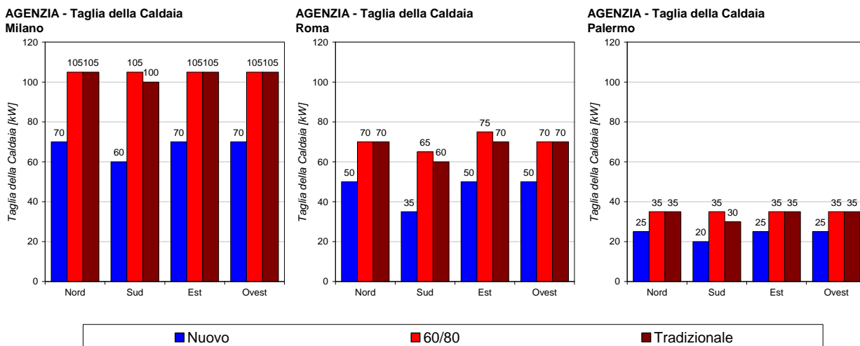
Figura 27. Taglia della caldaia per il piano agenzia nelle città di Milano, Roma e Palermo.
