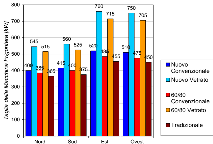
FILIALE - Taglia della Macchina Frigorifera Trieste
