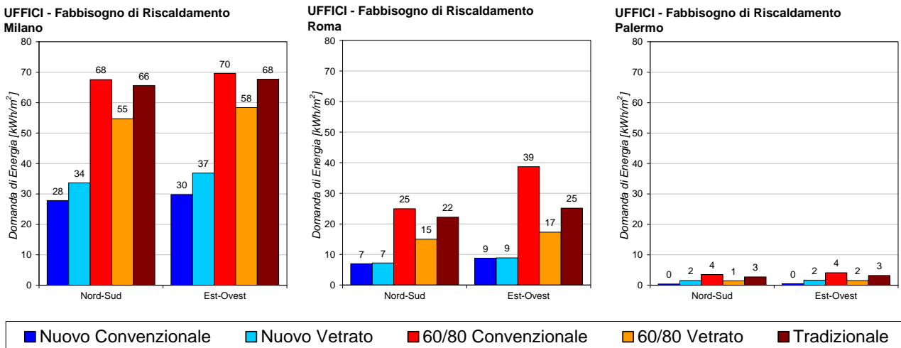
Figura 20. Fabbisogno di riscaldamento specifico relativo ai piani ad uso uffici nelle città di Milano, Roma e Palermo.
