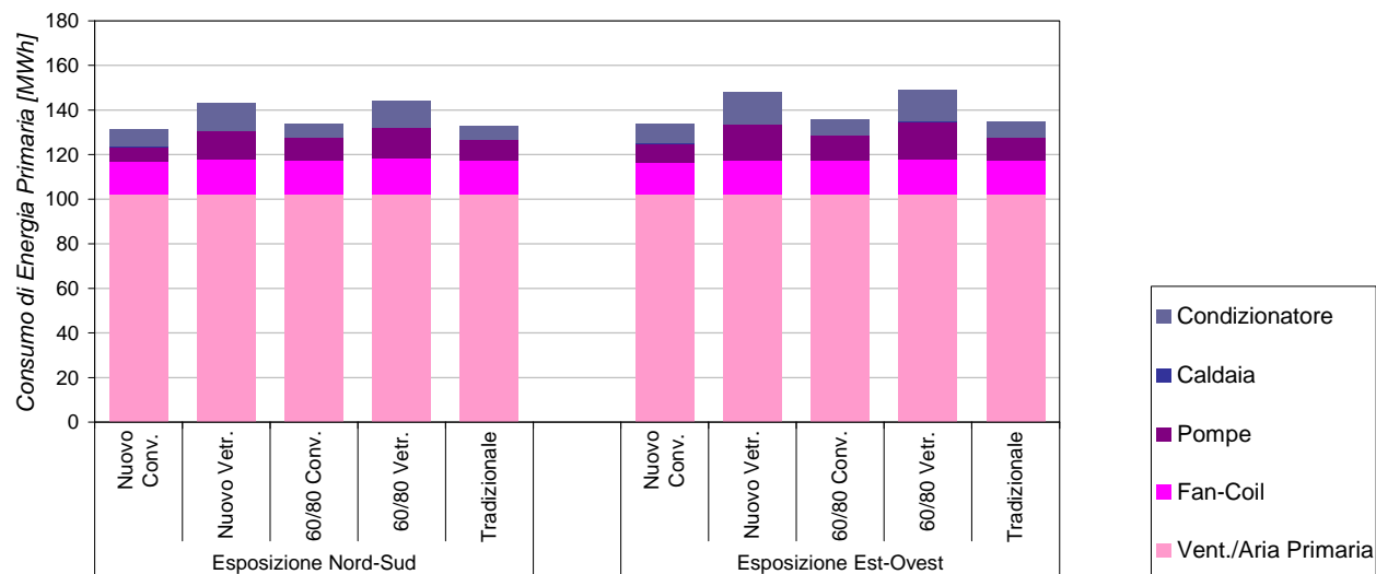
Figura 33. Composizione del consumo di energia primaria relativo agli ausiliari d’impianto per i piani adibiti ad uffici nella città di Milano.
