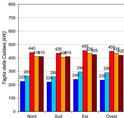
FILIALE - Taglia della Caldaia Pescara
