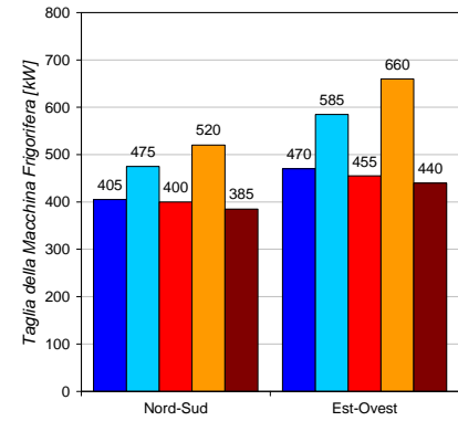
UFFICI - Taglia della Macchina Frigorifera Palermo
