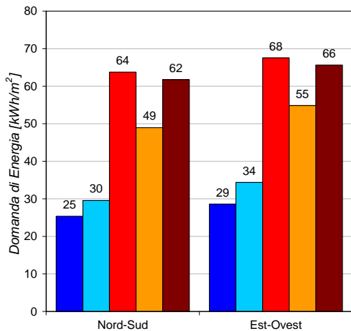
UFFICI - Fabbisogno di Riscaldamento
