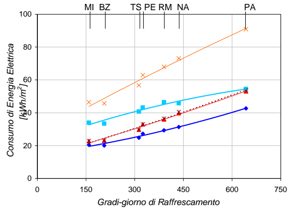
UFFICI - Energia Elettrica per Raffrescamento Esposizione Est-Ovest
