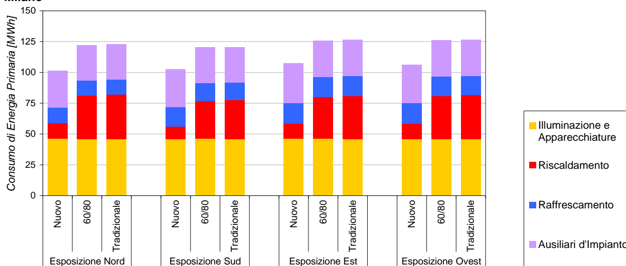
Figura 38. Composizione del consumo di energia primaria per il piano agenzia nella città di Milano.
