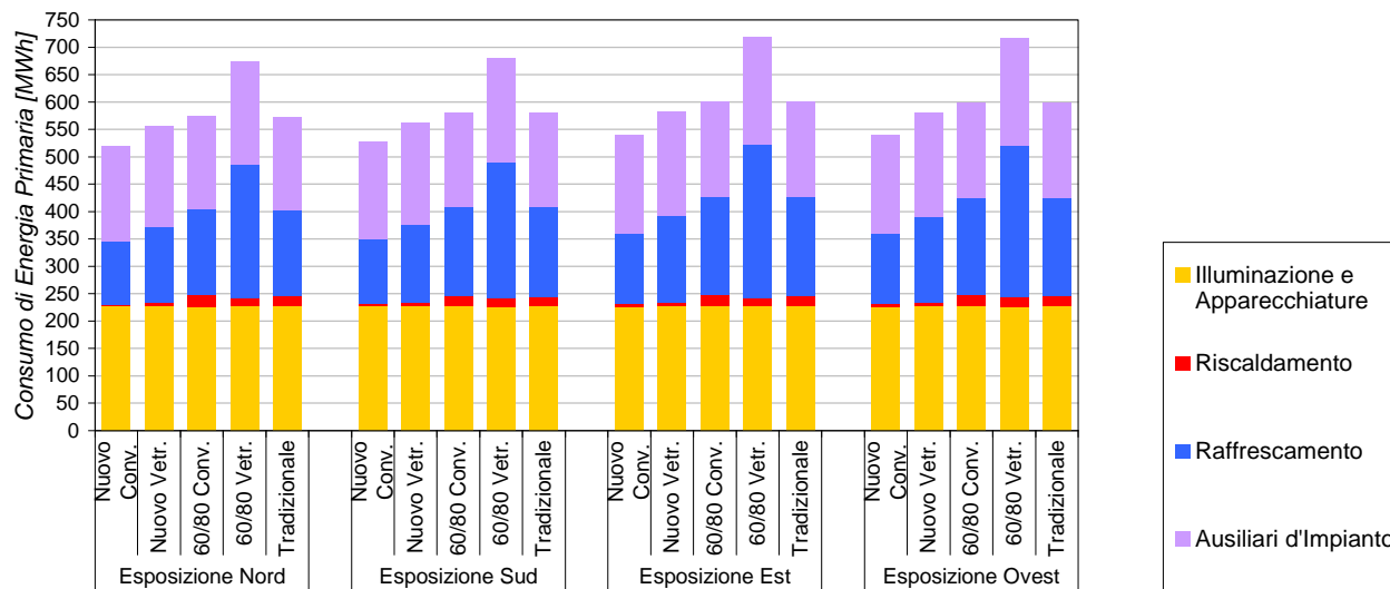
Figura 48. Composizione del consumo di energia primaria per l'edificio ad uso filiale nella città di Palermo.
