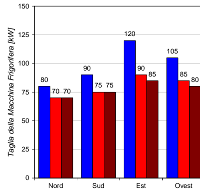
AGENZIA - Taglia della Macchina Frigorifera Roma
