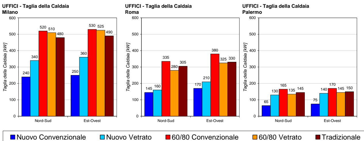
Figura 26. Taglia della caldaia per i piani ad uso ufficio nelle città di Milano, Roma e Palermo.
