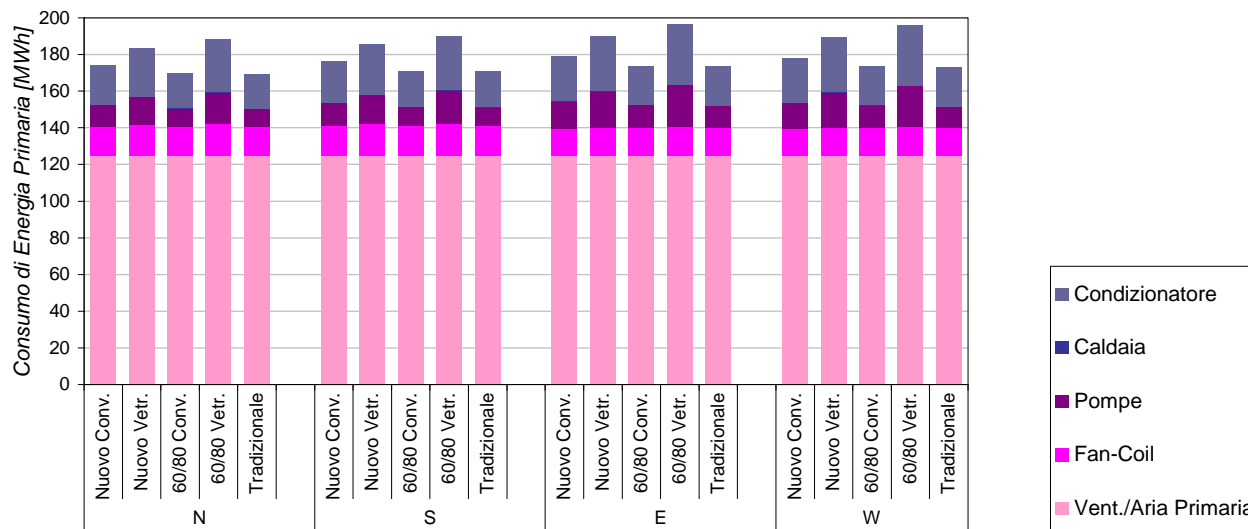
Figura 49. Composizione del consumo di energia primaria relativo agli ausiliari d’impianto per l’edificio ad uso filiale nella città di Palermo.
