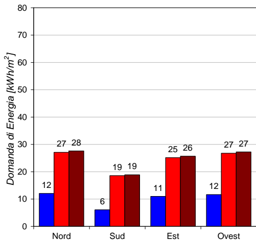
AGENZIA - Fabbisogno di Riscaldamento Pescara
