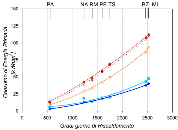
UFFICI - Energia Primaria per Riscaldamento Esposizione Nord-Sud
