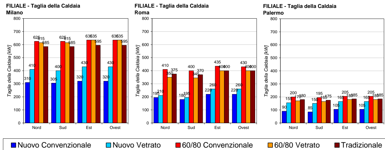
Figura 28. Taglia della caldaia per l'edificio ad uso filiale nelle città di Milano, Roma e Palermo.
