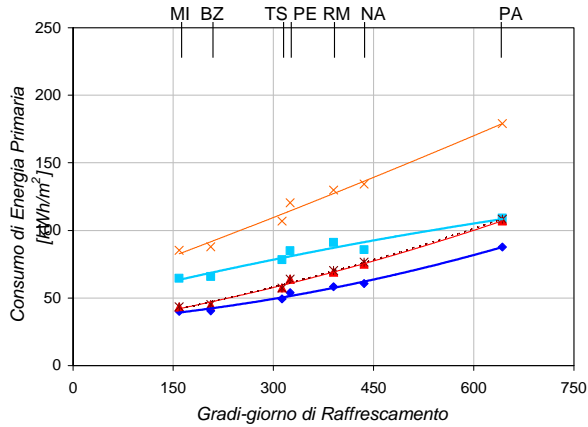
UFFICI - Energia Primaria per Raffrescamento Esposizione Nord-Sud
