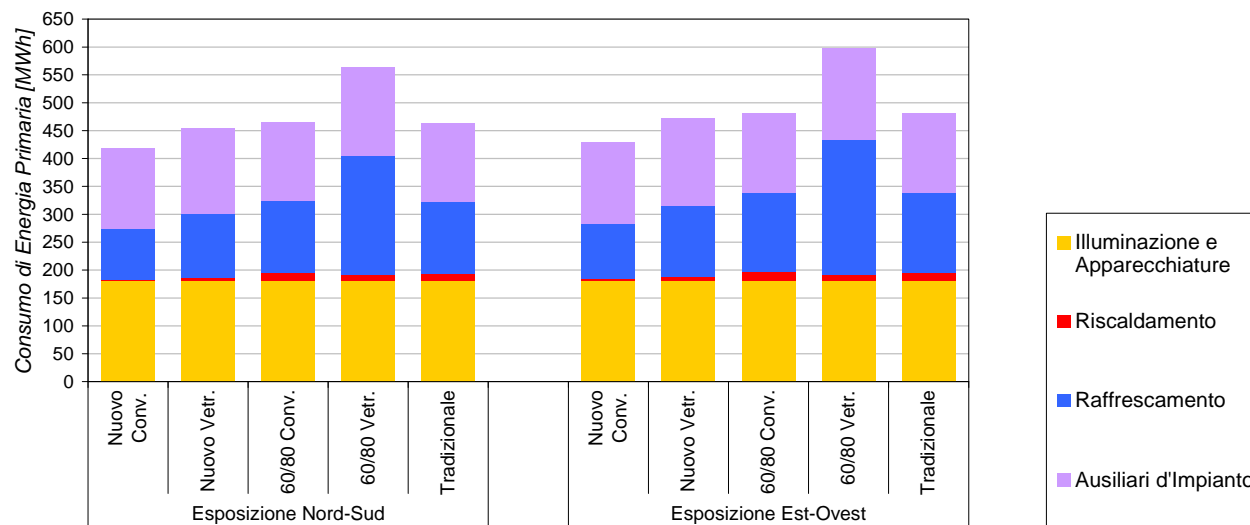
Figura 36. Composizione del consumo di energia primaria per i piani adibiti ad uffici nella città di Palermo.
