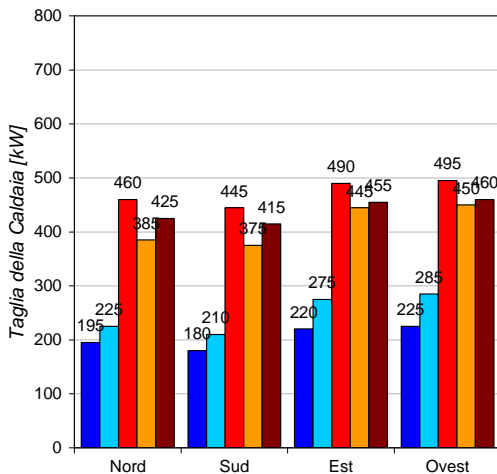
FILIALE - Taglia della Caldaia Trieste
