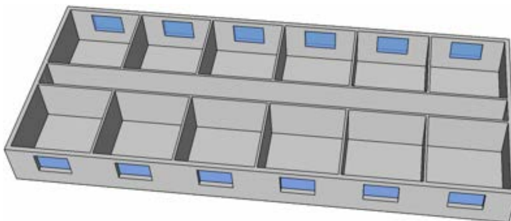
Figura 10: Schema tridimensionale di uno dei piani adibiti ad uffici (porzione finestrata convenzionale).
