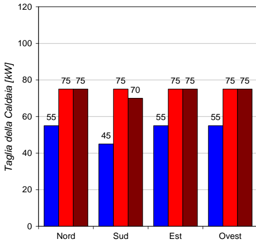
AGENZIA - Taglia della Caldaia Pescara
