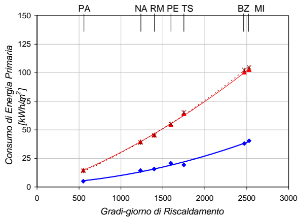
AGENZIA - Energia Primaria per Riscaldamento Esposizione Est
