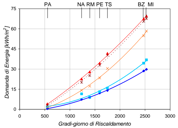
UFFICI - Fabbisogno di Riscaldamento Esposizione Est-Ovest
