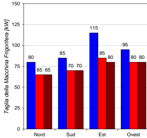
AGENZIA - Taglia della Macchina Frigorifera Bolzano
