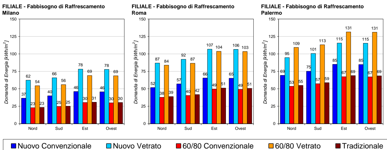
Figura 25. Fabbisogno di raffrescamento specifico relativo all’edificio ad uso filiale nelle città di Milano, Roma e Palermo.
