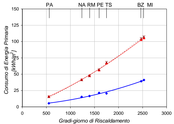
AGENZIA - Energia Primaria per Riscaldamento Esposizione Ovest
