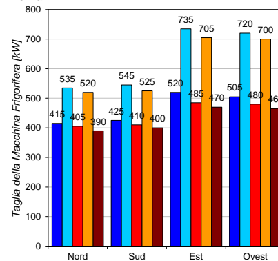
FILIALE - Taglia della Macchina Frigorifera Roma
