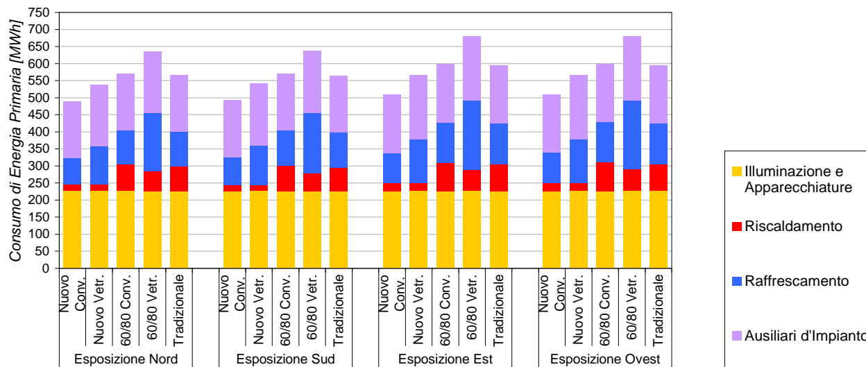
Figura 46. Composizione del consumo di energia primaria per l'edificio ad uso filiale nella città di Roma.
