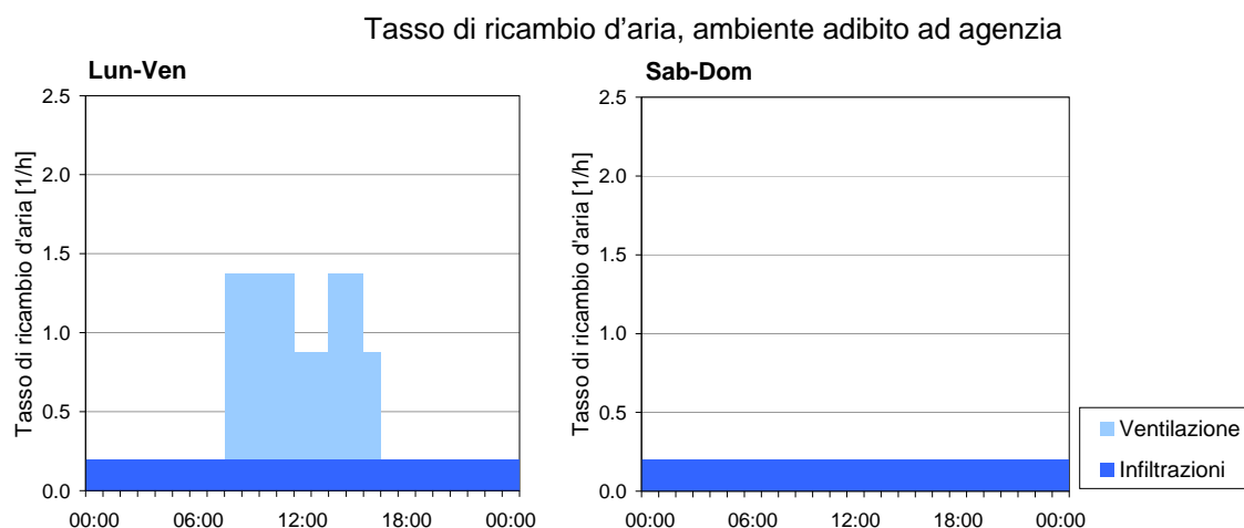
Figura 18: Profili orari del tasso di ricambio d'aria, in l/h, per i locali ad uso ufficio.
