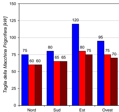
AGENZIA - Taglia della Macchina Frigorifera Milano
