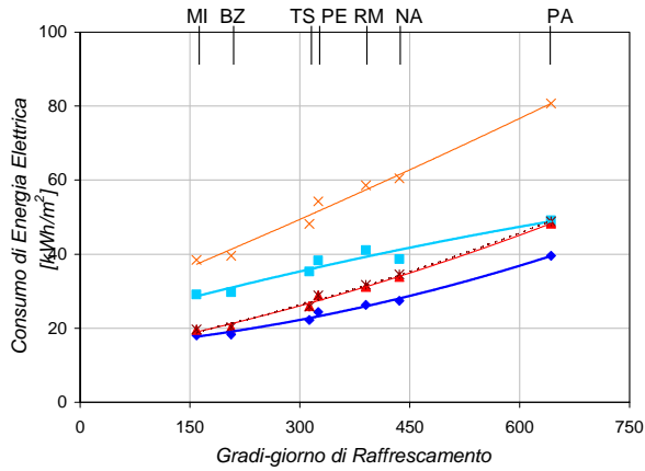
UFFICI - Energia Elettrica per Raffrescamento Esposizione Nord-Sud
