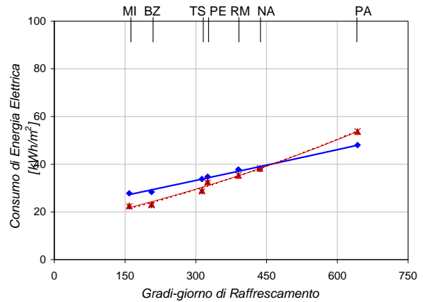
AGENZIA - Energia Elettrica per Raffrescamento Esposizione Ovest
