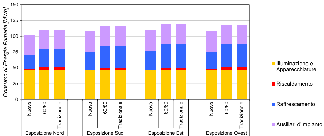
Figura 42. Composizione del consumo di energia primaria per il piano agenzia nella città di Palermo.
