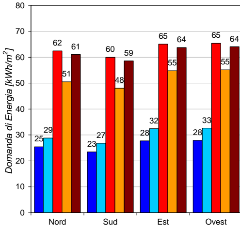
FILIALE - Fabbisogno di Riscaldamento Bolzano
