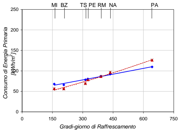
AGENZIA - Energia Primaria per Raffrescamento Esposizione Est
