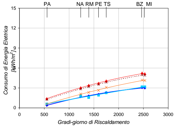
UFFICI - Energia Elettrica per Riscaldamento Esposizione Est-Ovest
