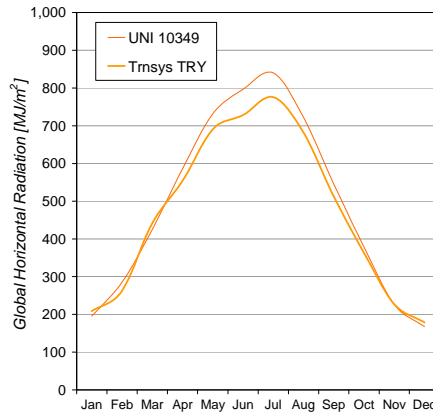
Figura 6. Valori medi mensili di temperatura dell'aria e di radiazione solare globale sull'orizzontale secondo norma UNI 10349 e derivati dal TRY fornito con TRNSYS. Città di Roma.
