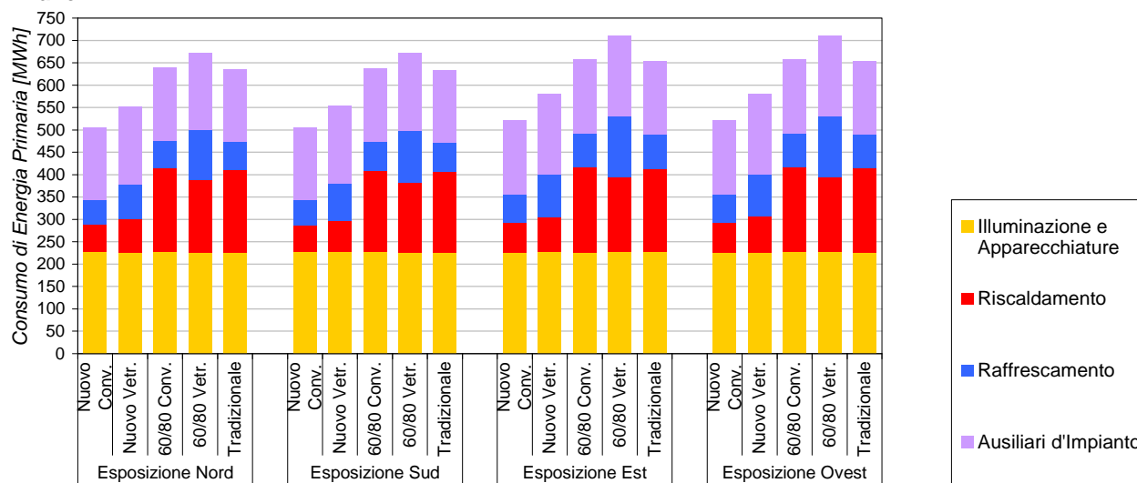
Figura 44. Composizione del consumo di energia primaria per l'edificio ad uso filiale nella città di Milano.
