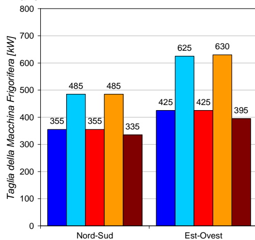
UFFICI - Taglia della Macchina Frigorifera
