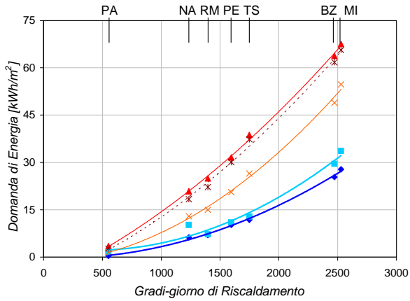
UFFICI - Fabbisogno di Riscaldamento Esposizione Nord-Sud
