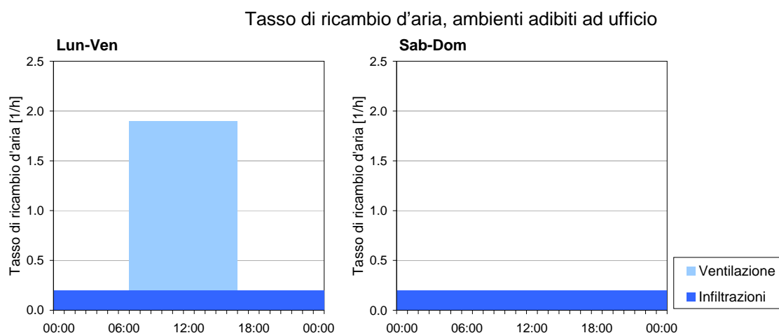
Figura 14: Profili orari del tasso di ricambio d'aria, in 1/h, per i locali ad uso ufficio.
