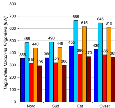
FILIALE - Taglia della Macchina Frigorifera Milano
