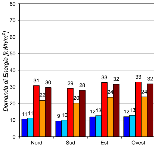
FILIALE - Fabbisogno di Riscaldamento Pescara
