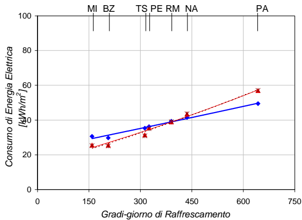
AGENZIA - Energia Elettrica per Raffrescamento Esposizione Est
