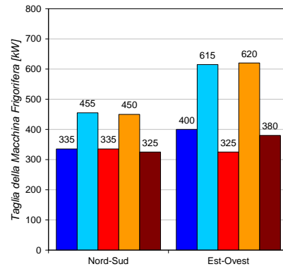
UFFICI - Taglia della Macchina Frigorifera Roma
