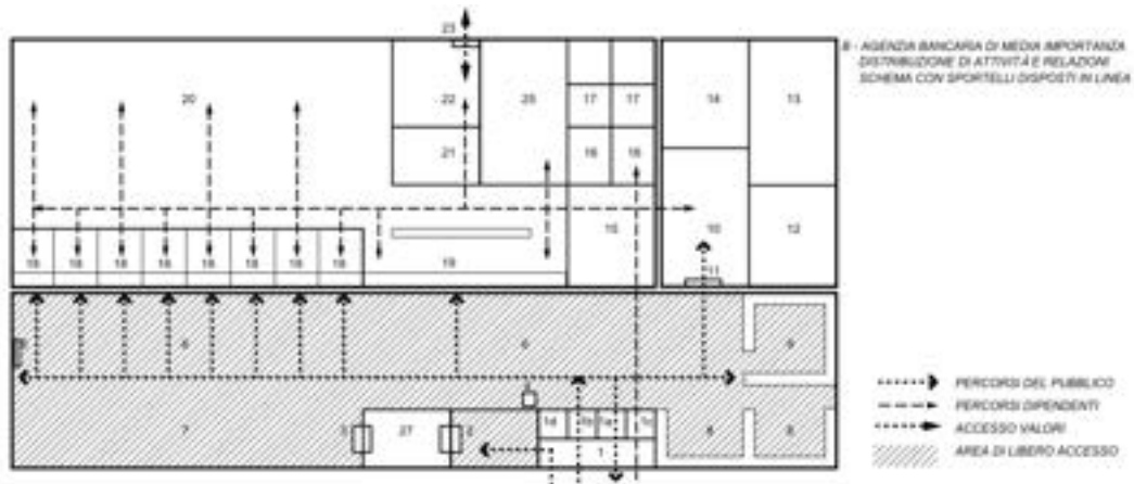
Figura 15: Schema distributivo di un'agenzia bancaria di media importanza (fonte: Zevi, 2003).
