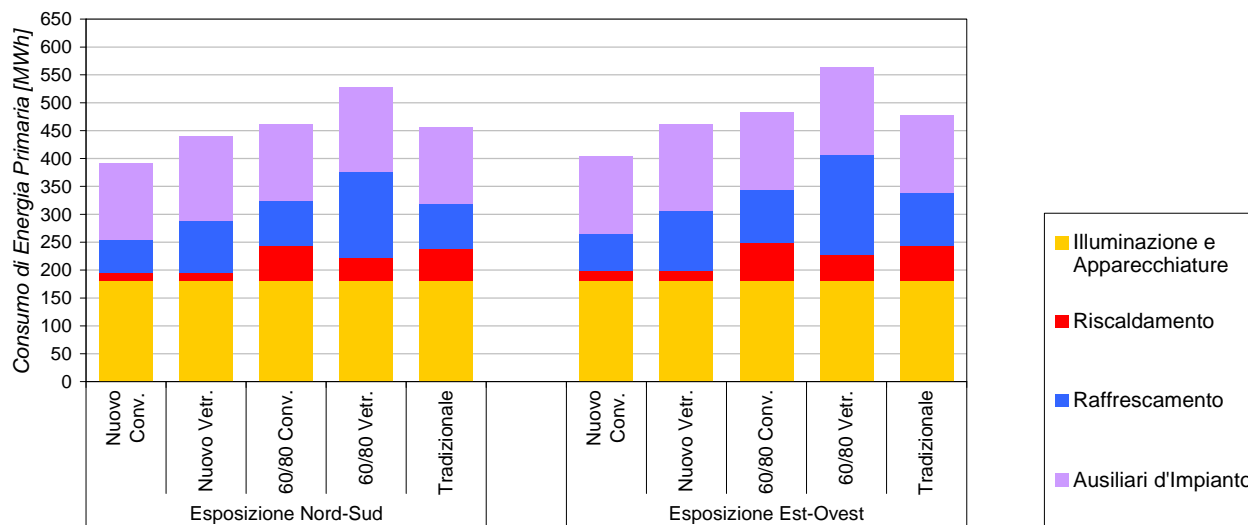
Figura 34. Composizione del consumo di energia primaria per i piani adibiti ad uffici nella città di Roma.
