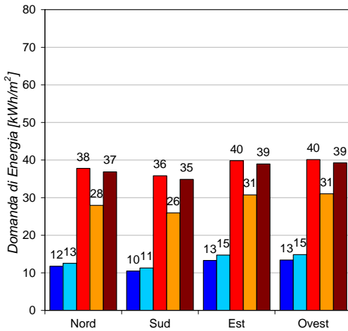
FILIALE - Fabbisogno di Riscaldamento Trieste
