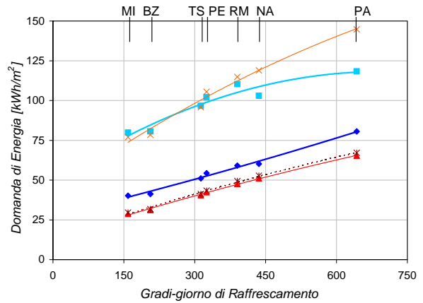
UFFICI - Fabbisogno di Raffrescamento Esposizione Est-Ovest
