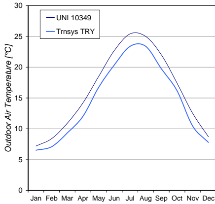
Figura 5. Valori medi mensili di temperatura dell'aria e di radiazione solare globale sull'orizzontale secondo norma UNI 10349 e derivati dal TRY fornito con TRNSYS. Città di Pescara.
