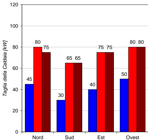
AGENZIA - Taglia della Caldaia Trieste
