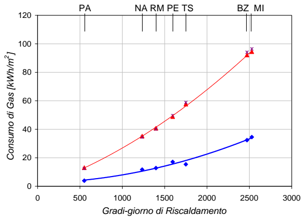
AGENZIA - Gas per Riscaldamento Esposizione Est
