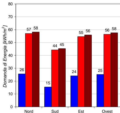
AGENZIA - Fabbisogno di Riscaldamento Bolzano
