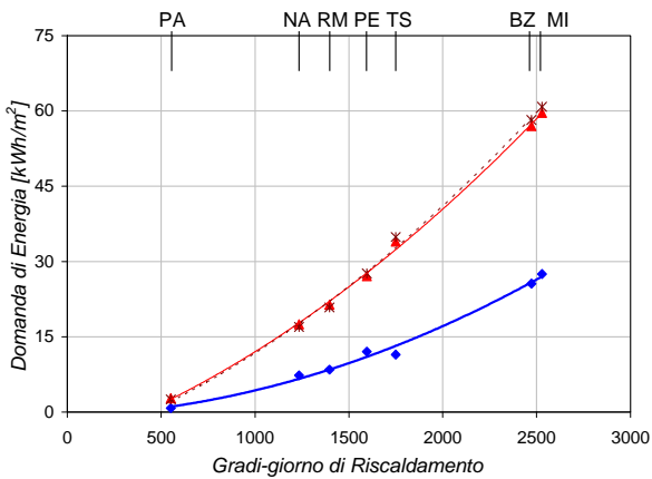
AGENZIA - Fabbisogno di Riscaldamento Esposizione Est
