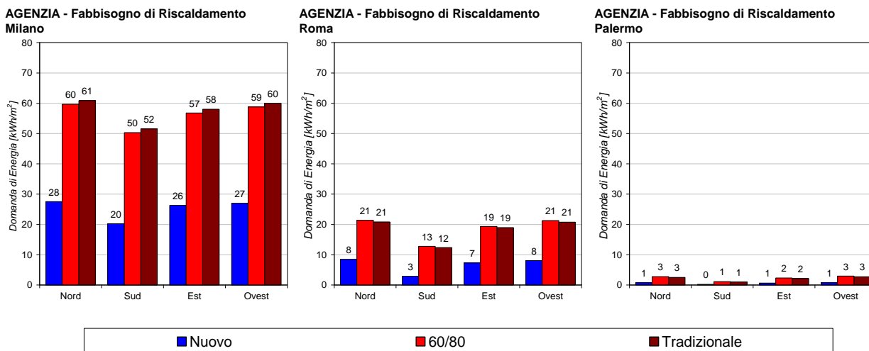
Figura 22. Fabbisogno di riscaldamento specifico relativo al piano agenzia nelle città di Milano, Roma e Palermo.
