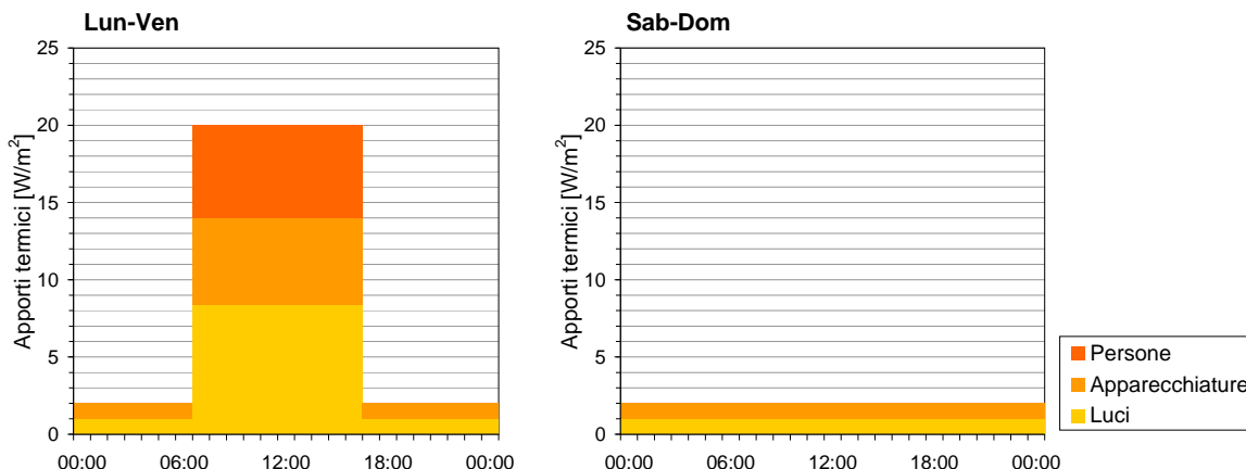
Figura 12: Profili orari dei carichi termici interni complessivi, in W/m 2 , nei locali ad uso ufficio.
