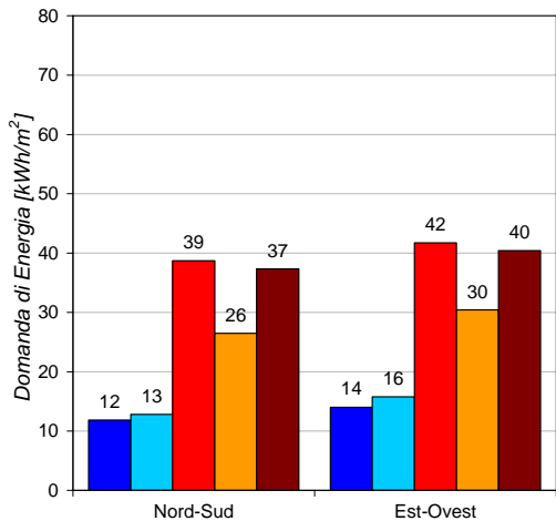
UFFICI - Fabbisogno di Riscaldamento
