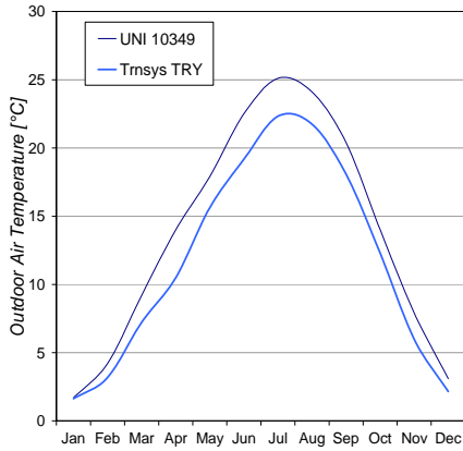
Figura 2. Valori medi mensili di temperatura dell'aria e di radiazione solare globale sull'orizzontale secondo norma UNI 10349 e derivati dal TRY fornito con TRNSYS. Città di Milano.
