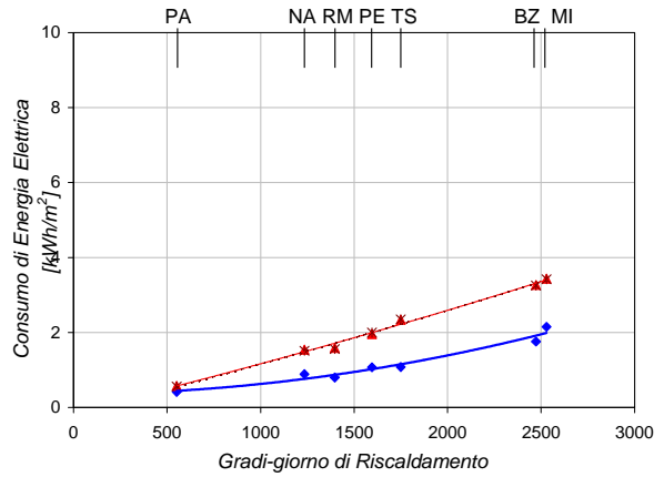
AGENZIA - Energia Elettrica per Riscaldamento Esposizione Ovest
