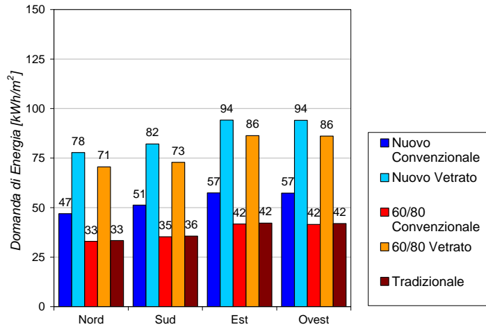
FILIALE - Fabbisogno di Raffrescamento Trieste
