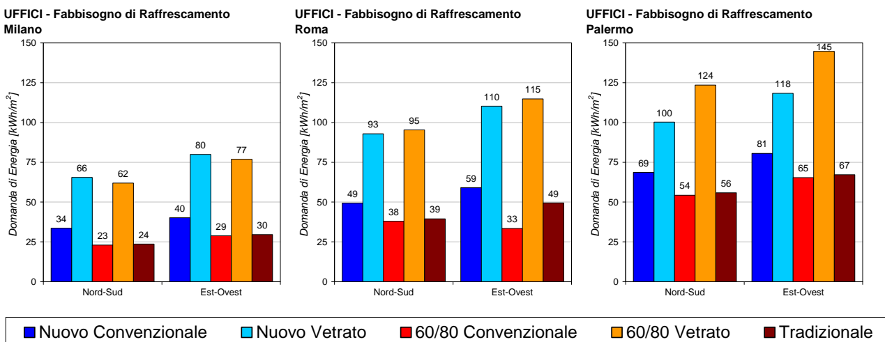
Figura 21. Fabbisogno di raffrescamento specifico relativo ai piani ad uso uffici nelle città di Milano, Roma e Palermo.
