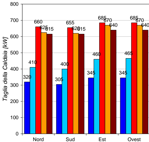
FILIALE - Taglia della Caldaia Bolzano
