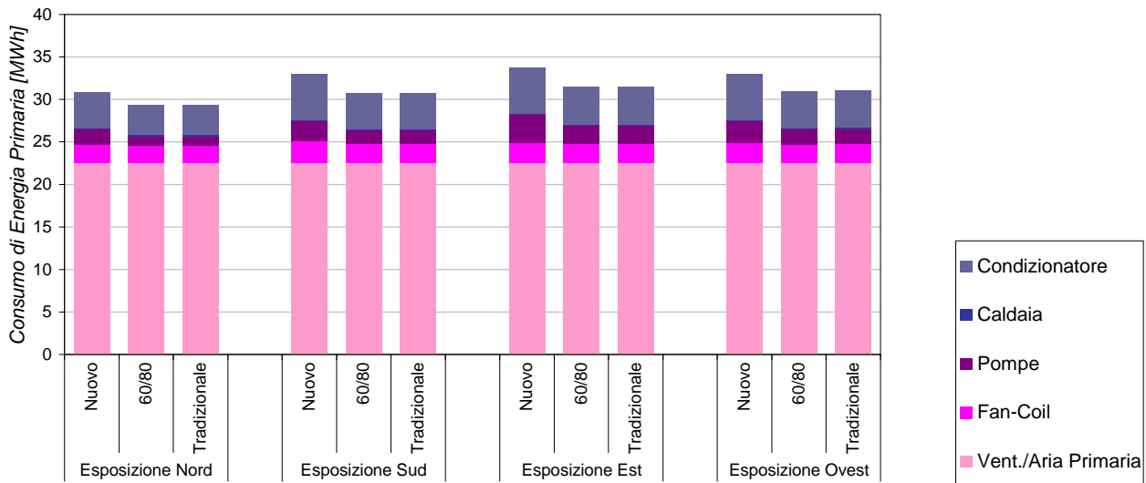
Figura 43. Composizione del consumo di energia primaria relativo agli ausiliari d'impianto per il piano agenzia nella città di Palermo.
