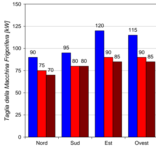
AGENZIA - Taglia della Macchina Frigorifera Pescara
