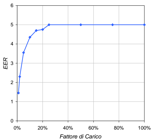
Figura 19. Curve di efficienza delle macchine frigorifere utilizzate nello studio, per gli edifici di nuova costruzione (sx) e per quelli più vecchi (dx).
