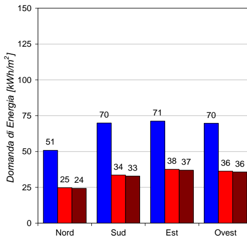
AGENZIA - Fabbisogno di Raffrescamento Bolzano
