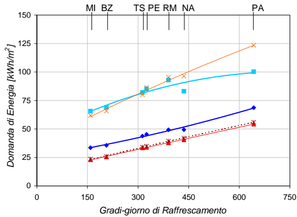
UFFICI - Fabbisogno di Raffrescamento Esposizione Nord-Sud
