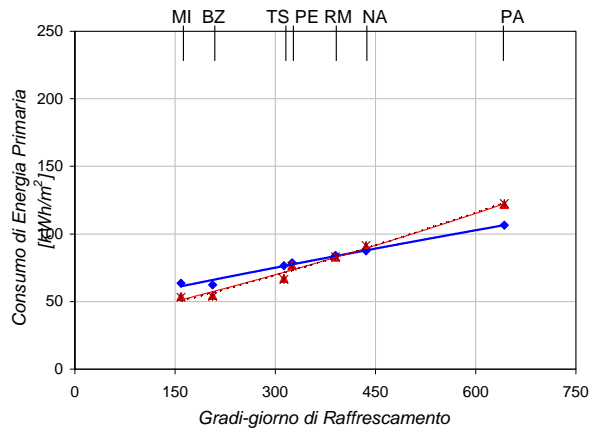
AGENZIA - Energia Primaria per Raffrescamento Esposizione Ovest
