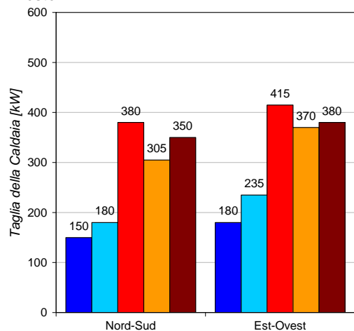
UFFICI - Taglia della Caldaia
