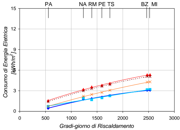
UFFICI - Energia Elettrica per Riscaldamento Esposizione Nord-Sud
