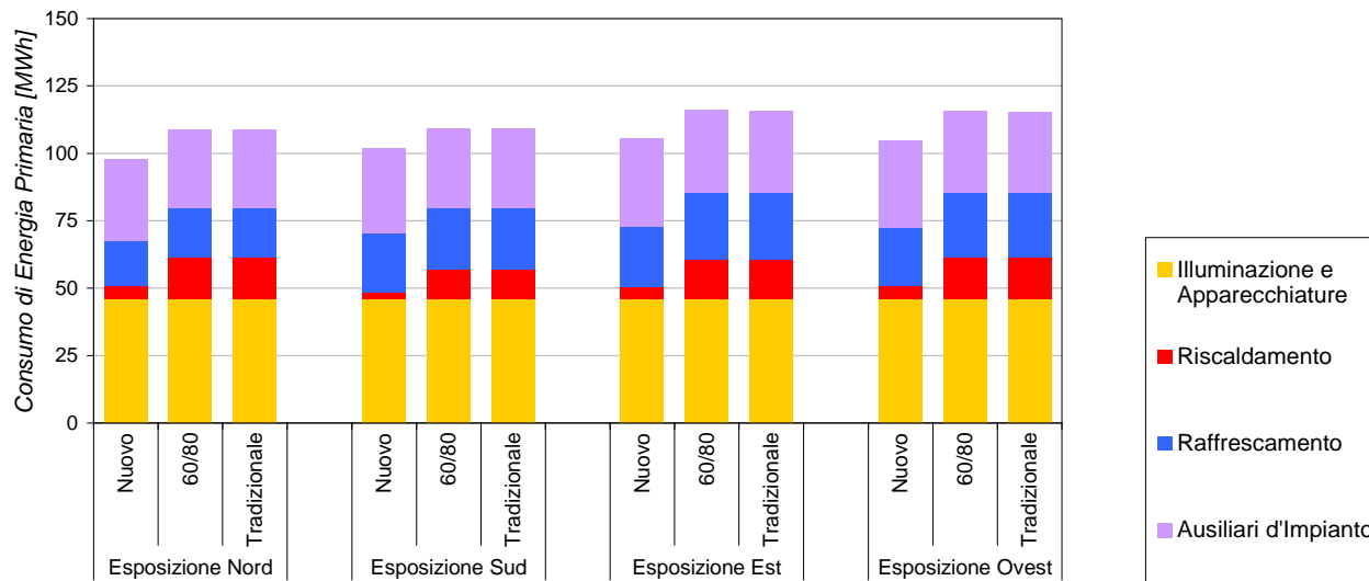
Figura 40. Composizione del consumo di energia primaria per il piano agenzia nella città di Roma.
