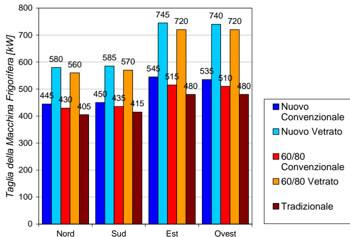
FILIALE - Taglia della Macchina Frigorifera Pescara
