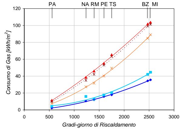
UFFICI - Gas per Riscaldamento Esposizione Est-Ovest
