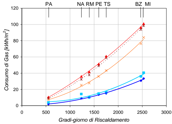
UFFICI - Gas per Riscaldamento Esposizione Nord-Sud
