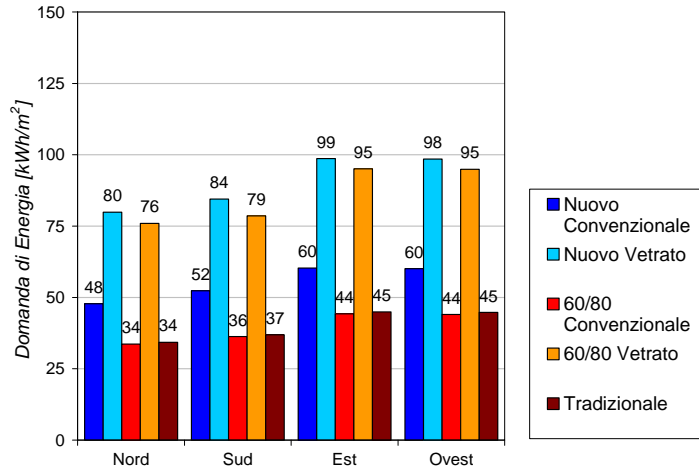
FILIALE - Fabbisogno di Raffrescamento Pescara
