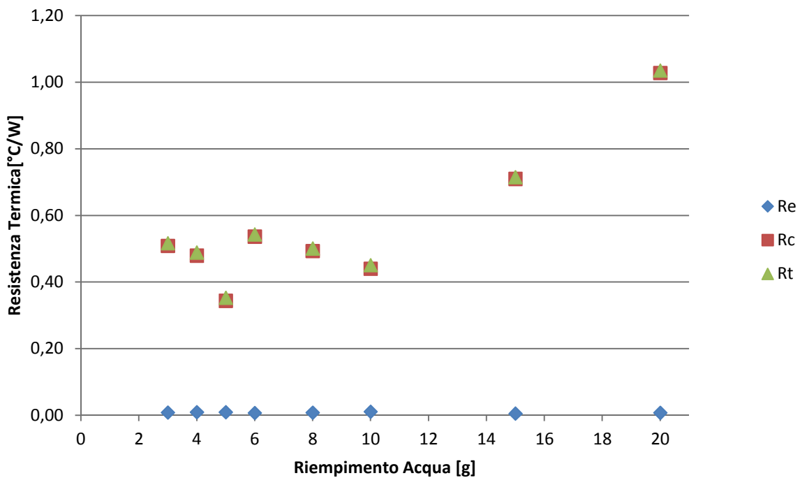
Fig. 3.20 – Resistenze termiche all'evaporatore, al condensatore e totale. Q_{in} = 155 W.
