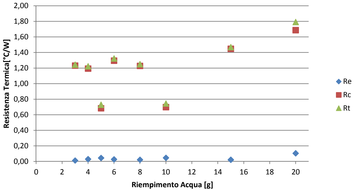
Fig. 3.19 – Resistenze termiche all'evaporatore, al condensatore e totale. Q_{in} = 70 W.
