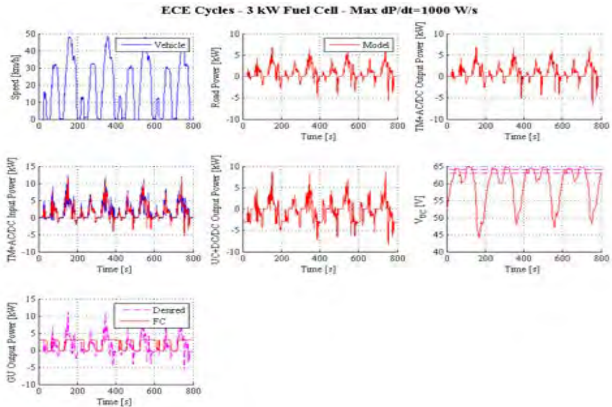
Figura 50 – Ibrido serie con FC e UC; Ciclo ECE; Strategia Start & Stop. Andamenti temporali
