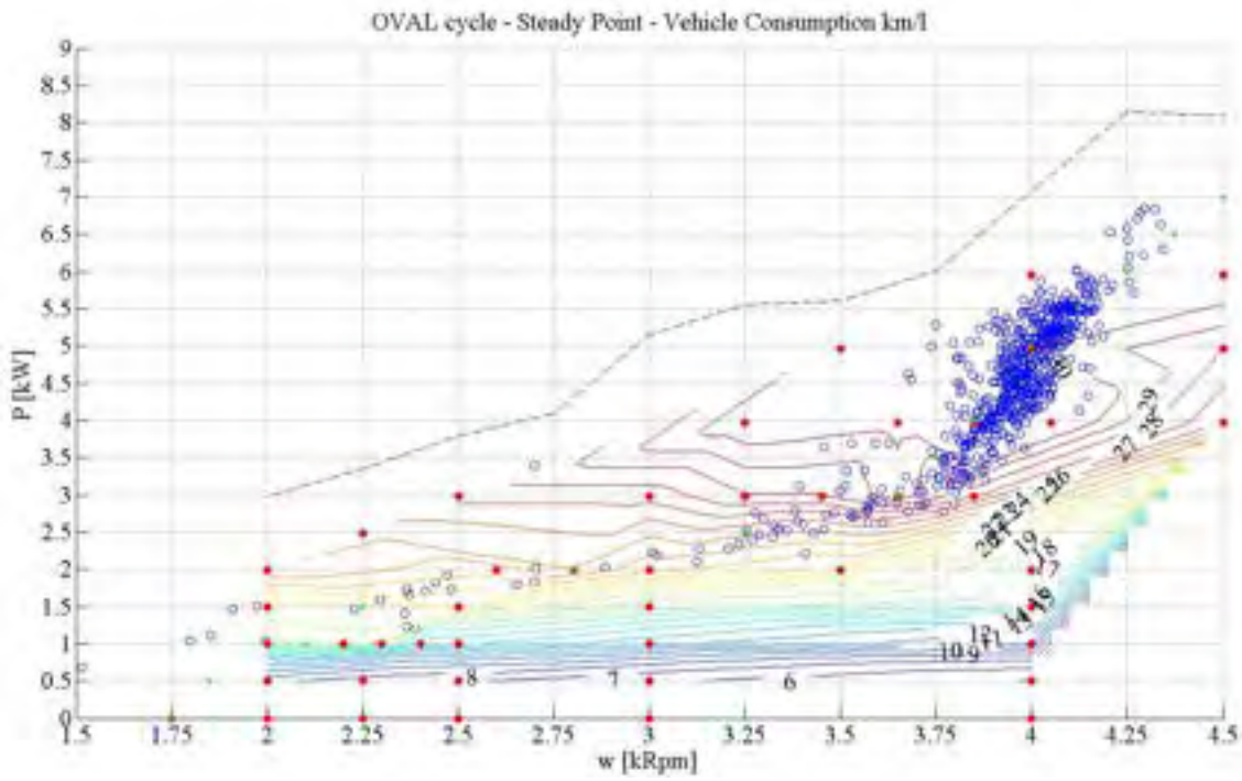
Figura 42 - Ciclo "Oval" con ON OFF + Load following: principali risultati
