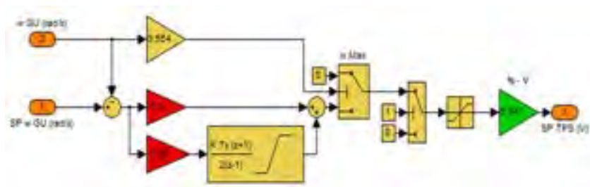
Figura 24 - Blocco ICE
