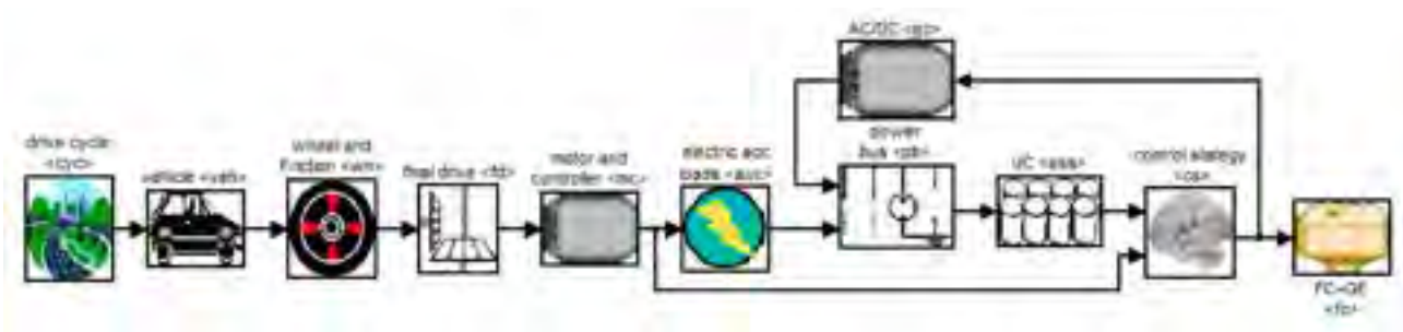
Figura 44 – Modello del sistema propulsivo e del veicolo
