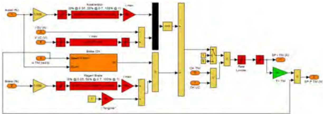
Figura 22 - Blocco TM
