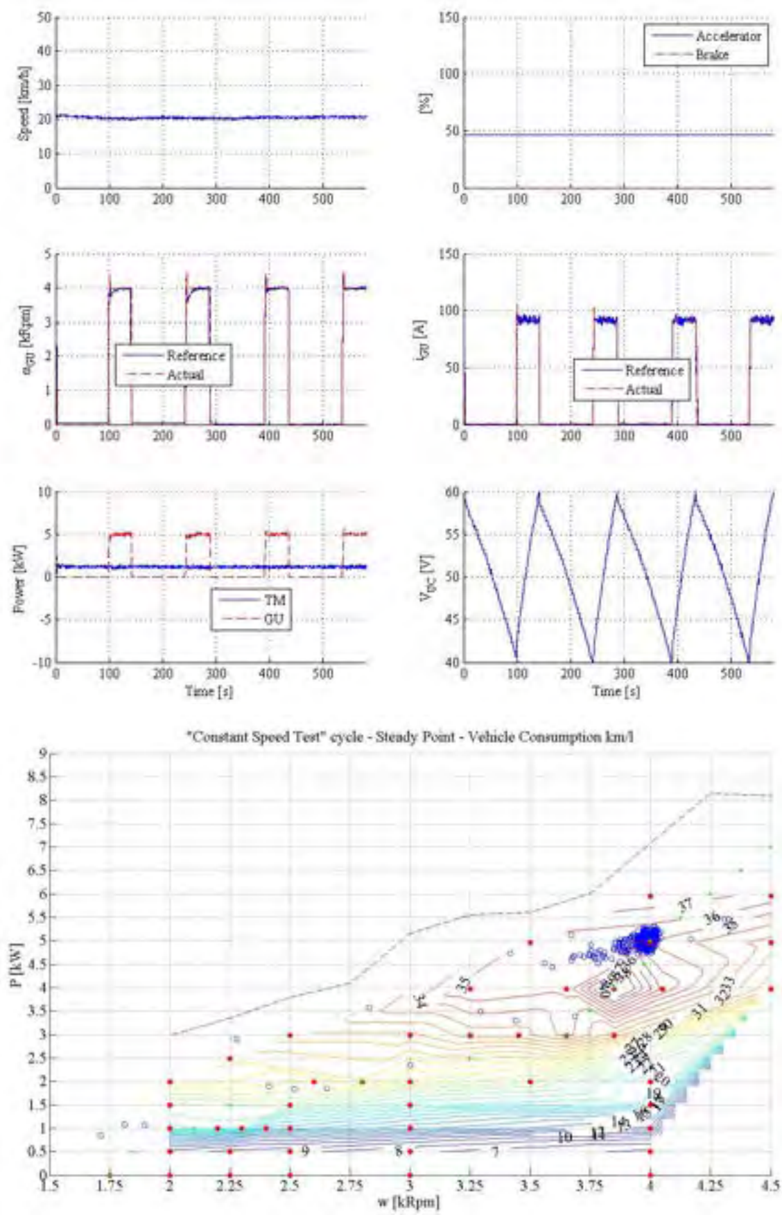
Figura 37 - Ciclo "Marathon" con ON OFF: principali risultati
