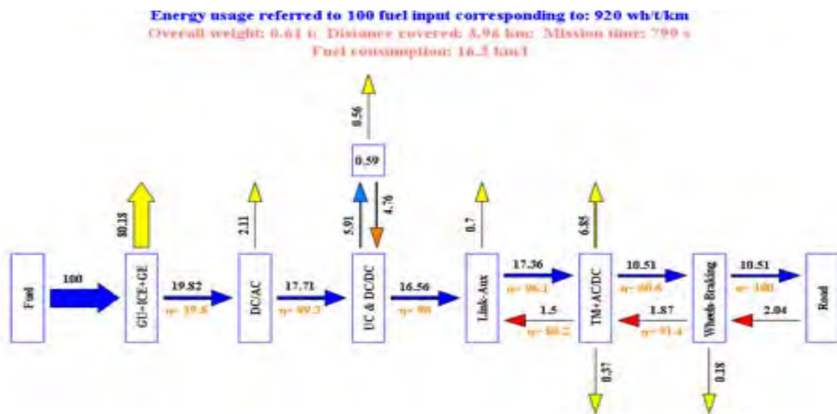
Figura 47 – Ibrido serie con MCI; Ciclo ECE; Strategia load follower. Flussi energetici
