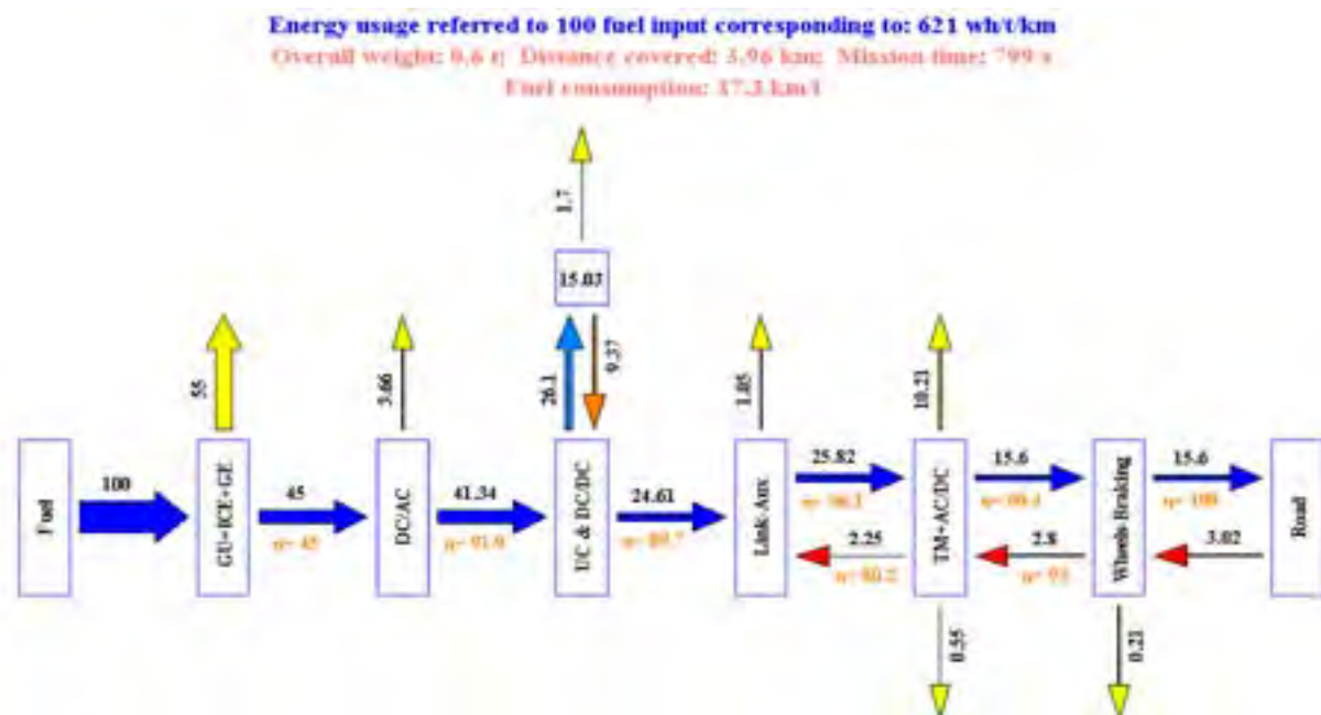
Figura 53 - Ibrido serie con FC e batt. ThunderSky; Ciclo ECE; Strat. Start & Stop. Flussi energetici
