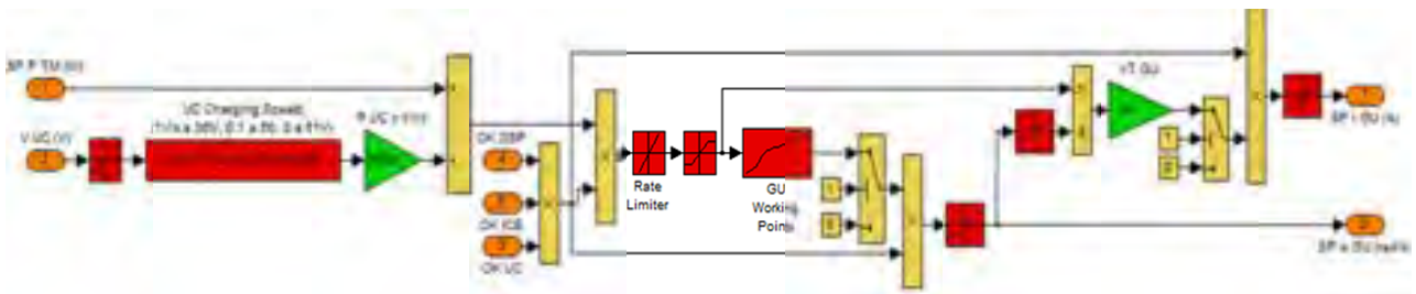
Figura 23 - Blocco GU
