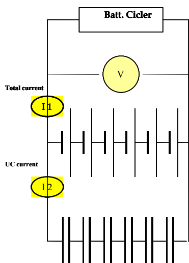
Fig. 1 - Schema e realizzazione dell'accumulo misto batterie + supercondensatori
