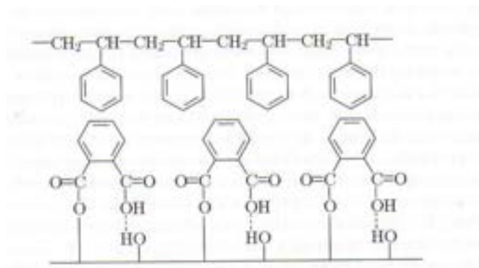
Fig.4.1 Ipotesi di interazione tra anidride italica e polistirene
