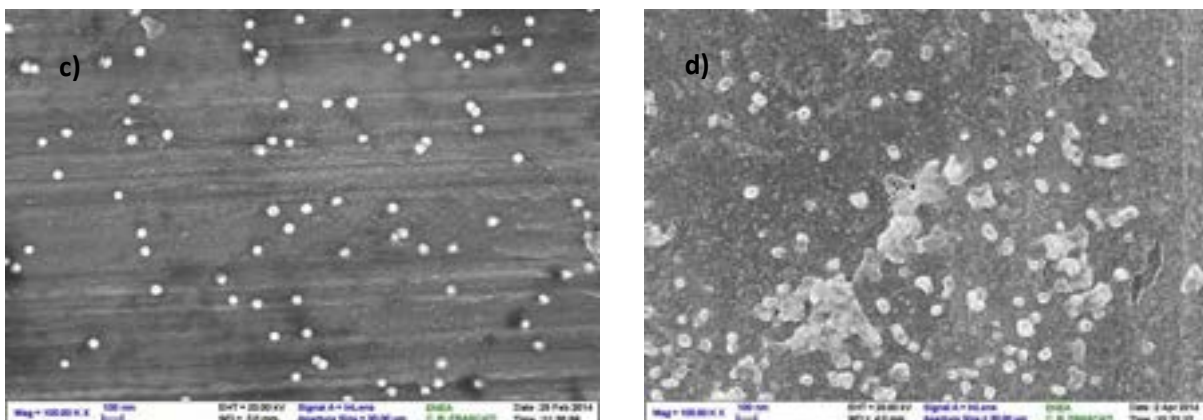
Figura 9c,d. Foto SEM ad alto ingrandimento di Au colloidale su acciaio prima (c) e dopo (d) l'annealing.
