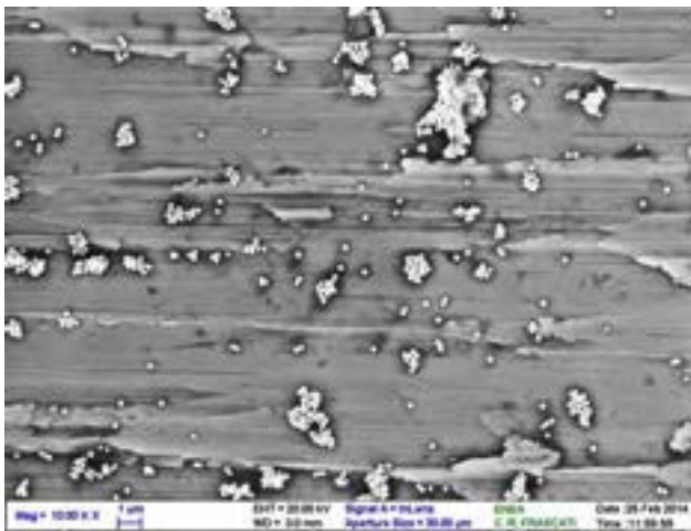
Figura 2a. Au colloidale depositato su acciaio con il metodo della goccia.
