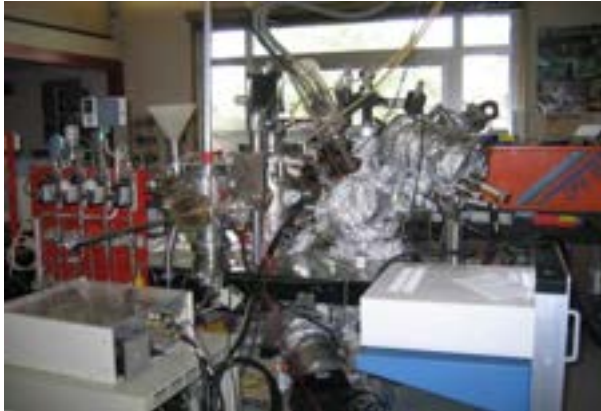
Figura 11. Sistema di deposizione CVD e sistema di analisi XPS presso UTAPRAD-MNF.
