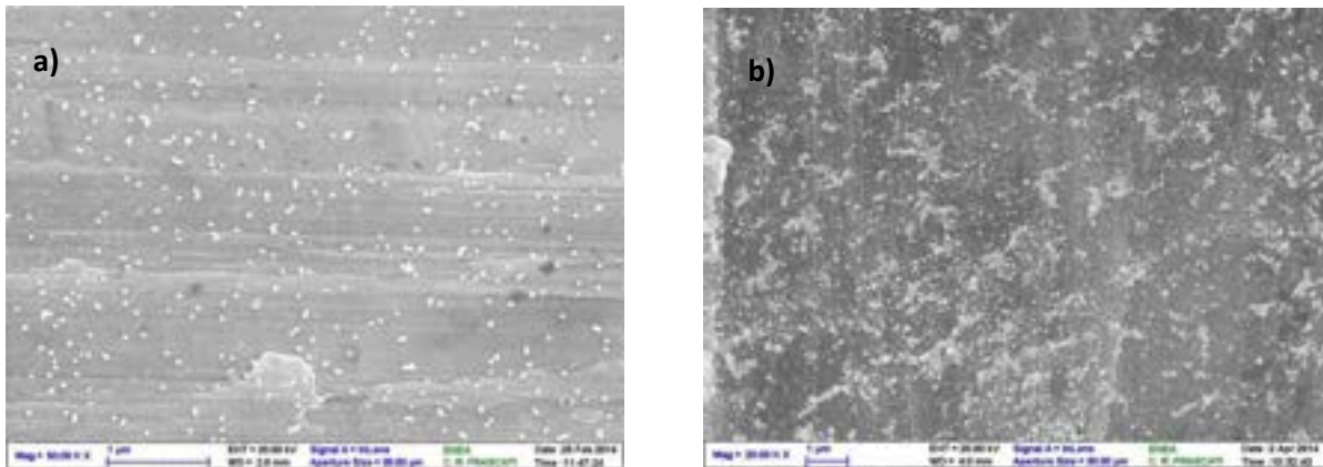
Figura 9a,b. Foto SEM a basso ingrandimento di Au colloidale su acciaio prima (a) e dopo (b) l'annealing.
