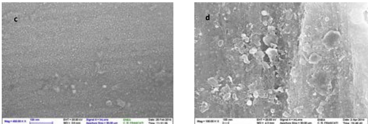
Figura 10c,d. Foto SEM di Au depositato tramite e-beam su acciaio (substrato #27) prima (c) e dopo (d) l'annealing.
