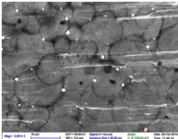
Figura 4a. Foto SEM a basso ingrandimento che evidenzia i diametri delle microgocce
