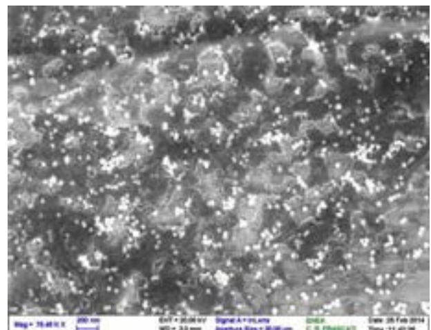
Figura 4b. Foto SEM: deposizione di Au colloidale 40nm con nebulizzatore
