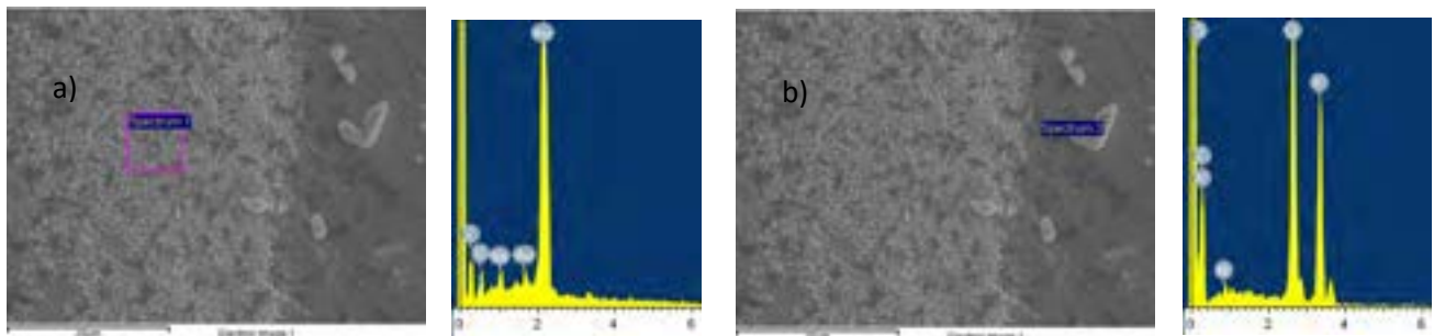
Fig. 2e: a) Spettro EDX sulle nanoparticelle di Au deposte da sospensione colloidale. b) Spettro EDX sui grani originati dalla sospensione colloidale
