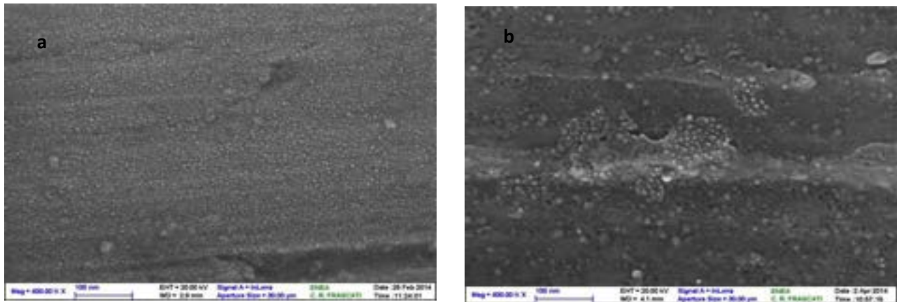
Figura 10a,b. Foto SEM di Au depositato tramite e-beam su acciaio (substrato #10) prima (a) e dopo (b) l'annealing.
