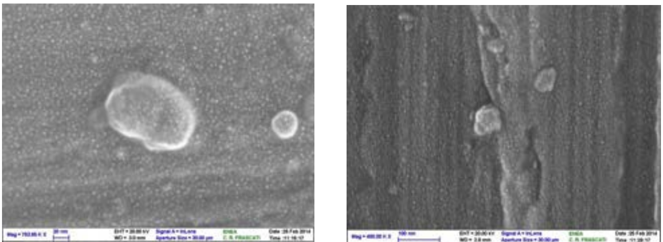
Figura 6: Immagini SEM ad alta risoluzione raffiguranti nanoparticelle di Au su acciaio ottenute mediante evaporazione PVD
