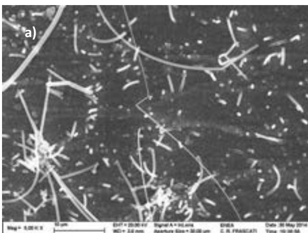
Figura 13a. Immagine SEM di un campione non sottoposto ad annealing preliminare prima della funzionalizzazione.
