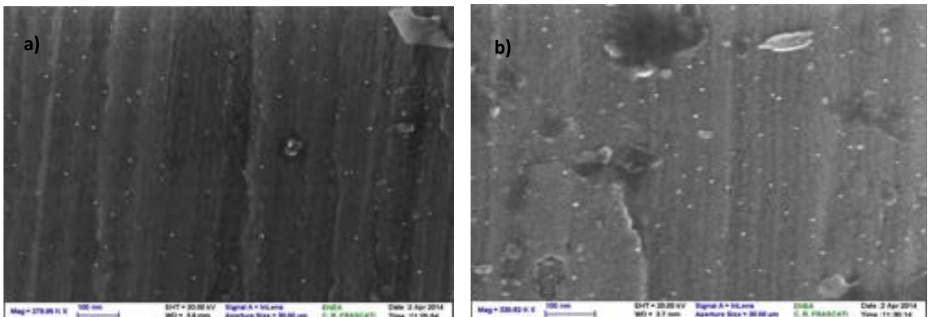
Figura 7: Immagini SEM ad alta risoluzione raffiguranti nanoparticelle di Au su acciaio ottenute mediante evaporazione PVD; a) t=30"; b) t=60"
