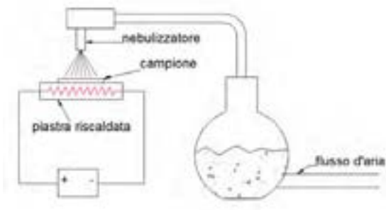
Fig. 3. Schema del sistema di nebulizzazione utilizzato per depositare l'Au da sospensione colloidale.
