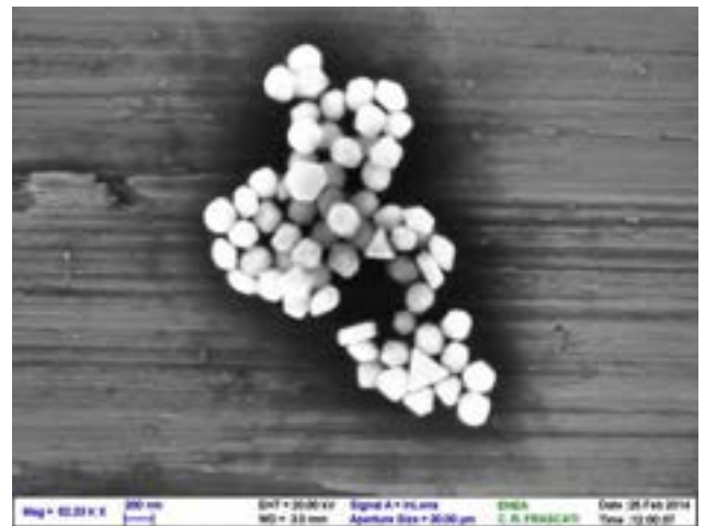
Figura 2b. Esempio di un aggregato di Au colloidale 200 nm formatosi su acciaio con il metodo della goccia.
