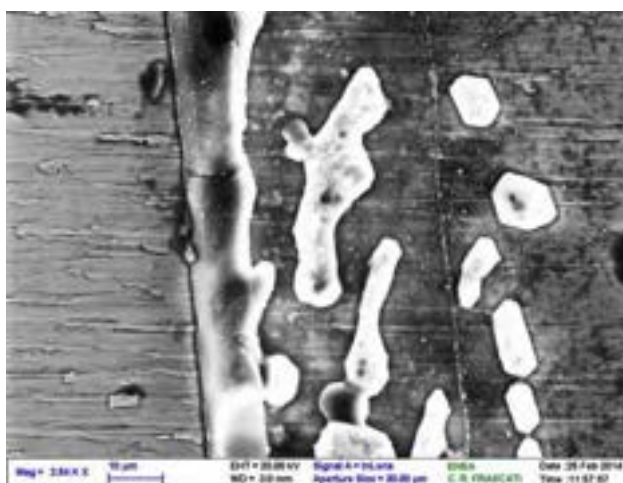
Figura 2c. Agglomerati dovuti alla presenza di stabilizzatori nella sospensione colloidale
