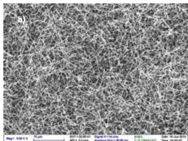
Figura 13b. Immagine SEM del campione #65 annilato a 700 °C prima di essere funzionalizzato con Au .
