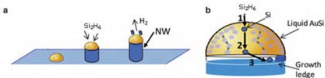
Fig.1 Schema del meccanismo di crescita VLS.
