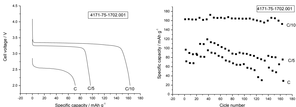
Figura 19. Profili di tensione in funzione della capacità specifica (a sinistra) e capacità specifica in funzione del numero dei cicli (a destra) per un elettrodo a base di \text{LiFePO}_4 per celle ad alta capacità fatto ciclare in una cella al litio metallico. La cella è fatta ciclare a C/10, C/5 e C rate. La carica è stata effettuata galvanostaticamente a C rate fino a 4.2 Volt seguita da una carica potenziostatica a 4.2 Volt fin quando la corrente diminuisce ad un valore pari a C/10.
