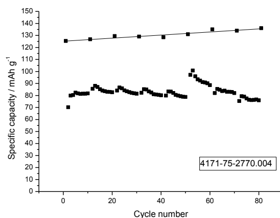
Figura 18. Profili di tensione in funzione del tempo (a sinistra) e capacità specifica in funzione del numero dei cicli (a destra) per un elettrodo a base di LiFePO 4 fatto ciclare in una cella al litio metallico. La cella è fatta ciclare a C rate. Ogni 10 cicli è stato effettuato un ciclo a C/10 per valutare la capacità esibita dall'elettrodo quando scaricato in condizioni meno stressanti. La carica è stata effettuata galvanostaticamente a C rate fino a 4.2 Volt seguita da una carica potenziostatica a 4.2 Volt fin quando la corrente diminuisce ad un valore pari a C/10.
