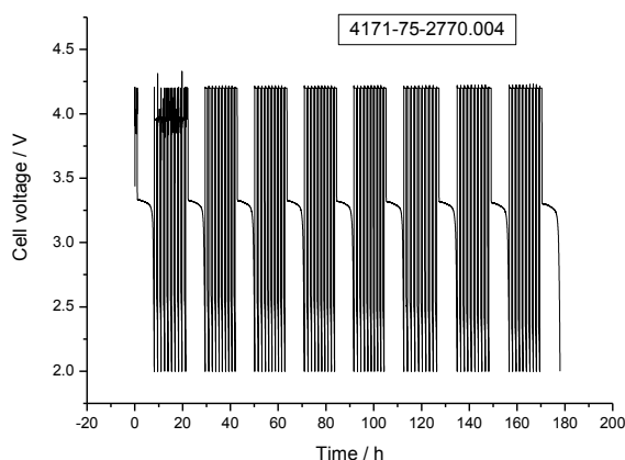
Figura 18. Profili di tensione in funzione del tempo (a sinistra) e capacità specifica in funzione del numero dei cicli (a destra) per un elettrodo a base di LiFePO 4 fatto ciclare in una cella al litio metallico. La cella è fatta ciclare a C rate. Ogni 10 cicli è stato effettuato un ciclo a C/10 per valutare la capacità esibita dall'elettrodo quando scaricato in condizioni meno stressanti. La carica è stata effettuata galvanostaticamente a C rate fino a 4.2 Volt seguita da una carica potenziostatica a 4.2 Volt fin quando la corrente diminuisce ad un valore pari a C/10.
