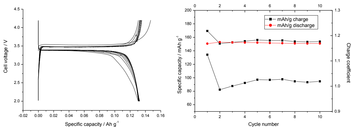
Figura 20. Profili di tensione in funzione della capacità specifica (a sinistra) e capacità specifica in funzione del numero dei cicli (a destra) per un elettrodo a base di \text{LiFePO}_4 fatto ciclare in una cella al litio metallico a rate di carica/scarica pari a C/10 .
