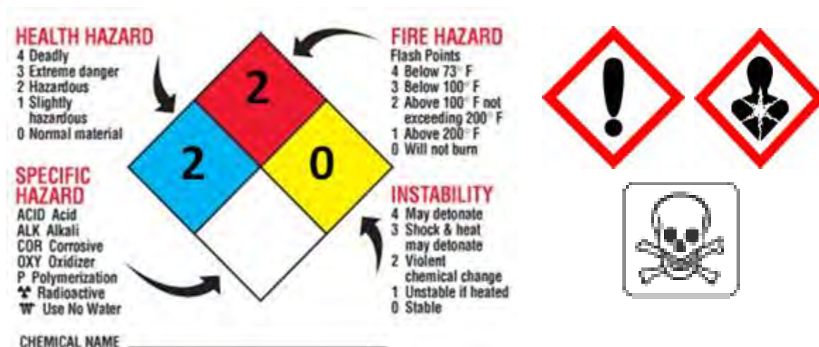
Figura 2. Caratteristiche di sicurezza della National Fire Protection Association e simboli di pericoli della Globally Harmonized System of Classification and Labelling of Chemicals e European Hazard Code relativi all'N-metil pirrolidone.
