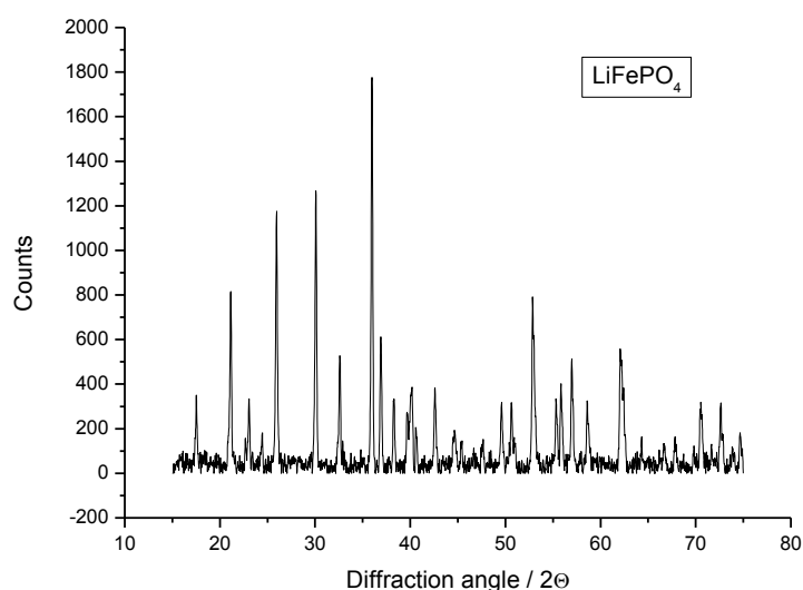
Figura 10. Diffrattogramma ai raggi X del campione di LiFePO 4 .
