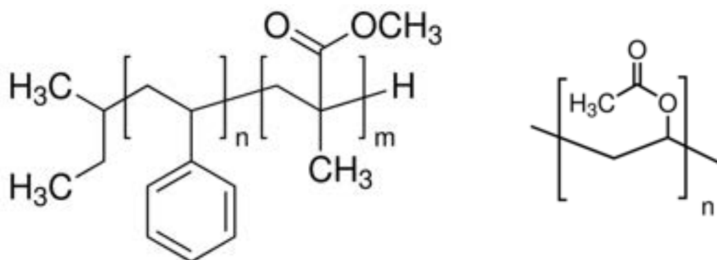
Figura 4. A sinistra formula di struttura del copolimero stirolo metil metacrilato (SMMA). A destra formula di struttura dell'omopolimero polivinilacetato (PVA).
