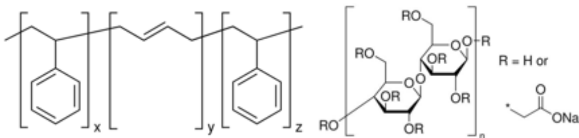
Figura 3. A sinistra formula di struttura del copolimero stirene-butadiene (SBR). A destra formula di struttura della metilcellulosa ( R = H ) o del sale sodico della carbossimetilcellulosa ( R = -CH_2COONa ).
