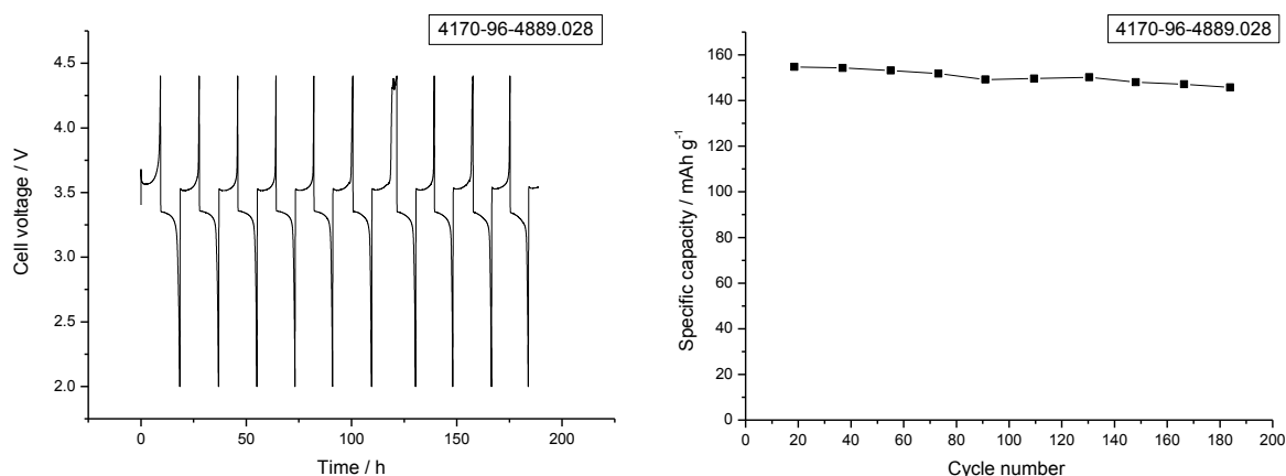
Figura 17. Profili di tensione in funzione del tempo (a sinistra) e capacità specifica in funzione del numero dei cicli (a destra) per un elettrodo a base di \text{LiFePO}_4 fatto ciclare in una cella al litio metallico a rate di carica/scarica pari a C/10.
