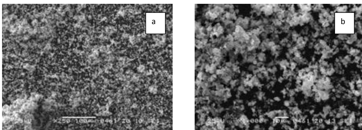
Figura 8. a) Micrografia a medio ingrandimento (X250) e b) ad alto ingrandimento (X1000) del \text{LiFePO}_4 .
