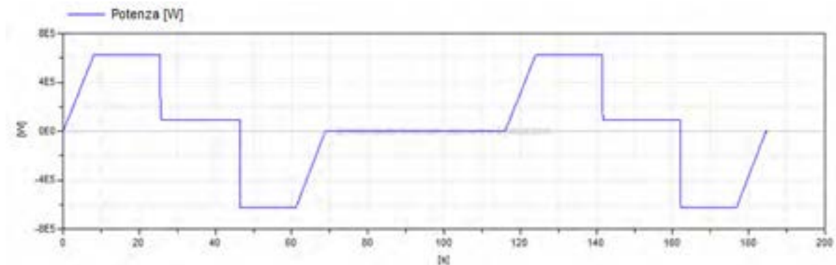
Figura 4. Andamento della potenza assorbita/erogata dal convoglio durante il ciclo
