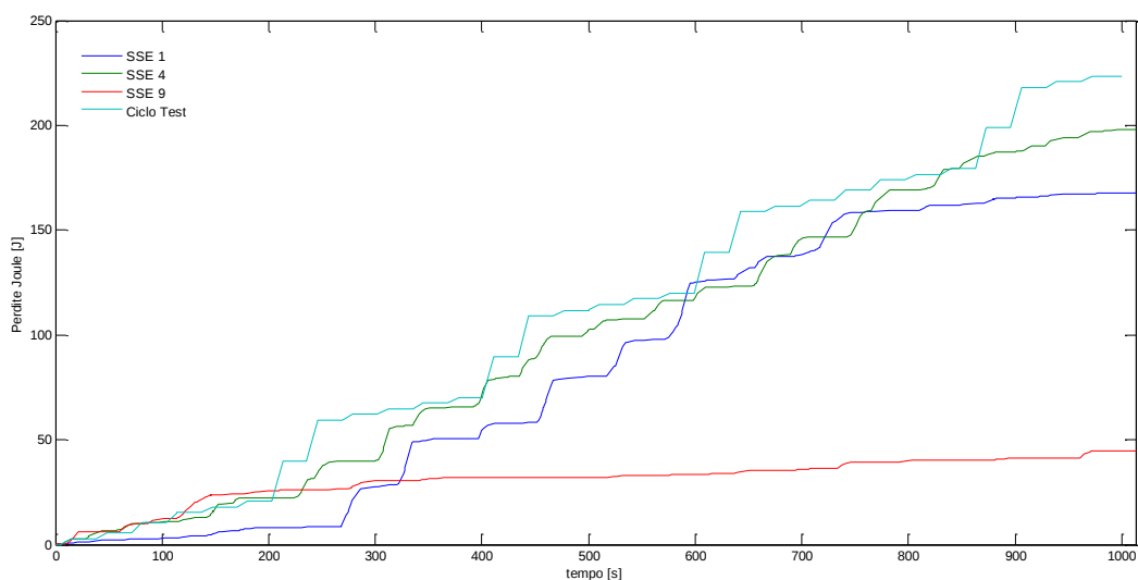
Figura 18. Energia dispersa per effetto Joule nei quattro cicli
