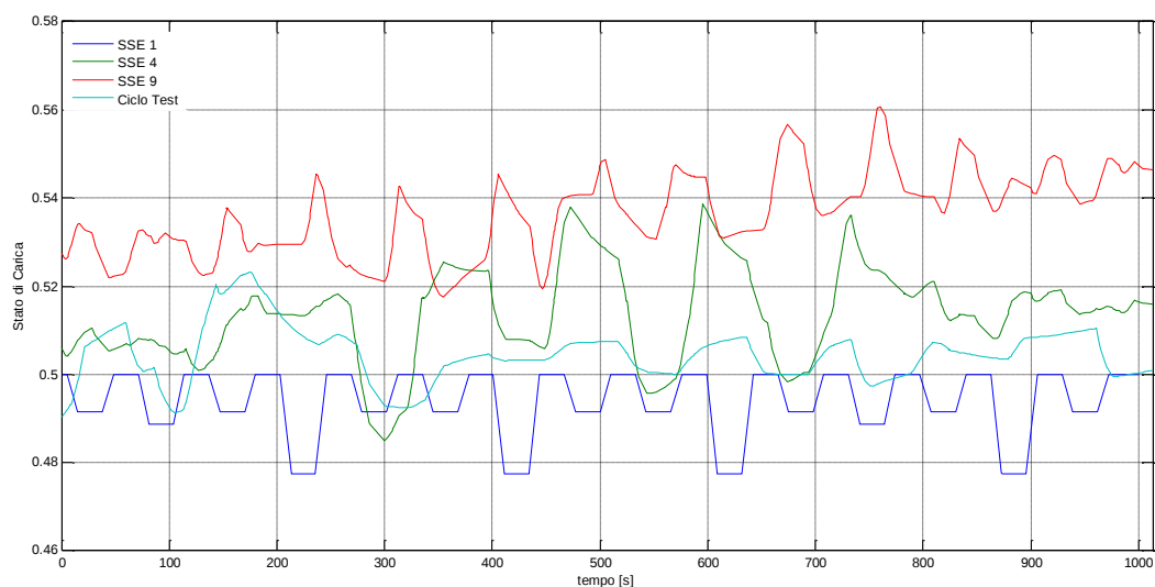
Figura 17. Variazioni di stato di carica
