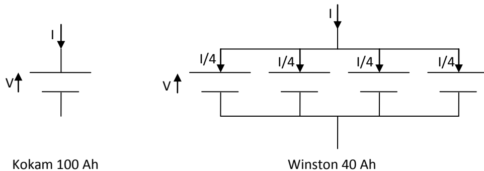
Figura 20. Costruzione del modulo batterie con celle da 100 Ah e con celle da 40 Ah
