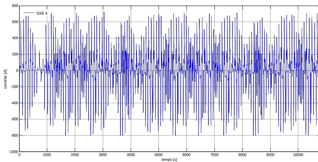
Figura 5. Corrente erogata/assorbita dall'accumulo della sottostazione quattro
