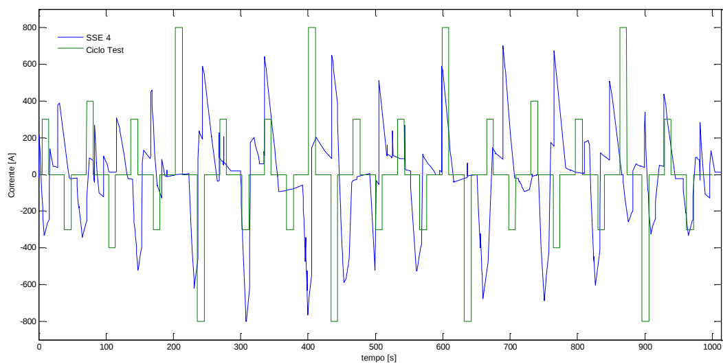
Figura 16. Confronto tra il ciclo test e l'andamento di corrente della SSE 4
