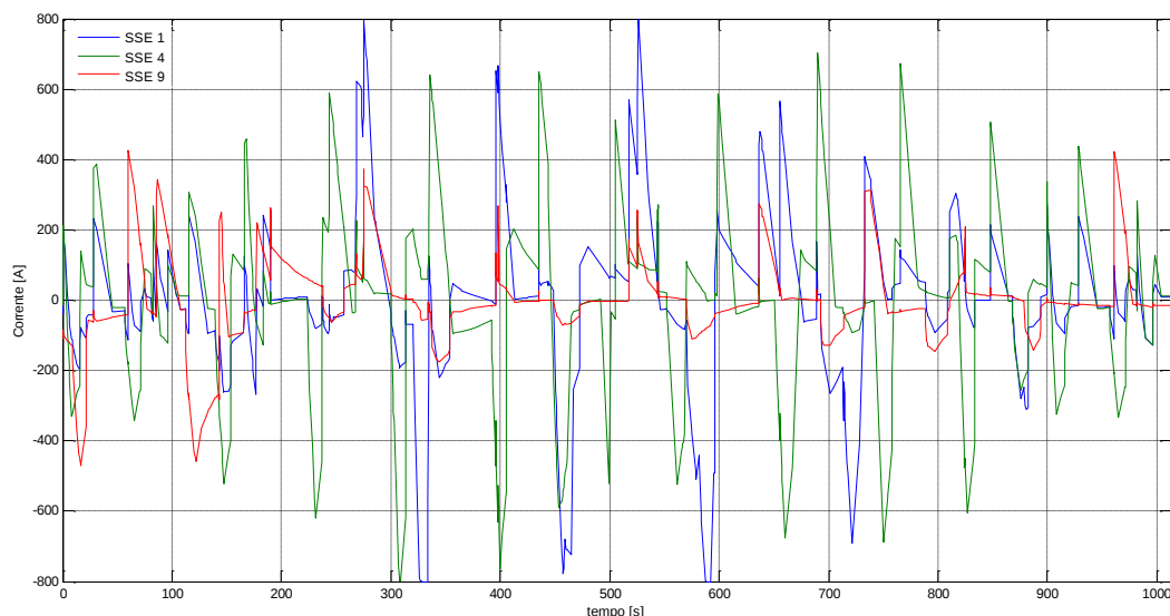
Figura 7. Correnti erogate dall'accumulo in un periodo di funzionamento
