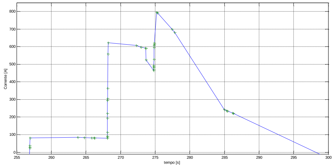
Figura 13. Picco della corrente erogata dalla SSE 1
