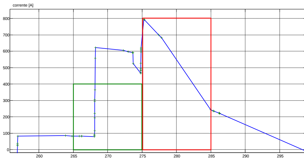
Figura 14. Gradini di corrente
