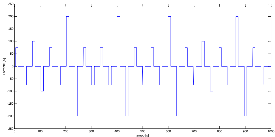
Figura 21. Ciclo Test per le batterie da 40 Ah
