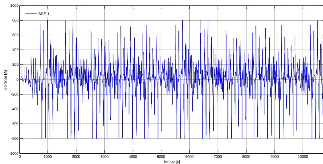
Figura 4. Corrente erogata/assorbita dall'accumulo della sottostazione uno
