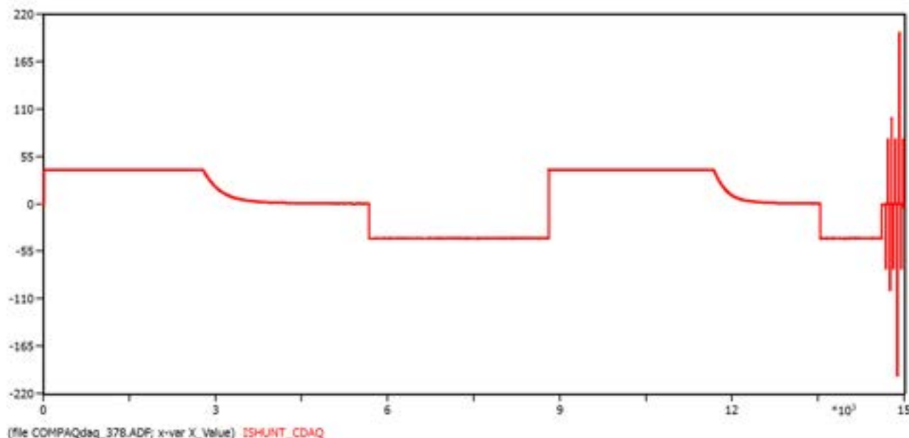
Figura 26. Ciclo di carica e scarica per la misura della capacità – andamento della corrente
