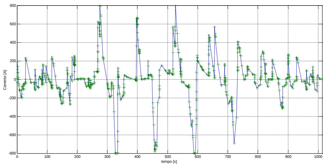
Figura 12. Corrente erogata dalla SSE 1
