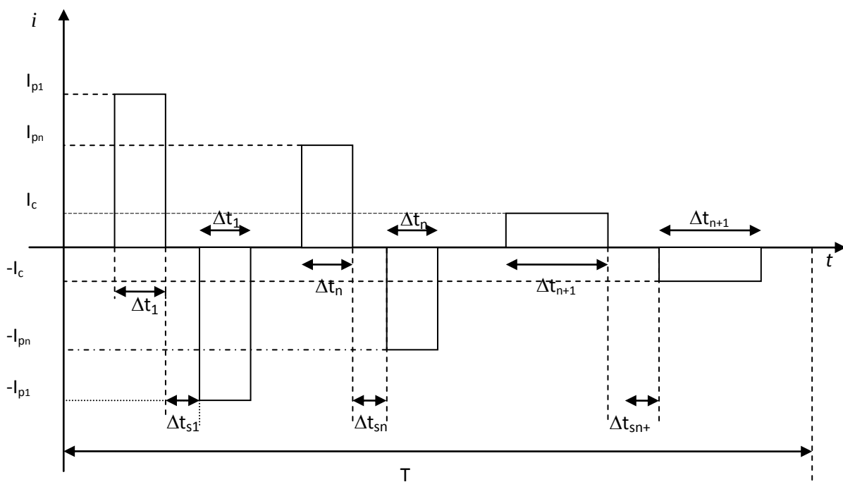
Figura 10. Struttura base del ciclo di riferimento
