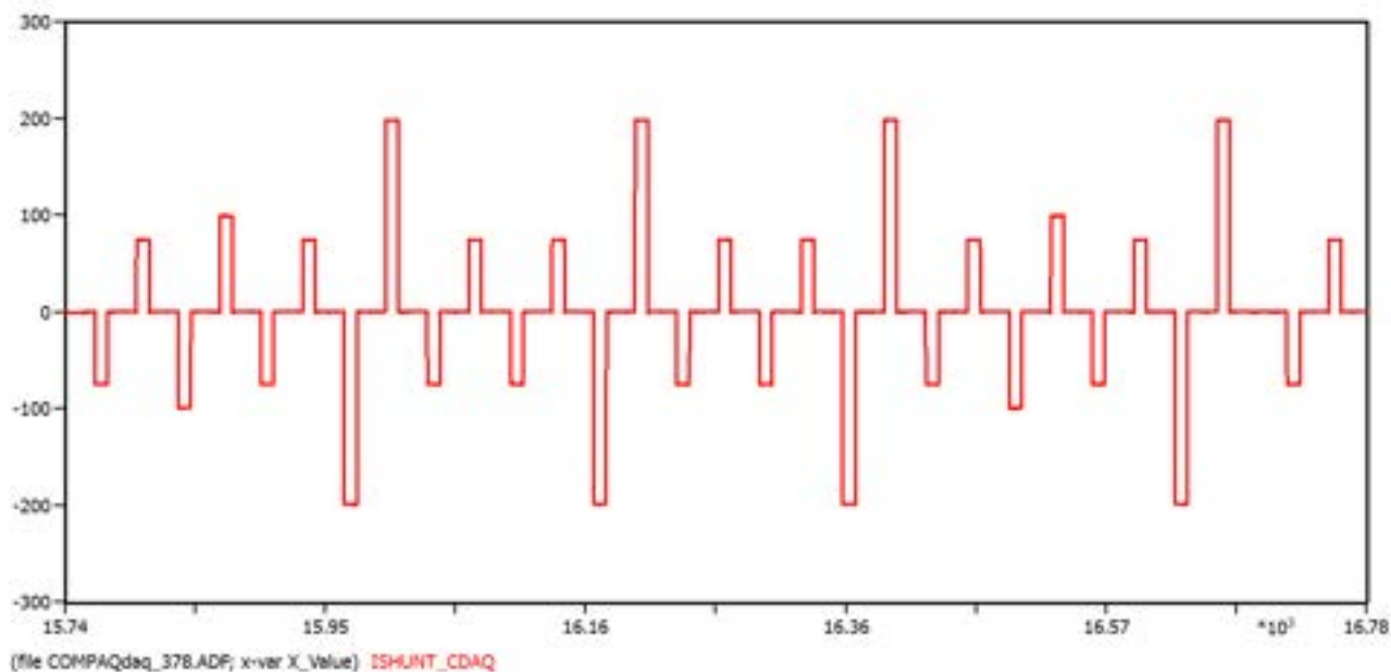
Figura 22. Particolare dell'andamento della corrente nella prova di laboratorio
