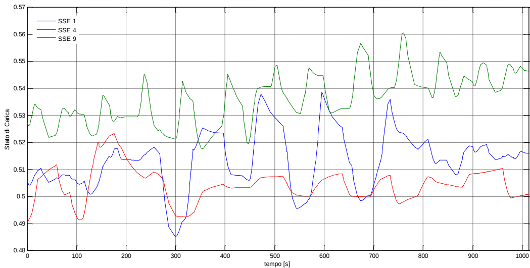
Figura 8. Andamento dello stato di carica
