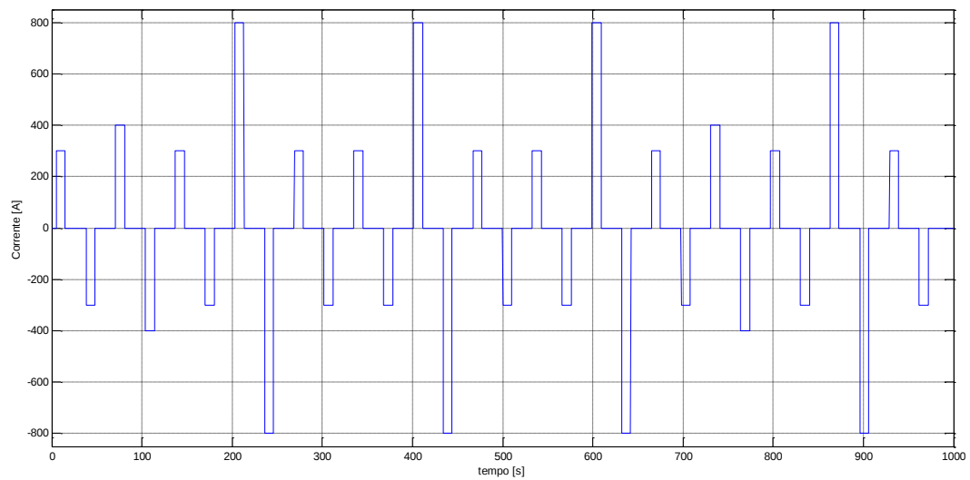
Figura 15. Ciclo di riferimento
