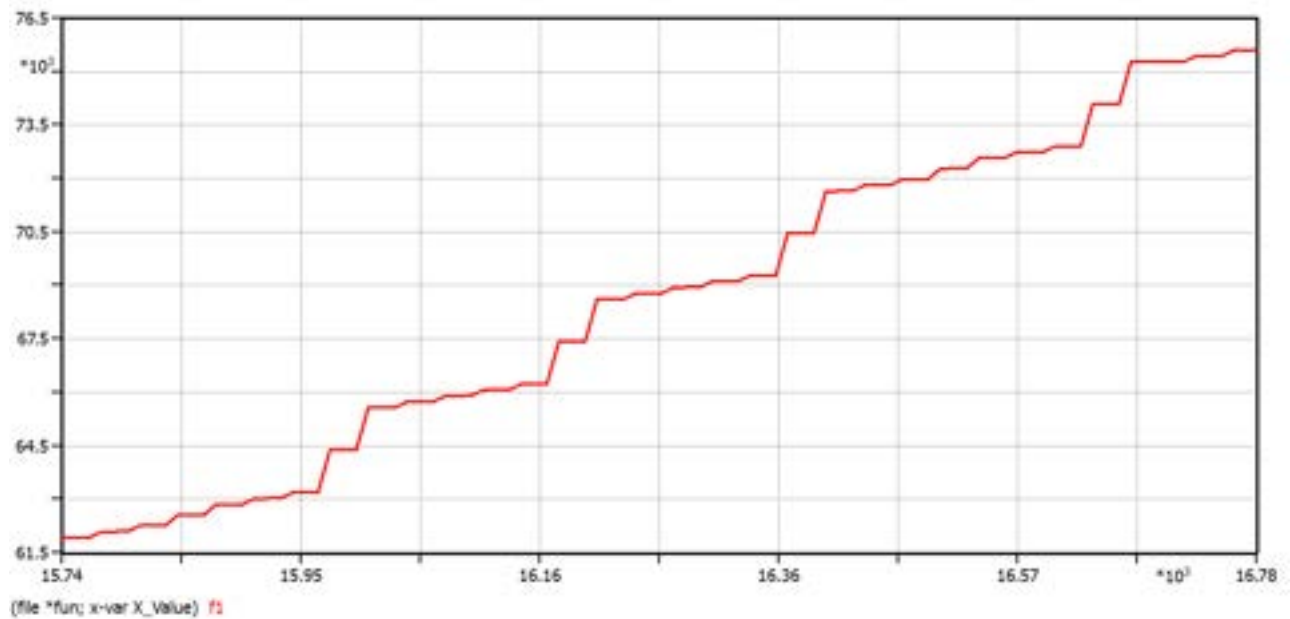
Figura 24. Energia dispersa per effetto Joule
