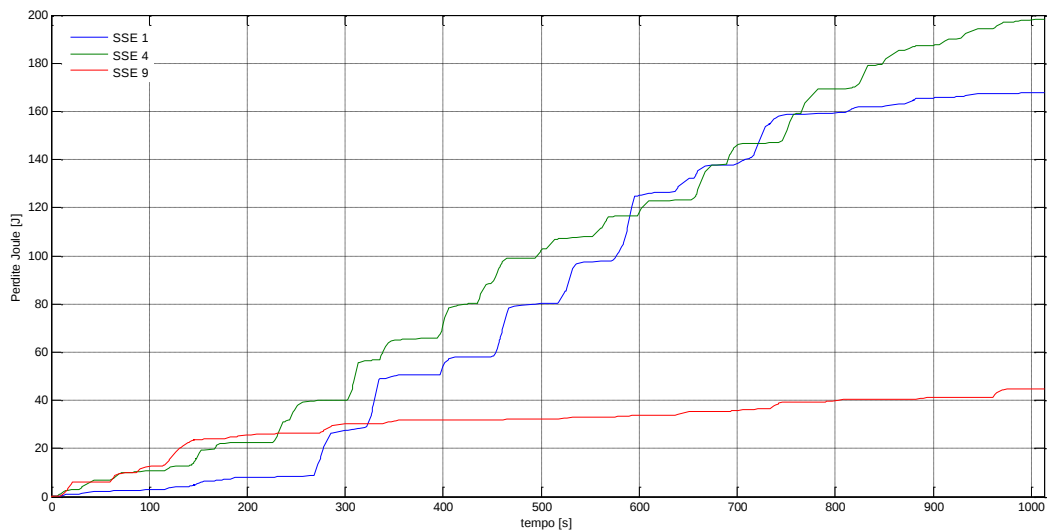
Figura 9. Perdite Joule
