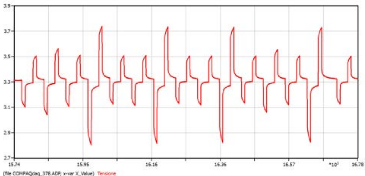
Figura 23. Particolare dell'andamento della tensione di cella
