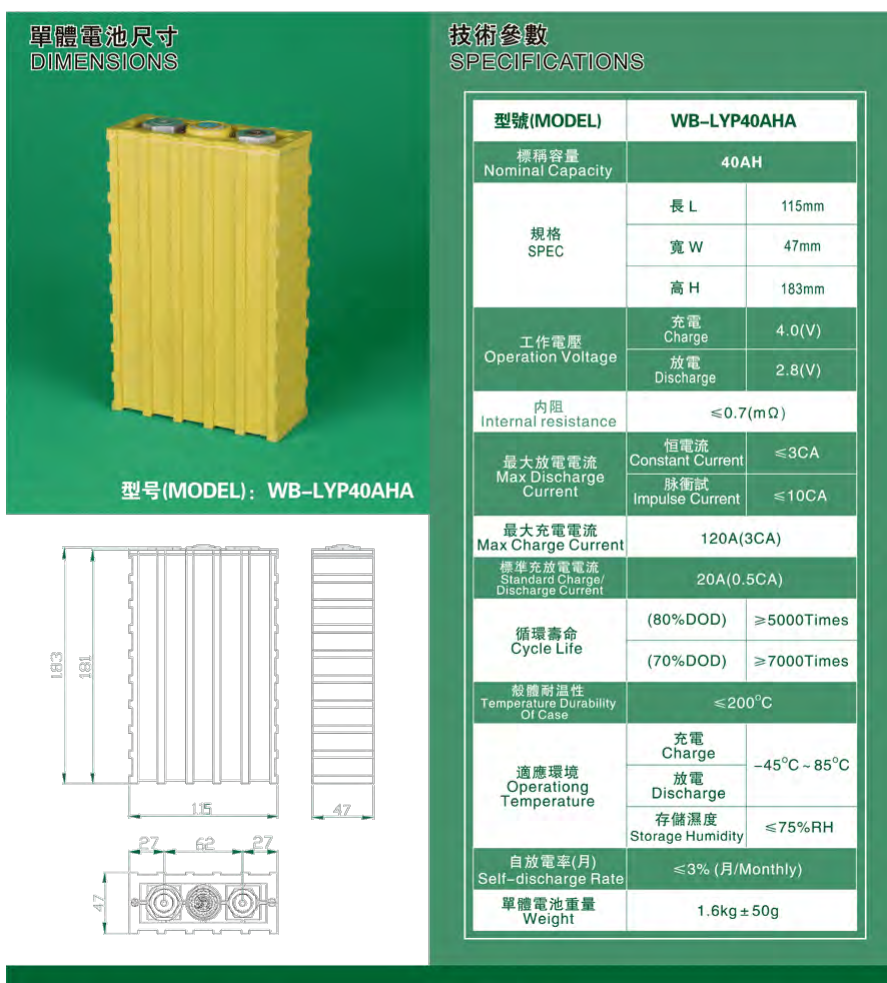
Figura 19. Caratteristiche delle batterie sottoposte a test
