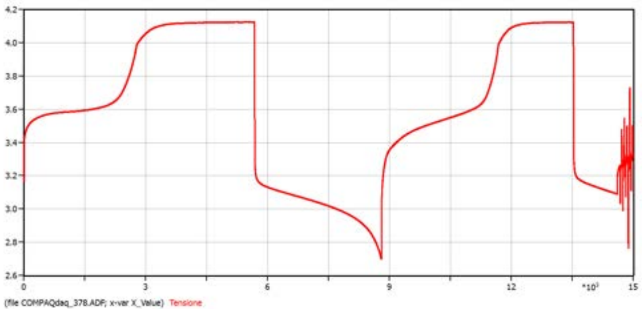
Figura 27. Andamento delle tensioni nel ciclo di carica e scarica standard
