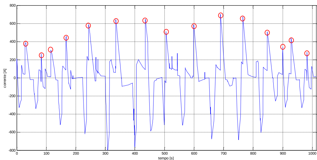
Figura 11. Picchi di corrente nella SSE 4
