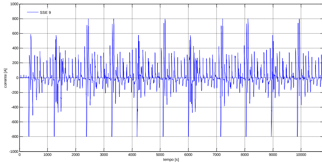
Figura 6. Corrente erogata/assorbita dall'accumulo della sottostazione nove
