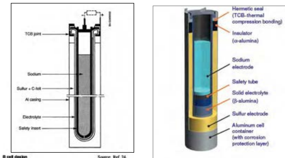
Figura 5. Cella ABB con tecnologia Na/S
