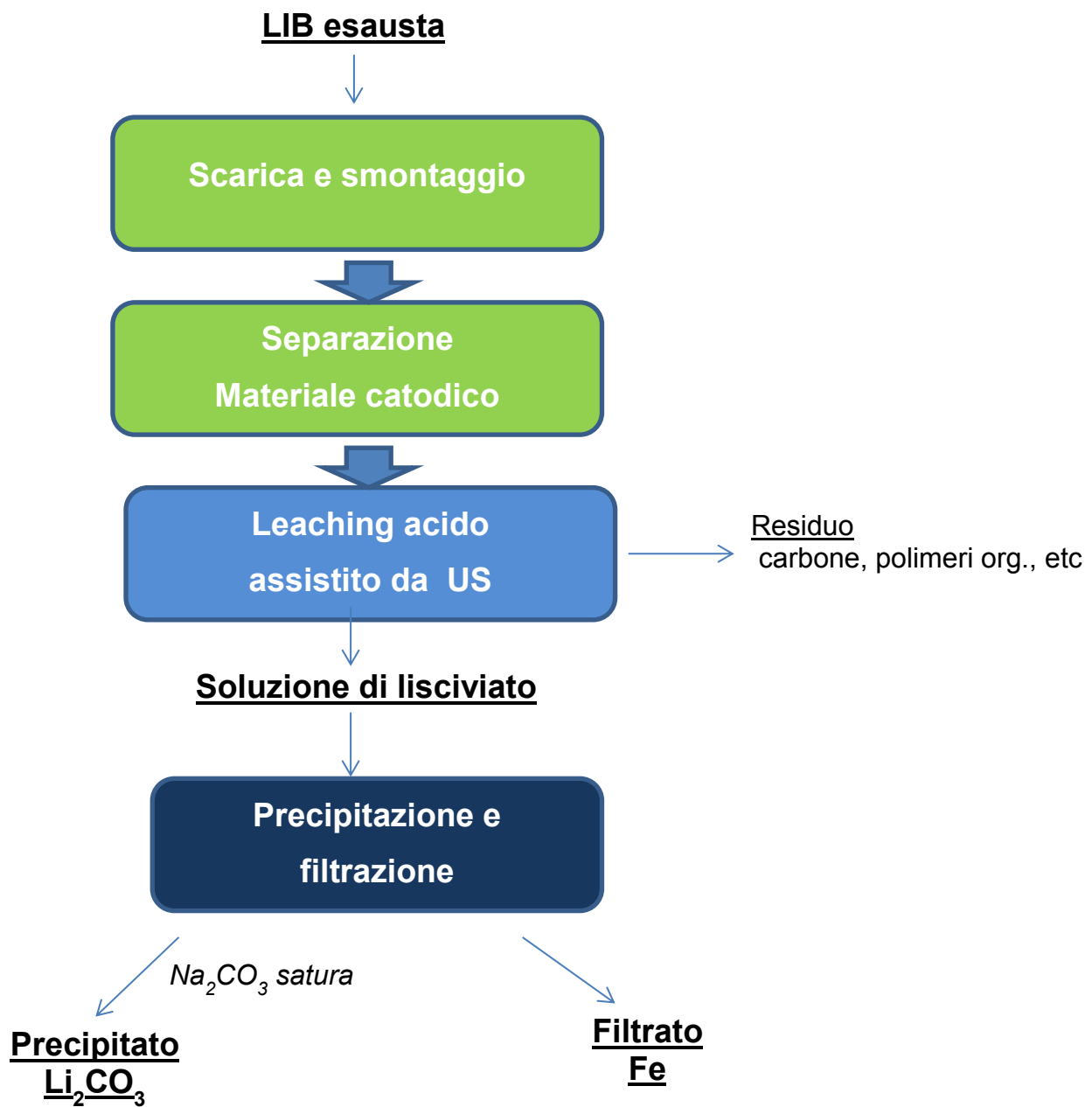
Figura 4. Schema del processo di trattamento proposto
