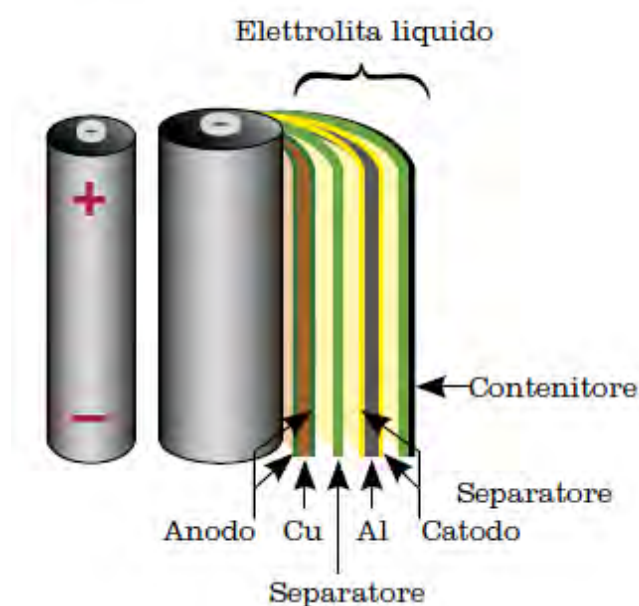
Figura 1. Struttura schematica di una batteria al litio
