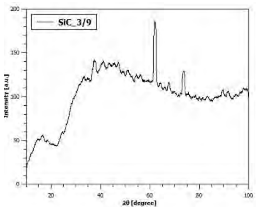
Figura 31. Diffrattogramma ottenuto su filtro in SiC + 25% catalizzatore
