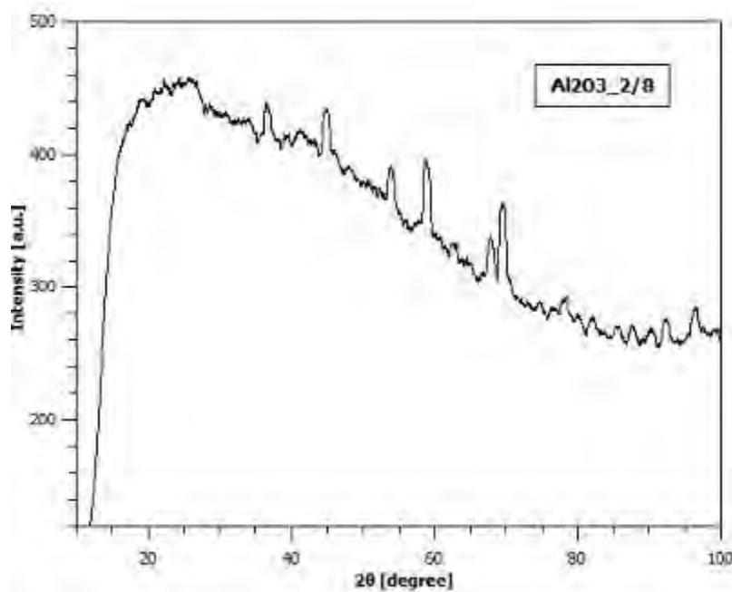
Figura 33. Diffratogramma ottenuto su filtro in Al_2O_3 non catalizzato
