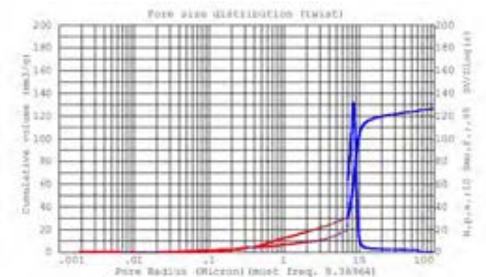
Figura 27. Porogramma relativo a SiC + 15% catalizzatore
