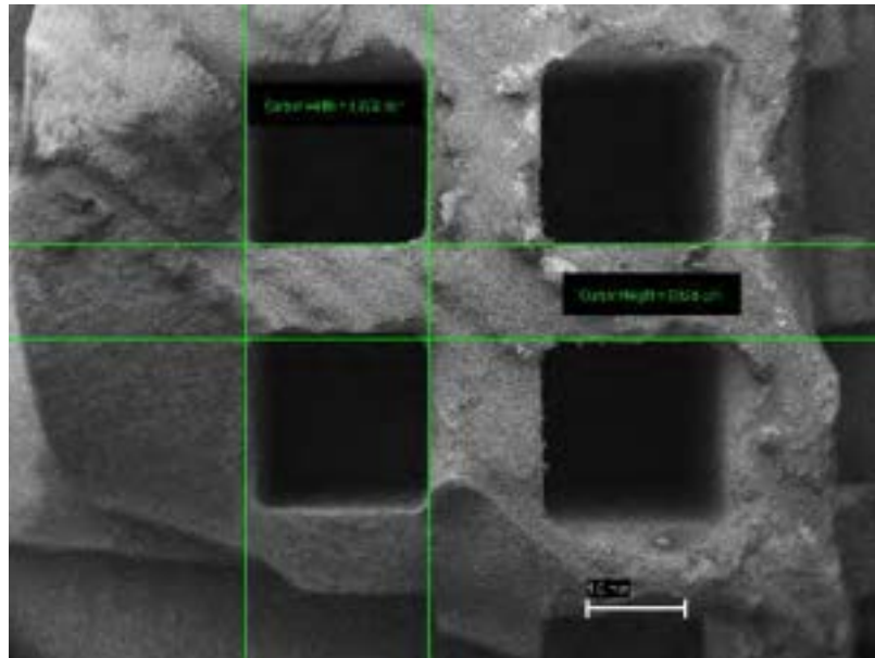
Figura 17. Analisi al SEM della sezione del filtro \text{Al}_2\text{O}_3 92% a basso ingrandimento
