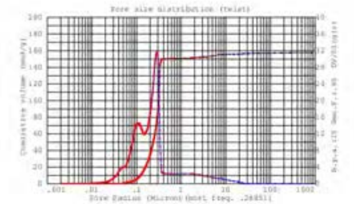
Figura 28. Porogramma relativo ad Al 2 O 3 92%
