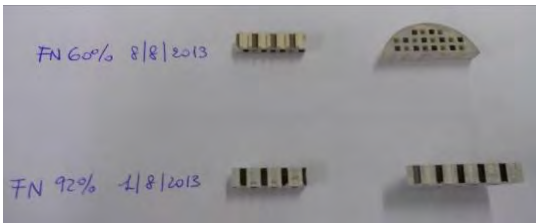
Figura 34. Immagini di campioni in Al 2 O 3 prima della metallizzazione
