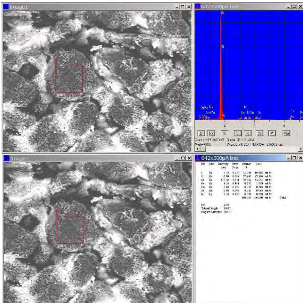
Figura E4 – Analisi EDS
