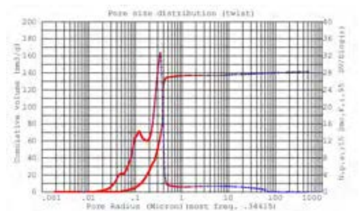
Figura 29. Porogramma relativo ad Al 2 O 3 60%
