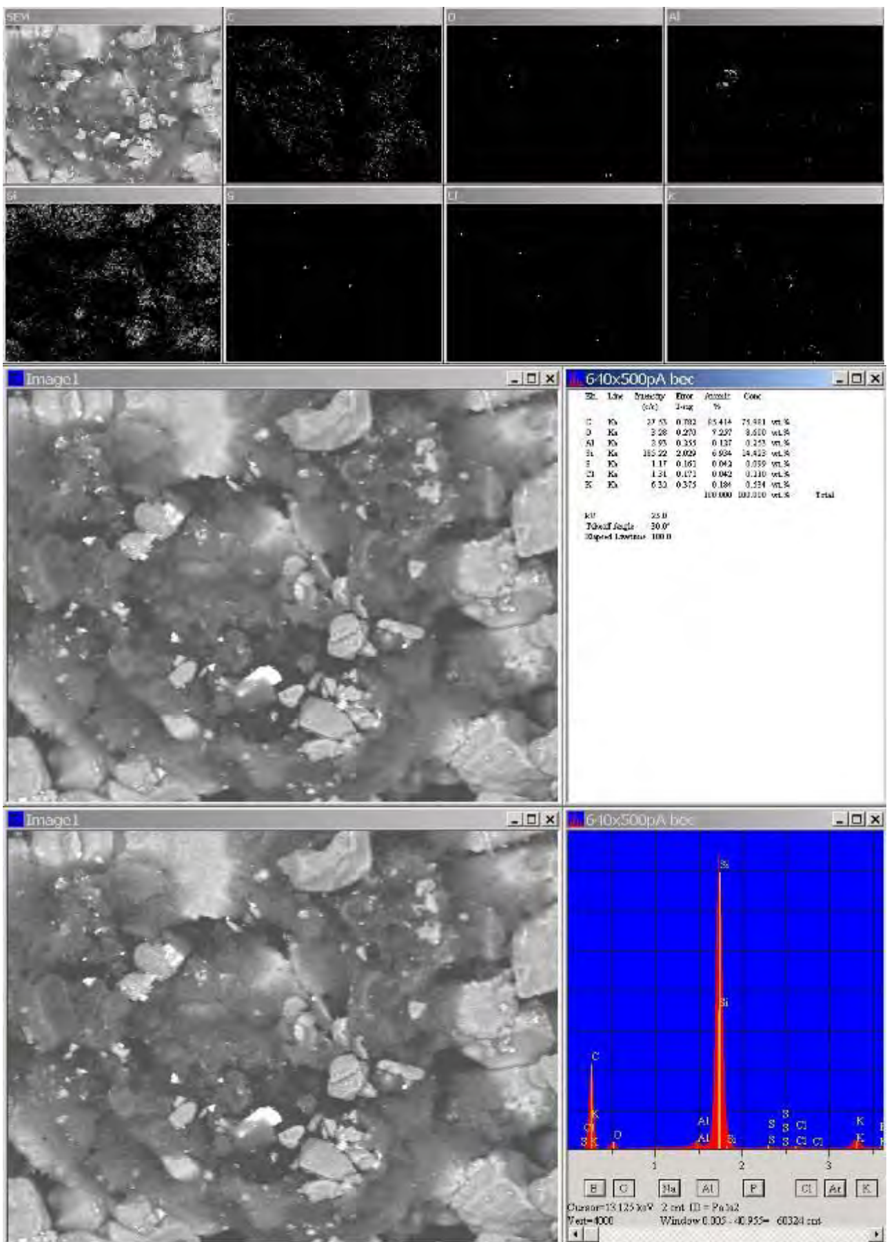
Figura C2 – Analisi EDS
