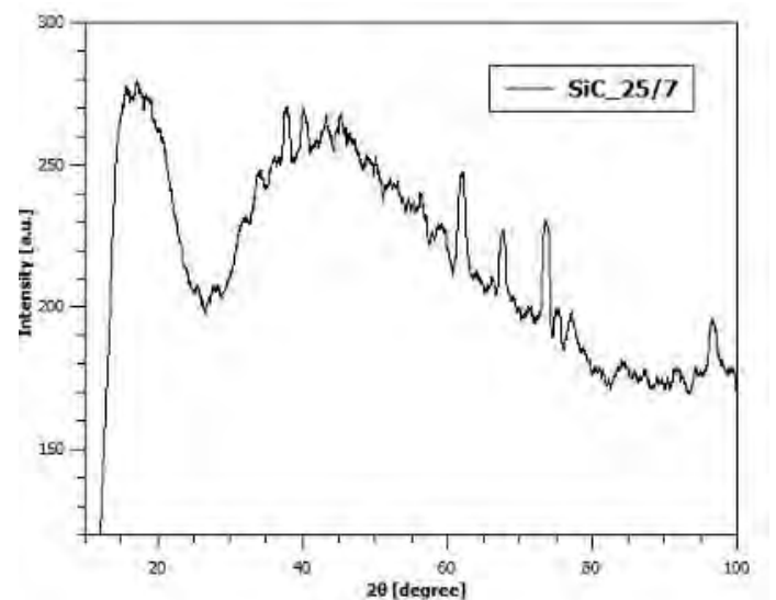
Figura 30. Diffrattogramma ottenuto su filtro in SiC non catalizzato
