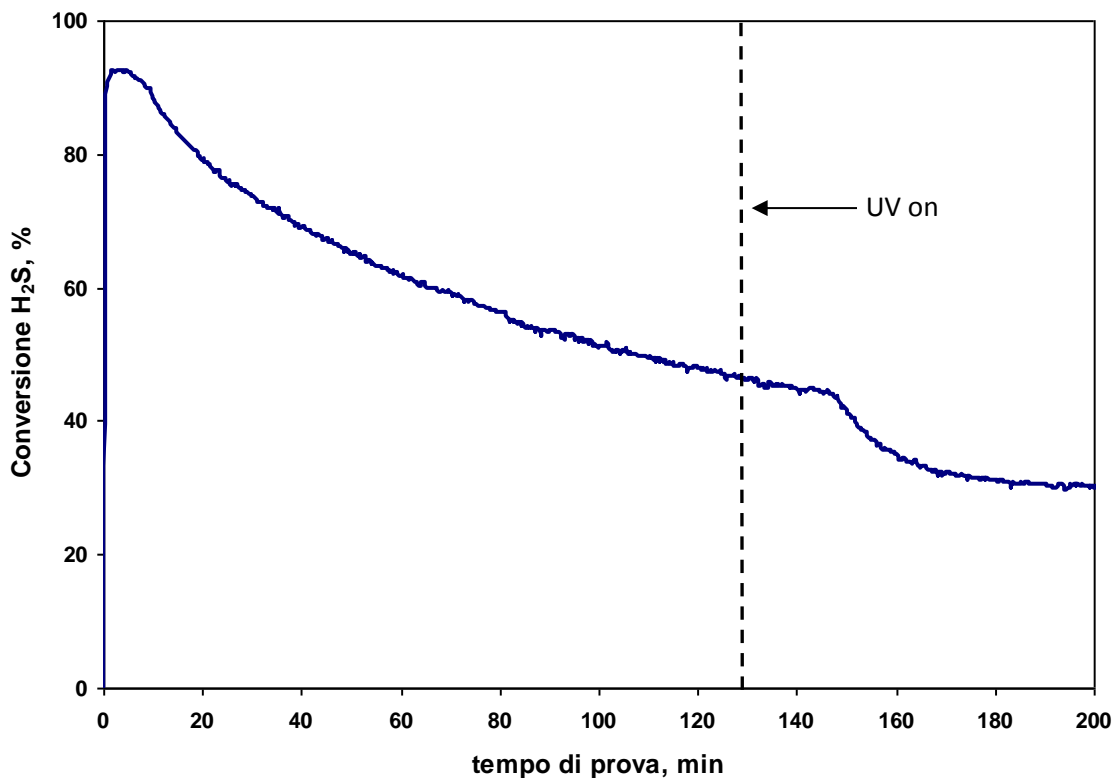
Figura 2. Andamento della conversione di H_2S in funzione del tempo di prova; portata totale: 39\text{ NL/h} ; temperatura di reazione: 50\text{ }^\circ\text{C}
